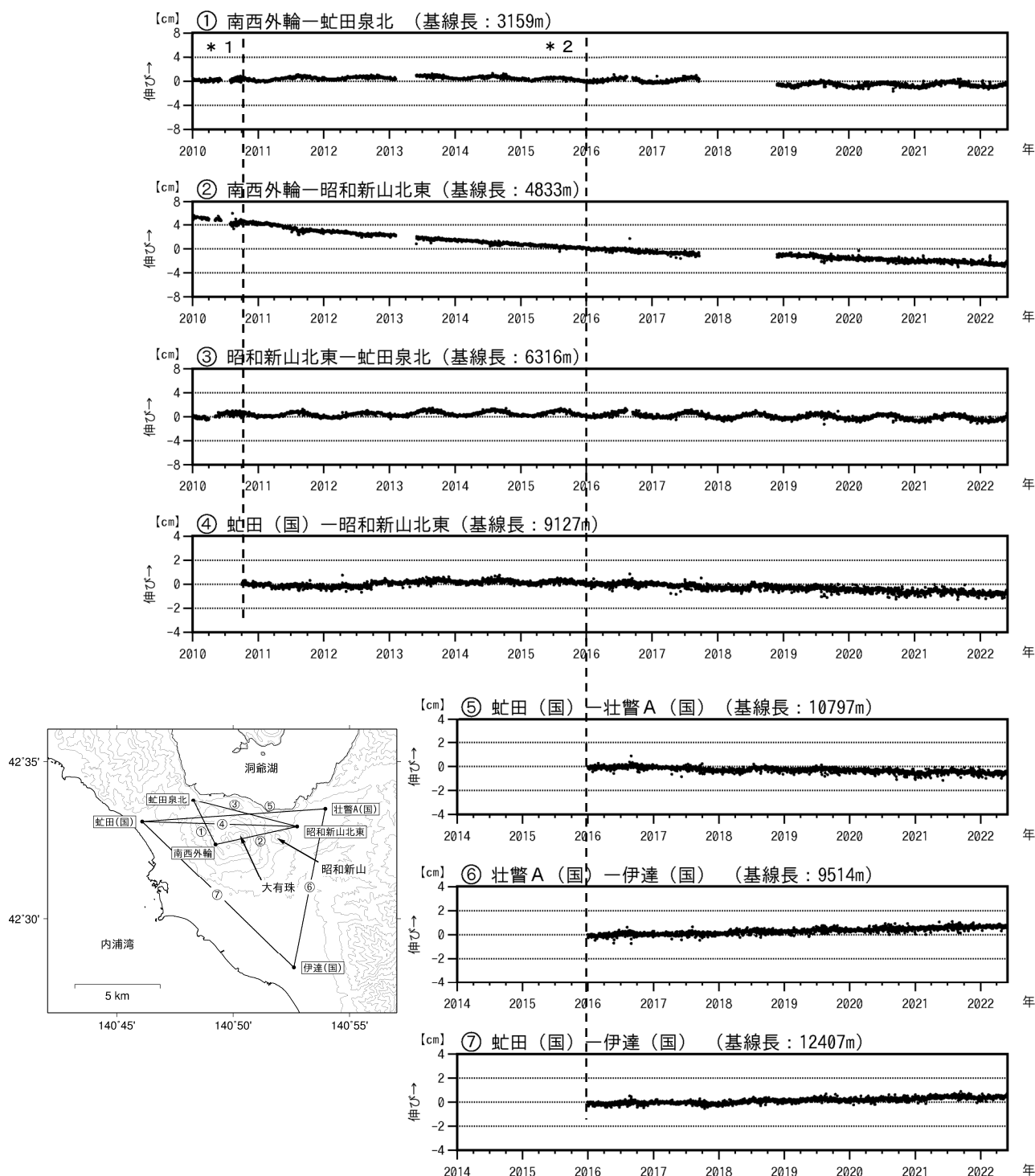
図6 有珠山 GNSS連続観測による基線長変化（2010年1月～2022年5月）及び観測点配置図
