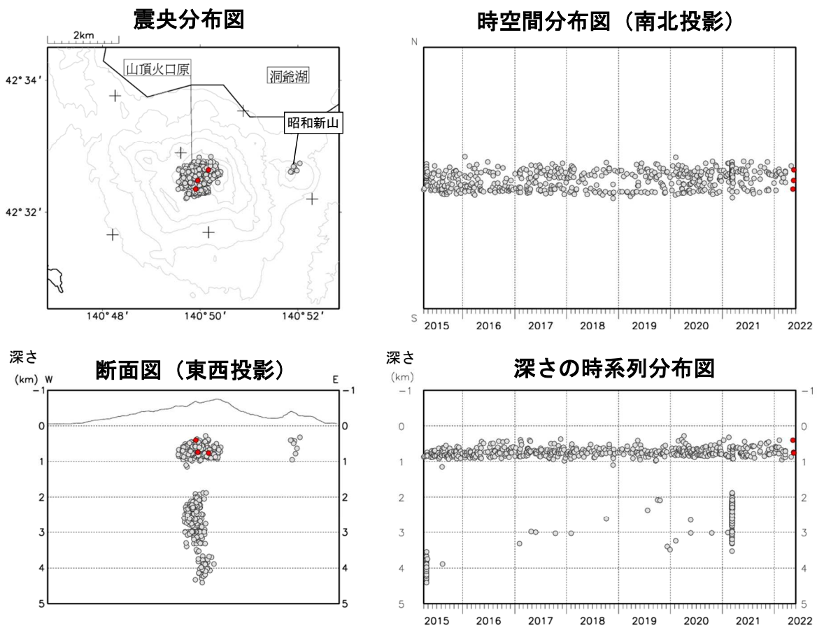
図5 有珠山 火山性地震の震源分布（2015年4月～2022年5月）
