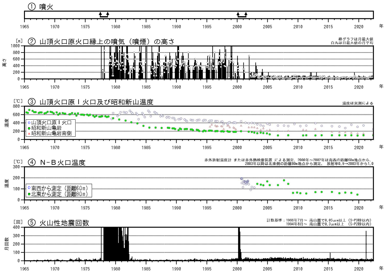
図1 有珠山 火山活動経過図（1965年1月～2022年5月）
