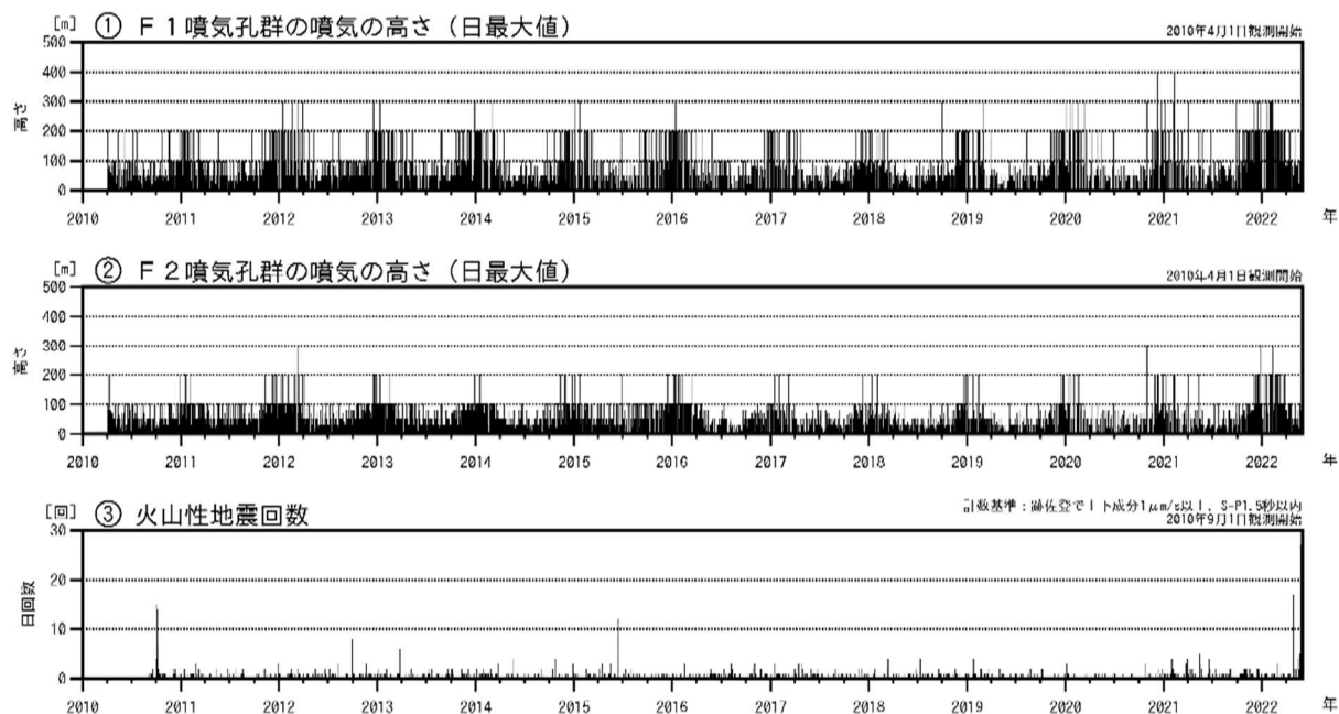
図1 アトサヌプリ 火山活動経過図（2010年4月～2022年5月）
