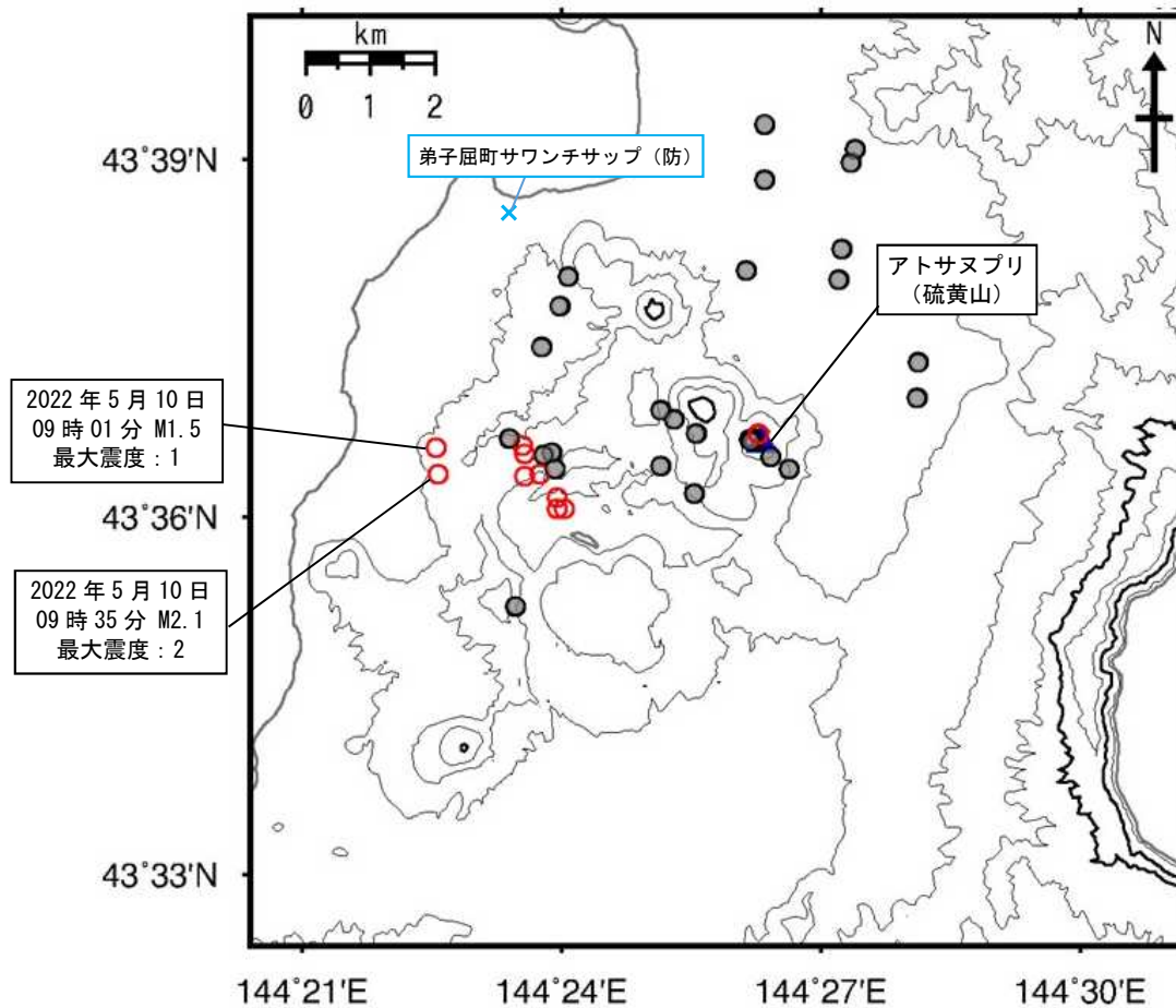
図3 アトサヌプリ 火山性地震の震央分布 (2019年10月～2022年5月)
