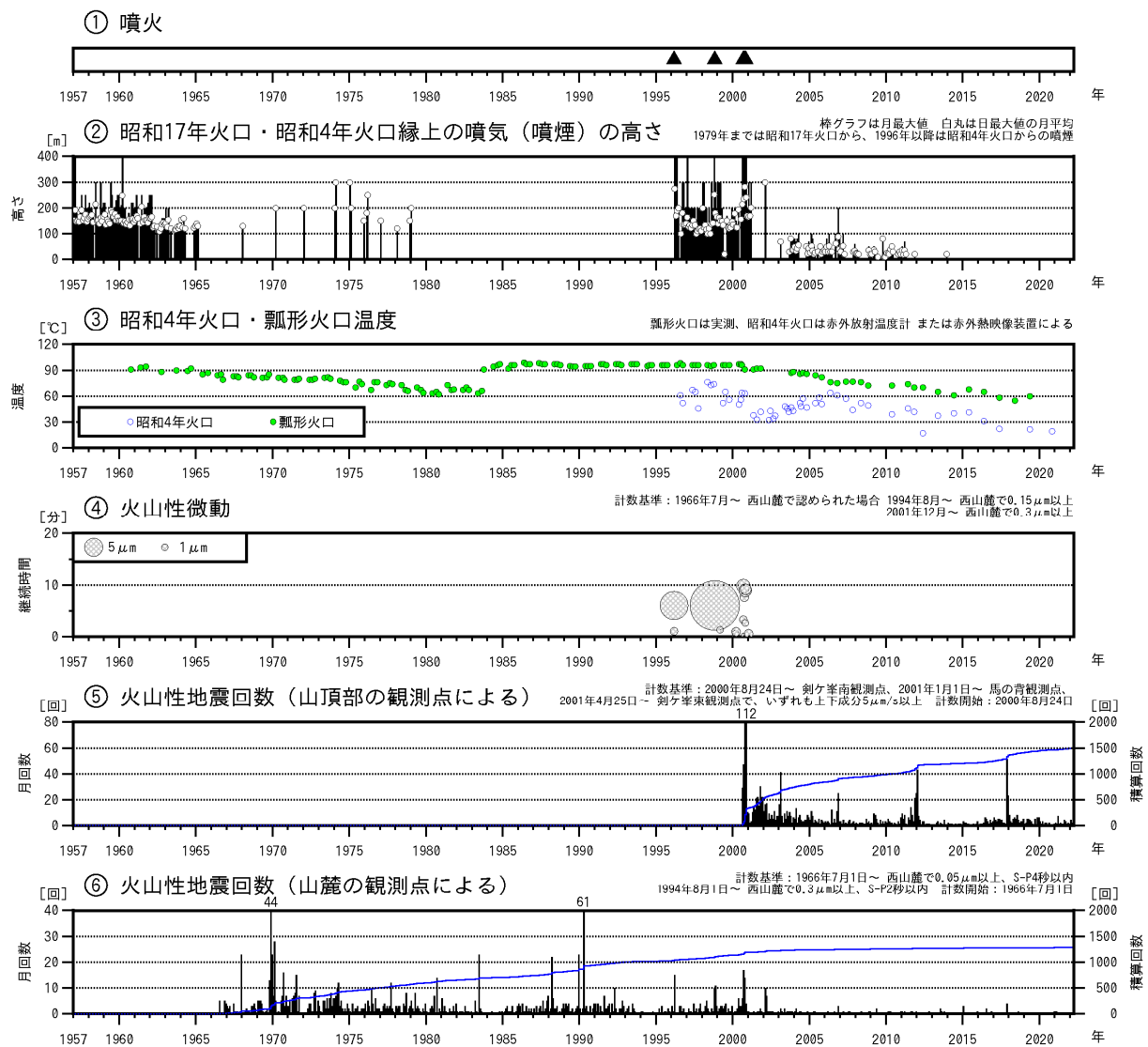
図1 北海道駒ヶ岳 火山活動経過図（1957年1月～2022年3月）
