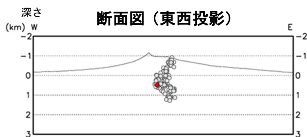
図4 北海道駒ヶ岳 火山性地震の震源分布（2002年12月～2022年3月）
