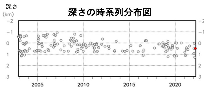
図4 北海道駒ヶ岳 火山性地震の震源分布（2002年12月～2022年3月）
