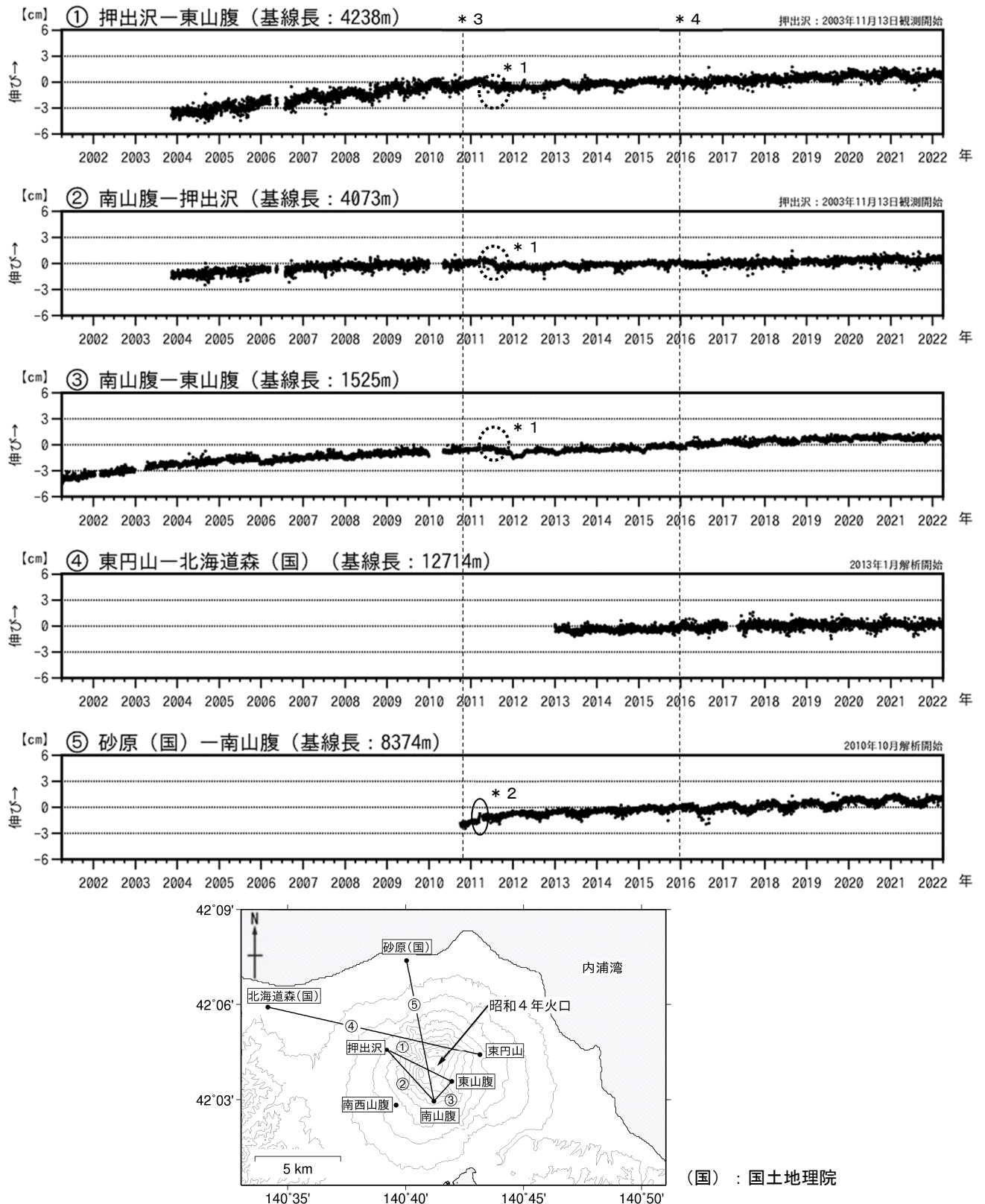
図5 北海道駒ヶ岳 GNSS連続観測による基線長変化（2001年4月～2022年3月）及び観測点配置図 グラフ①～⑤は観測点配置図の基線①～⑤に対応しています。 グラフの空白部分は欠測を示します。 ①～③の点線円内の変動（* 1）は、2011年8月の機器更新によるものです。 ⑤の楕円内の変動（* 2）は、2011年3月11日に発生した「平成23年（2011年）東北地方太平洋沖地震」の影響によるものです。 2010年10月（* 3）及び2016年1月（* 4）に解析方法を変更しています。
