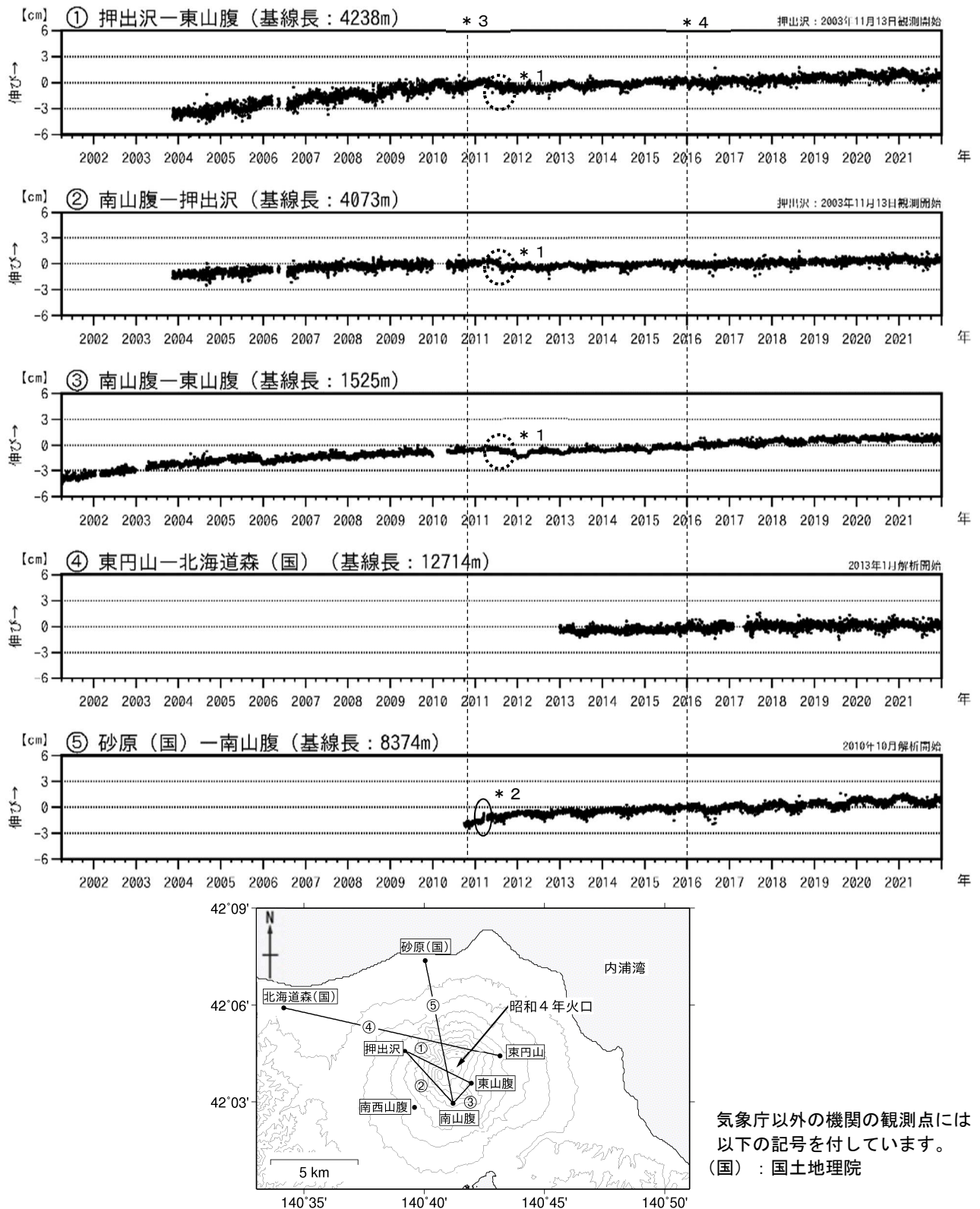
図5 北海道駒ヶ岳 GNSS連続観測による基線長変化（2001年4月～2021年12月）及び観測点配置図
