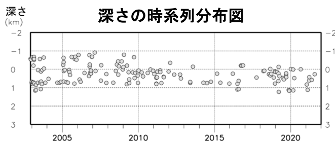
図4 北海道駒ヶ岳 火山性地震の震源分布（2002年12月～2021年12月）
