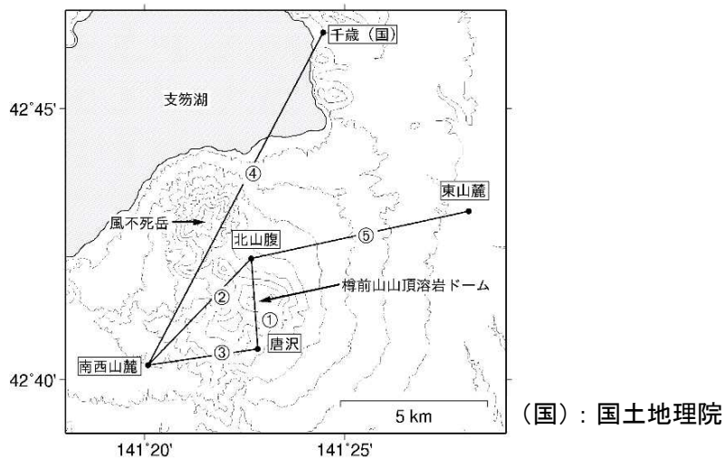
図8 樽前山 GNSS連続観測による基線長変化（2005年1月～2021年9月）及び観測点配置図
