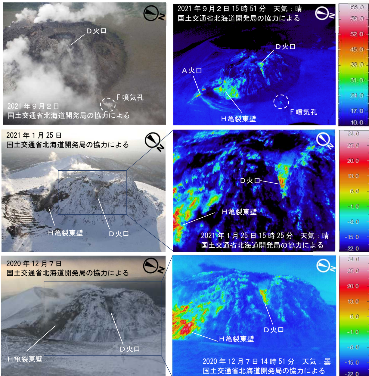
図5 樽前山 赤外熱映像装置による山頂溶岩ドーム東側の地表面温度分布
