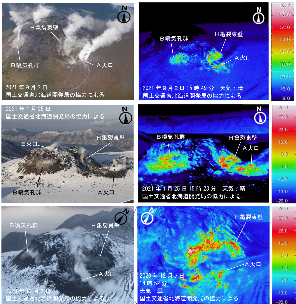
図6 樽前山 赤外熱映像装置による山頂溶岩ドーム南側～南東側の地表面温度分布
