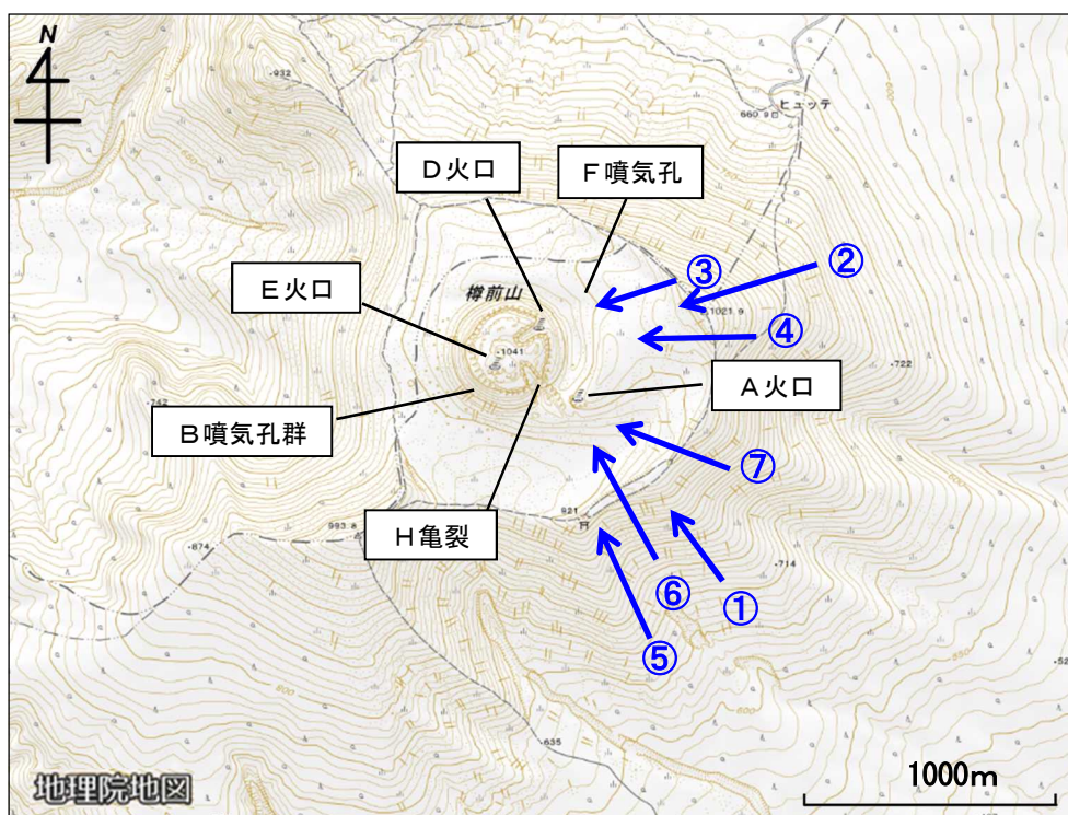
図4 樽前山 山頂溶岩ドーム周辺図と赤外熱映像及び写真の撮影方向（矢印）
