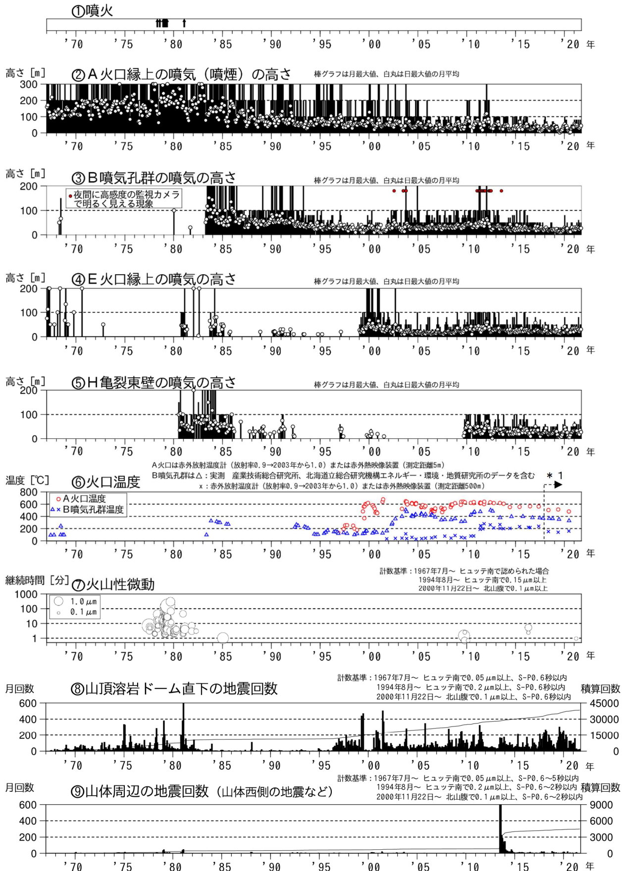
図2 樽前山 火山活動経過図(1967年1月~2021年9月)
