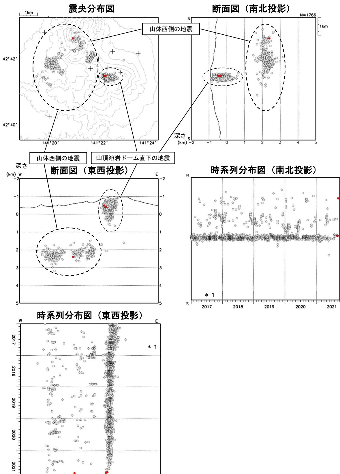
図7 樽前山 火山性地震の震源分布（2017年1月～2021年9月） ○印：2017年1月～2021年8月の震源、●印：2021年9月の震源、+印：地震観測点 2017年10月31日（*1）以降、震源計算に利用する観測点を変更しています。
