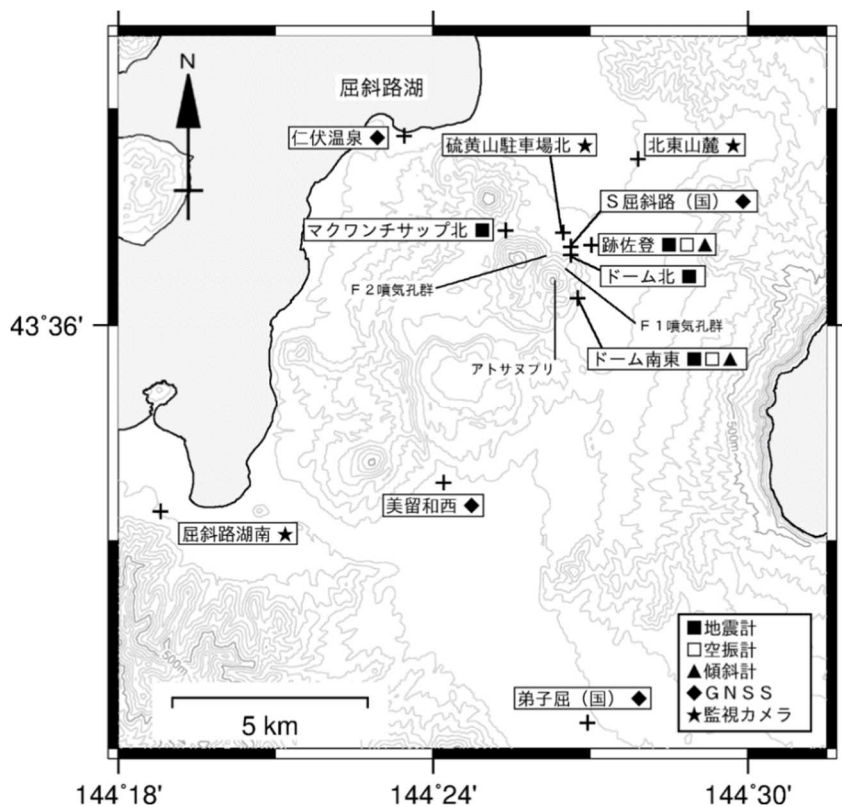
図10 アトサヌプリ 観測点配置図
