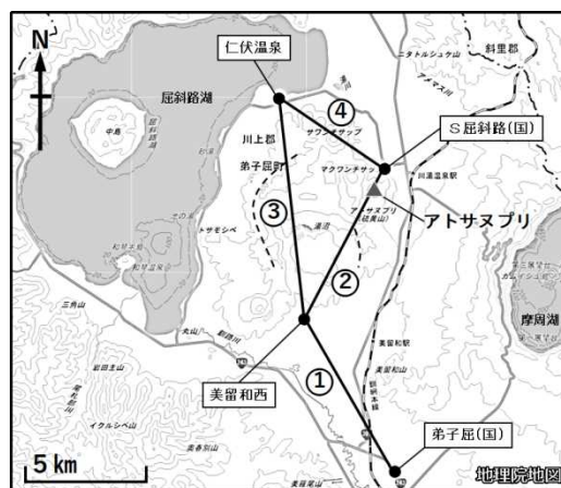
図5 アトサヌプリ GNSS連続観測による基線長変化（2010年10月～2021年7月）及び観測点配置図 ①～②の破線円内の変動（*1）は、美留和西観測点の局所的な動きによるもので、火山活動によるものではないと考えられます。 ①の破線円内の変動（*2）は、弟子屈(国)付近の樹木の影響及び伐採（2012年9月下旬）によるものです。 グラフの空白部分は欠測を示します。 *3 勝井義雄（1958）阿寒・屈斜路火山群、地球科学、39巻。
