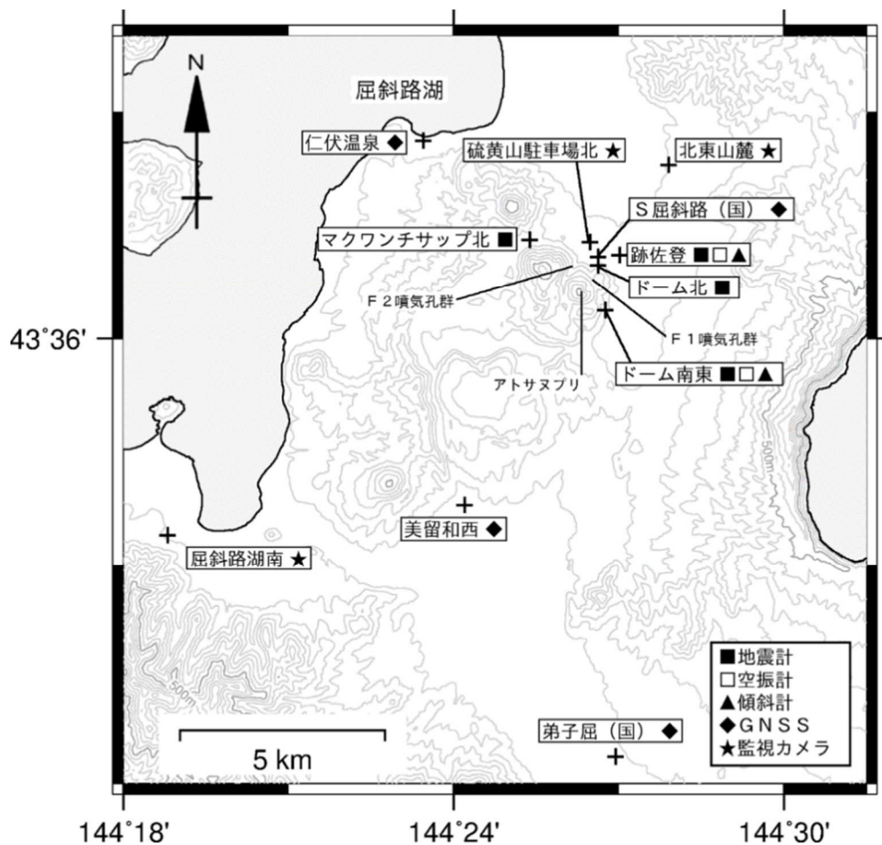
図6 アトサヌプリ 観測点配置図
