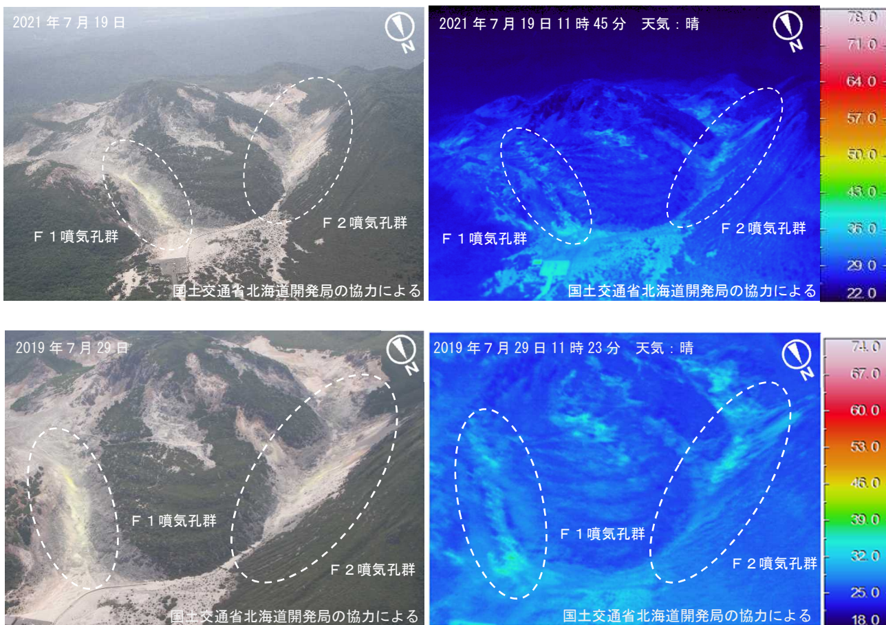
図4 アトサヌプリ 赤外熱映像観測装置によるF1噴気孔群及びF2噴気孔群の地表面温度分布（図3の①から撮影）
