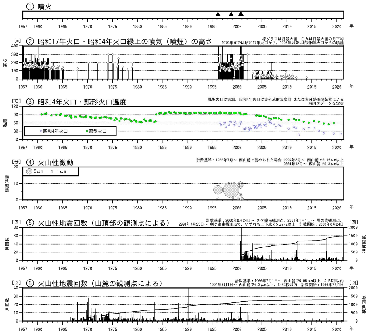
図1 北海道駒ヶ岳 火山活動経過図（1957年1月～2021年5月）
