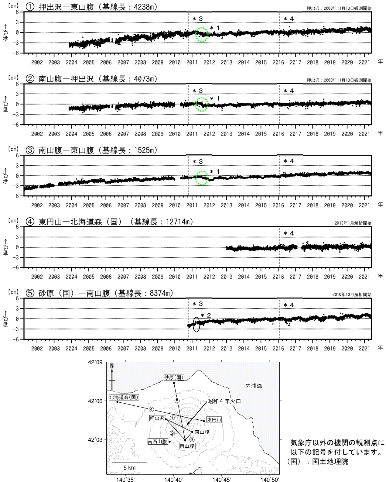
図5 北海道駒ヶ岳 GNSS連続観測による基線長変化（2001年4月～2021年5月）及び観測点配置図 グラフ①～⑤は観測点配置図の基線①～⑤に対応しています。 グラフの空白部分は欠測を示します。 ①～③の緑点線円内の変動（＊1）は、2011年8月の機器更新によるものです。 ⑤の黒楕円内の変動（＊2）は、2011年3月11日に発生した「平成23年（2011年）東北地方太平洋沖地震」の影響によるものです。 2010年10月（＊3）及び2016年1月（＊4）に解析方法を変更しています。
