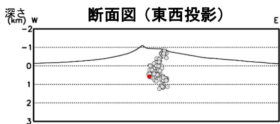
図4 北海道駒ヶ岳 火山性地震の震源分布（2002年12月～2021年5月）
