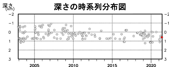
図4 北海道駒ヶ岳 火山性地震の震源分布（2002年12月～2021年5月）
