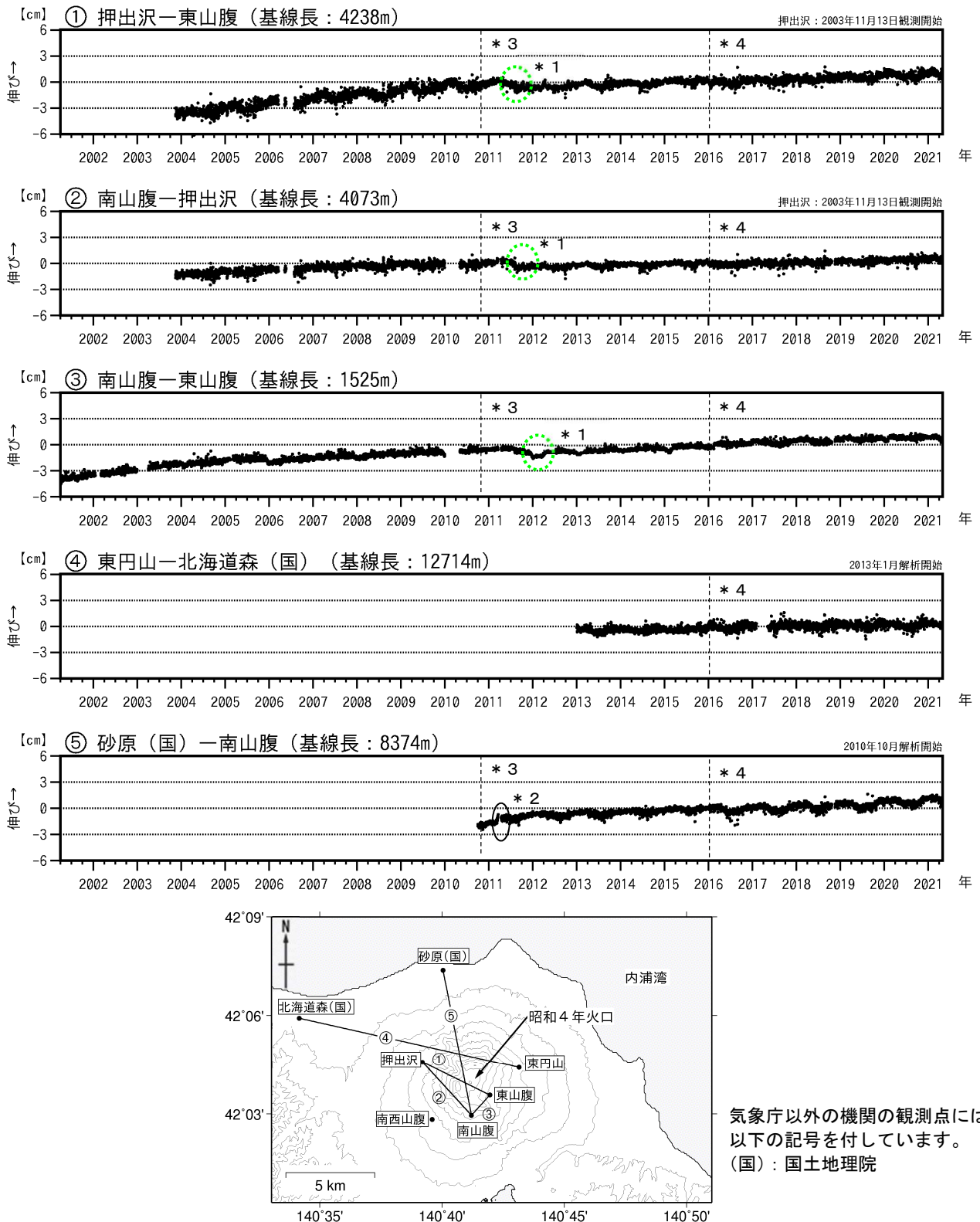
図5 北海道駒ヶ岳 GNSS連続観測による基線長変化（2001年4月～2021年4月）及び観測点配置図 GNSS基線①～⑤は観測点配置図の①～⑤に対応しています。 GNSS基線の空白部分は欠測を示します。 ①～③の緑点線円内の変動（*1）は、機器更新によるものです。 ⑤の黒楕円内の変動（*2）は、2011年3月11日に発生した「平成23年（2011年）東北地方太平洋沖地震」の影響によるものです。 2010年10月（*3）及び2016年1月（*4）に解析方法を変更しています
