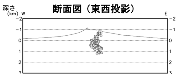
図4 北海道駒ヶ岳 火山性地震の震源分布（2002年12月～2021年4月）
