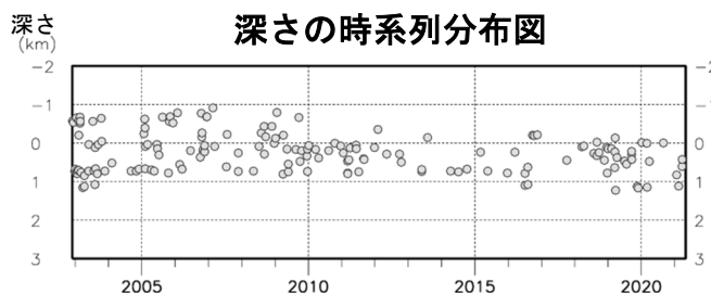
図4 北海道駒ヶ岳 火山性地震の震源分布（2002年12月～2021年4月）
