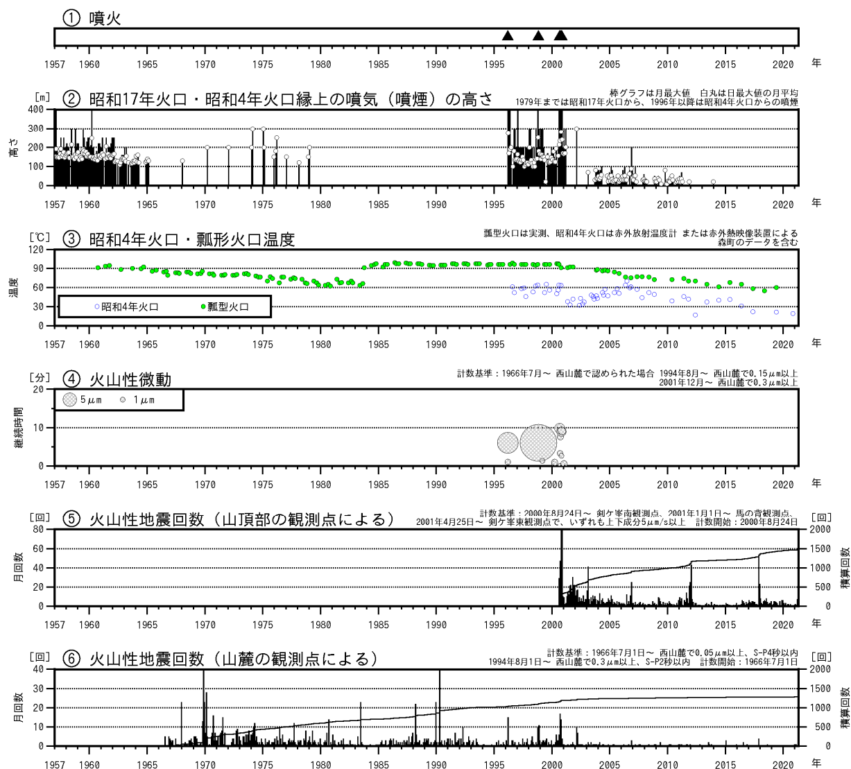
図1 北海道駒ヶ岳 火山活動経過図（1957年1月～2021年4月）
