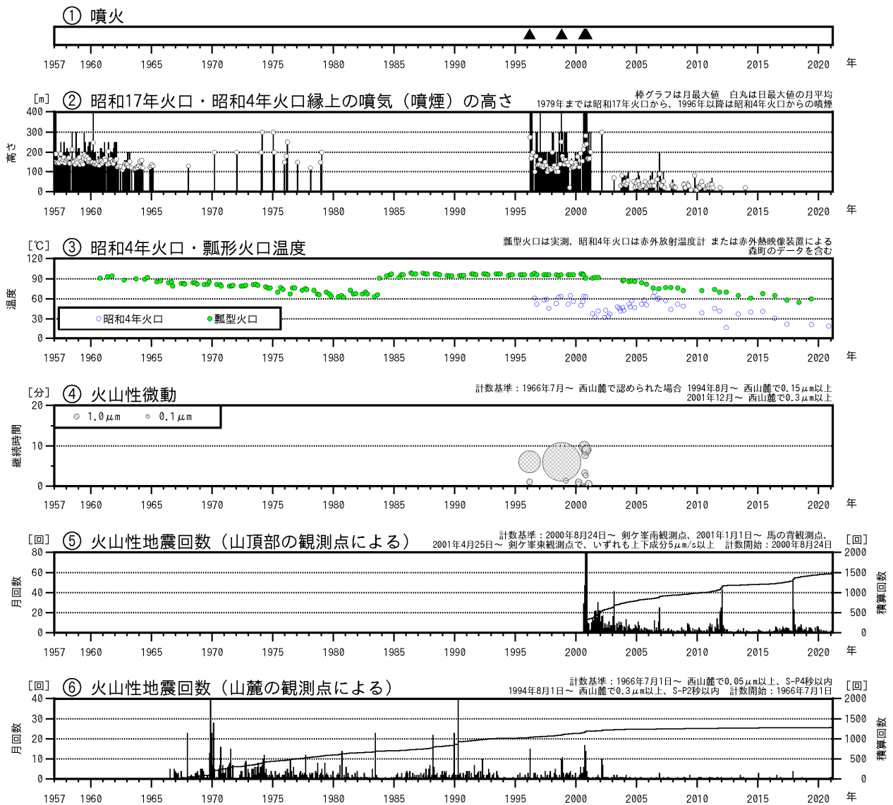
図1 北海道駒ヶ岳 火山活動経過図（1957年1月～2021年2月）
