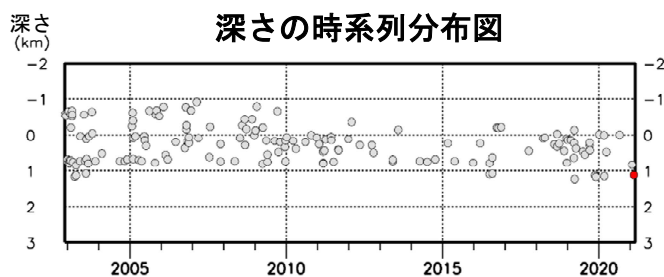
図4 北海道駒ヶ岳 火山性地震の震源分布（2002年12月～2021年2月）
