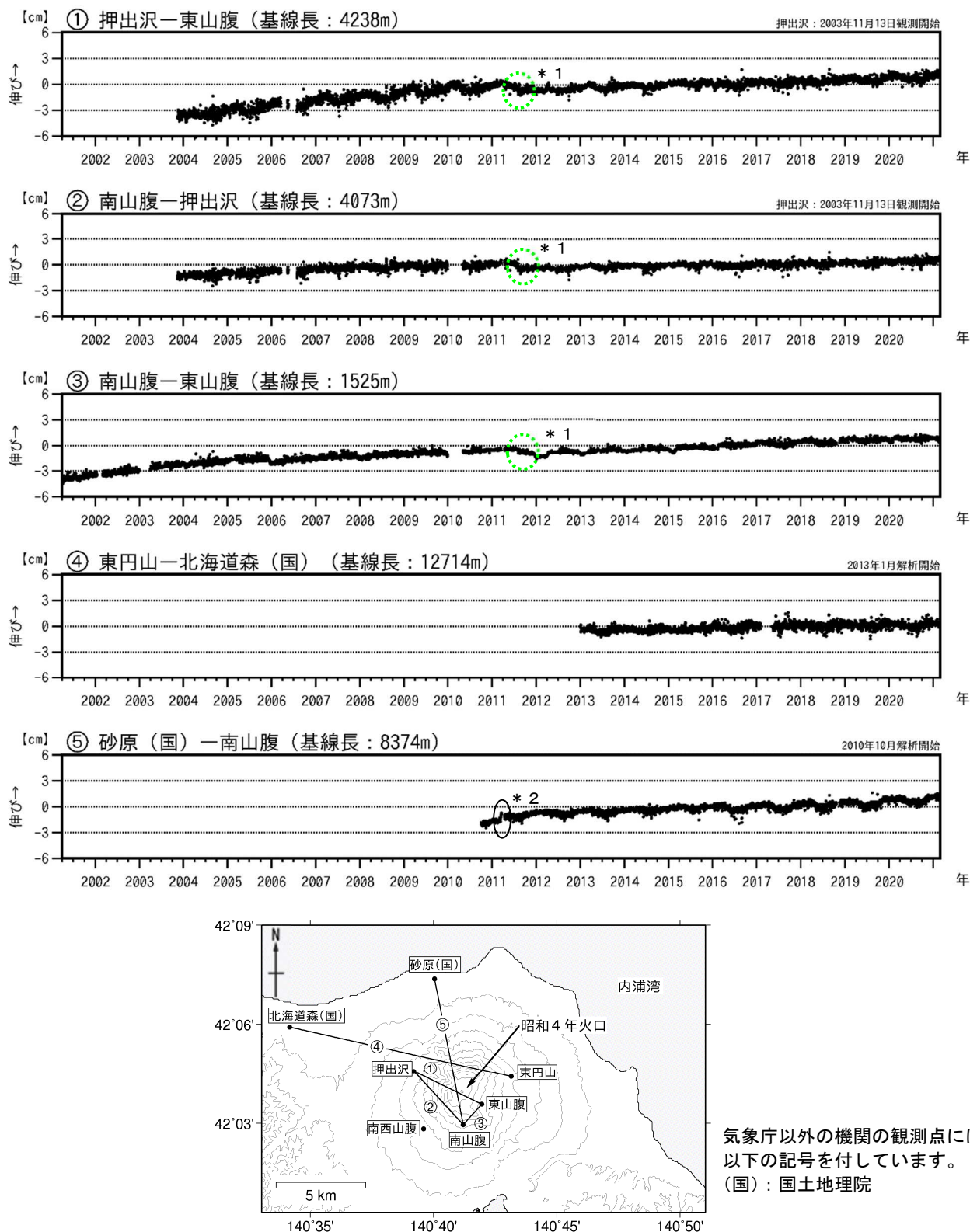
図5 北海道駒ヶ岳 GNSS連続観測による基線長変化（2001年4月～2021年2月）及び観測点配置図
