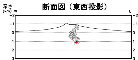
図4 北海道駒ヶ岳 火山性地震の震源分布（2002年12月～2021年2月）
