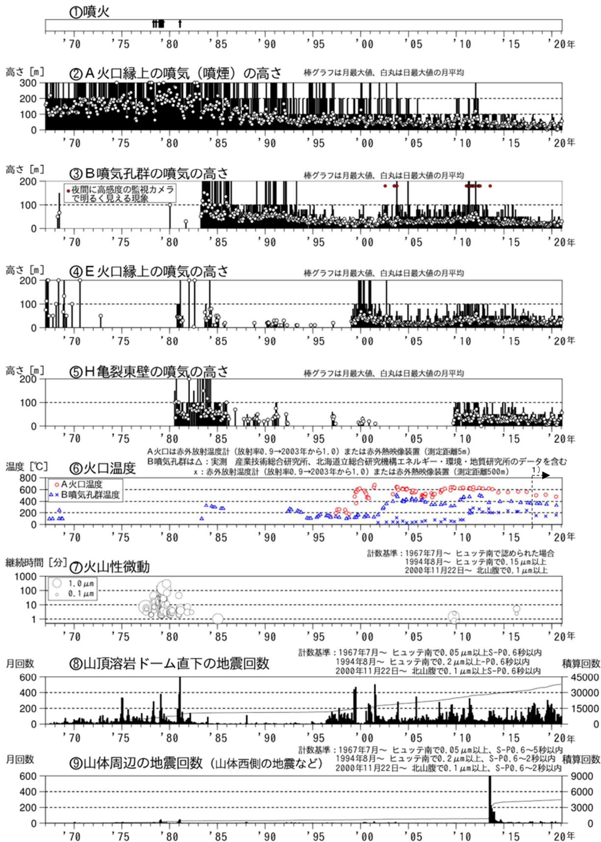
図1 樽前山 火山活動経過図(1967年1月~2021年1月)
