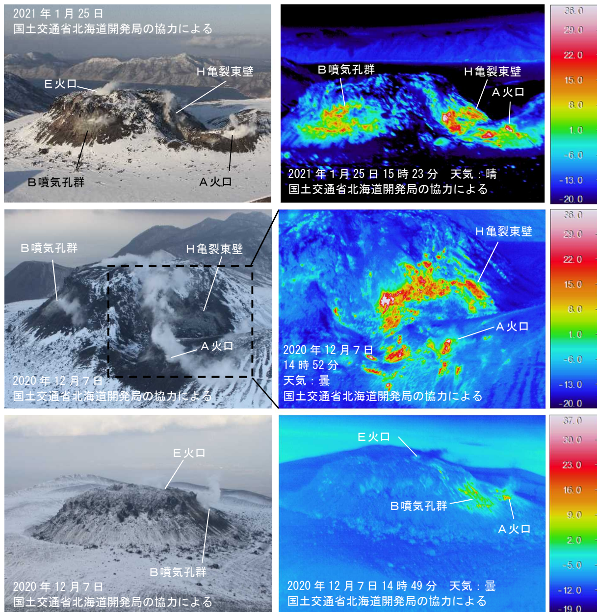
図5 樽前山 赤外熱映像装置による山頂溶岩ドーム西側と南側の地表面温度分布 上：南側上空（図3の③）から撮影 中：南東側上空（図3の④）から撮影 下：西側上空（図3の⑤）から撮影 ・山頂溶岩ドームの噴気や地表面温度分布の状況に変化は認められませんでした。
