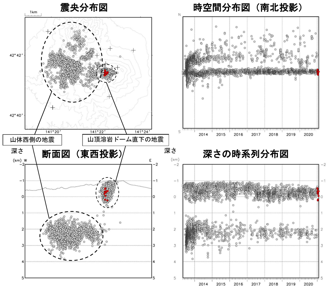
図6 樽前山 火山性地震の震源分布（2013年5月～2021年1月） ●印：2013年5月～2020年12月の震源、●印：2021年1月の震源、+印：地震観測点 2017年10月31日以降、震源計算に利用する観測点を変更しています。 ・地震は山頂溶岩ドーム直下の標高0km付近で発生しました。
