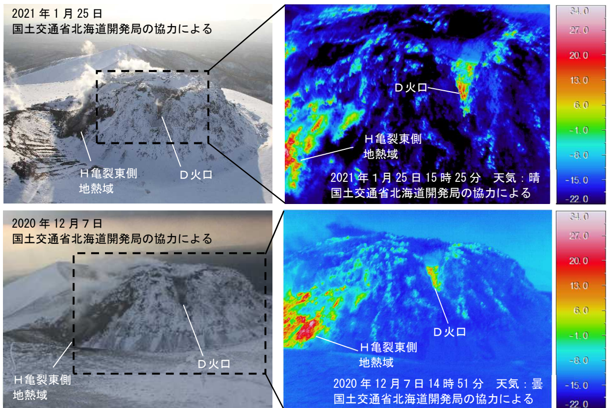
図4 樽前山 赤外熱映像装置による山頂溶岩ドーム北東側の状況及び地表面温度分布 上：東側上空（図3の①）から撮影 下：東側上空（図3の②）から撮影 ・山頂溶岩ドームの噴気や地表面温度分布の状況に変化は認められませんでした。
