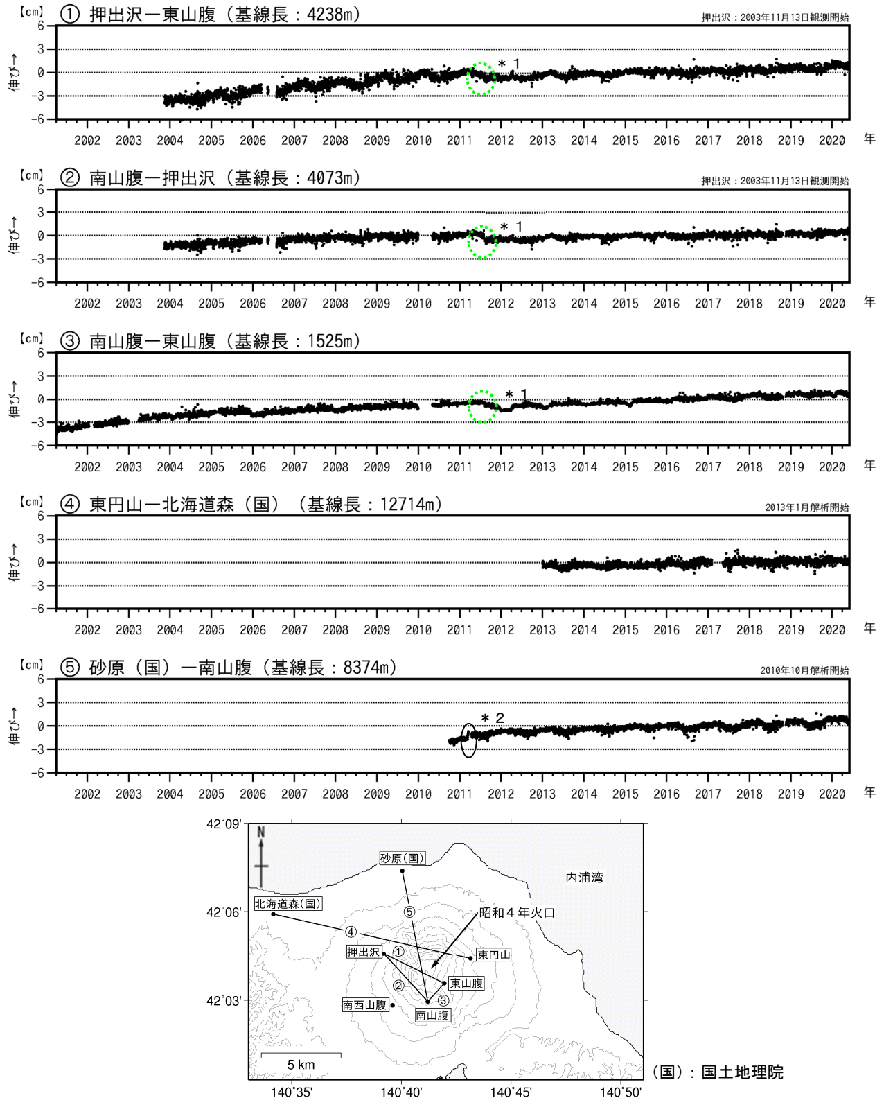
図5 北海道駒ヶ岳 GNSS連続観測による基線長変化（2001年4月～2020年5月）及び観測点配置図 GNSS基線①～⑤は観測点配置図の①～⑤に対応しています。 GNSS基線の空白部分は欠測を示します。 ①～③の緑点線円内の変動（＊1）は、機器更新によるものです。 ⑤の黒点線円内の変動（＊2）は、2011年3月11日に発生した「平成23年（2011年）東北地方太平洋沖地震」の影響によるものです。 2010年10月及び2016年1月に解析方法を変更しています
