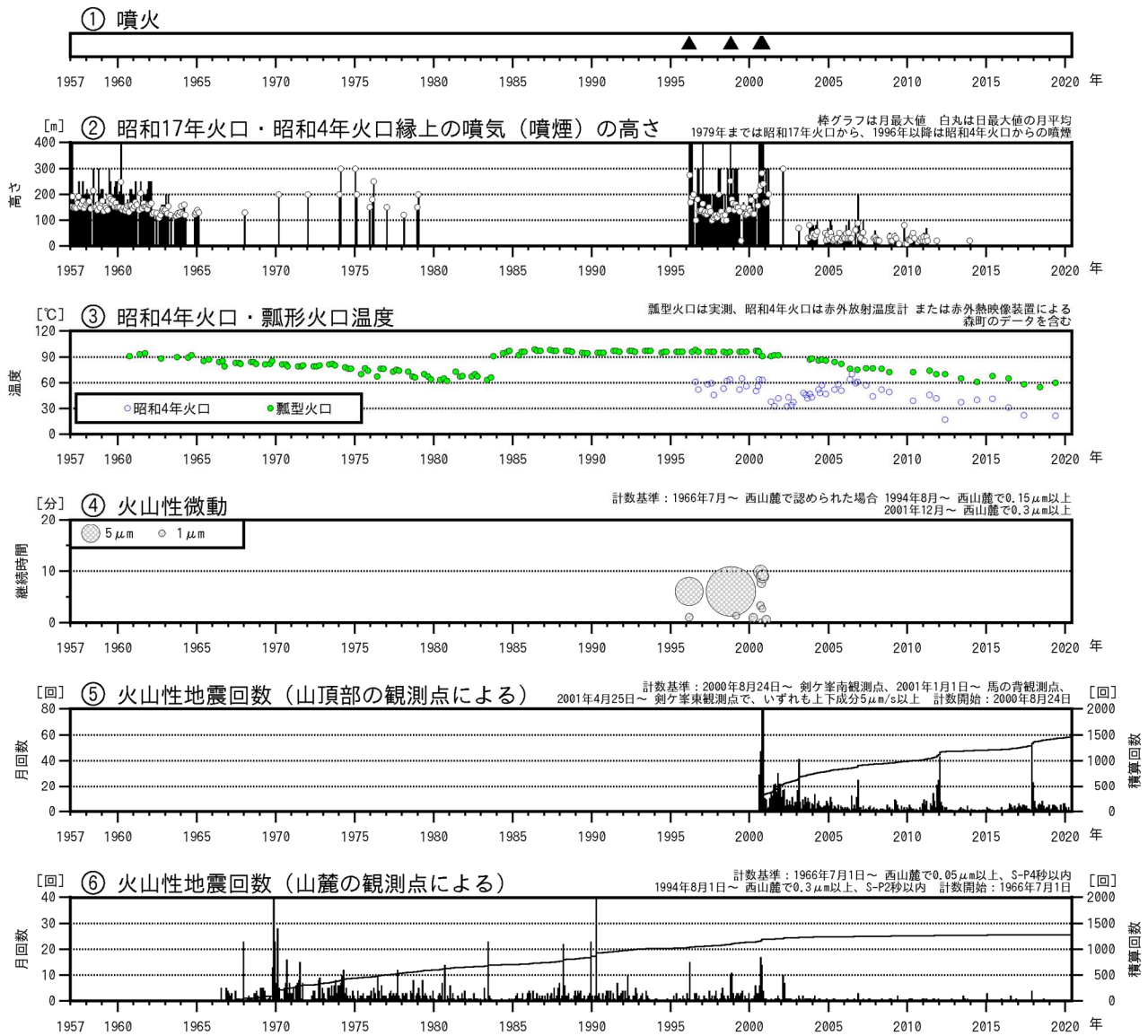
図1 北海道駒ヶ岳 火山活動経過図（1957年1月～2020年5月）
