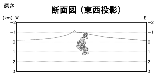
図4 北海道駒ヶ岳 火山性地震の震源分布（2002年12月～2020年5月）
