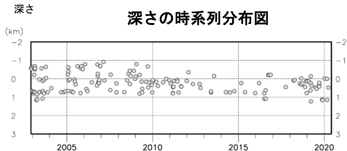
図4 北海道駒ヶ岳 火山性地震の震源分布（2002年12月～2020年5月）
