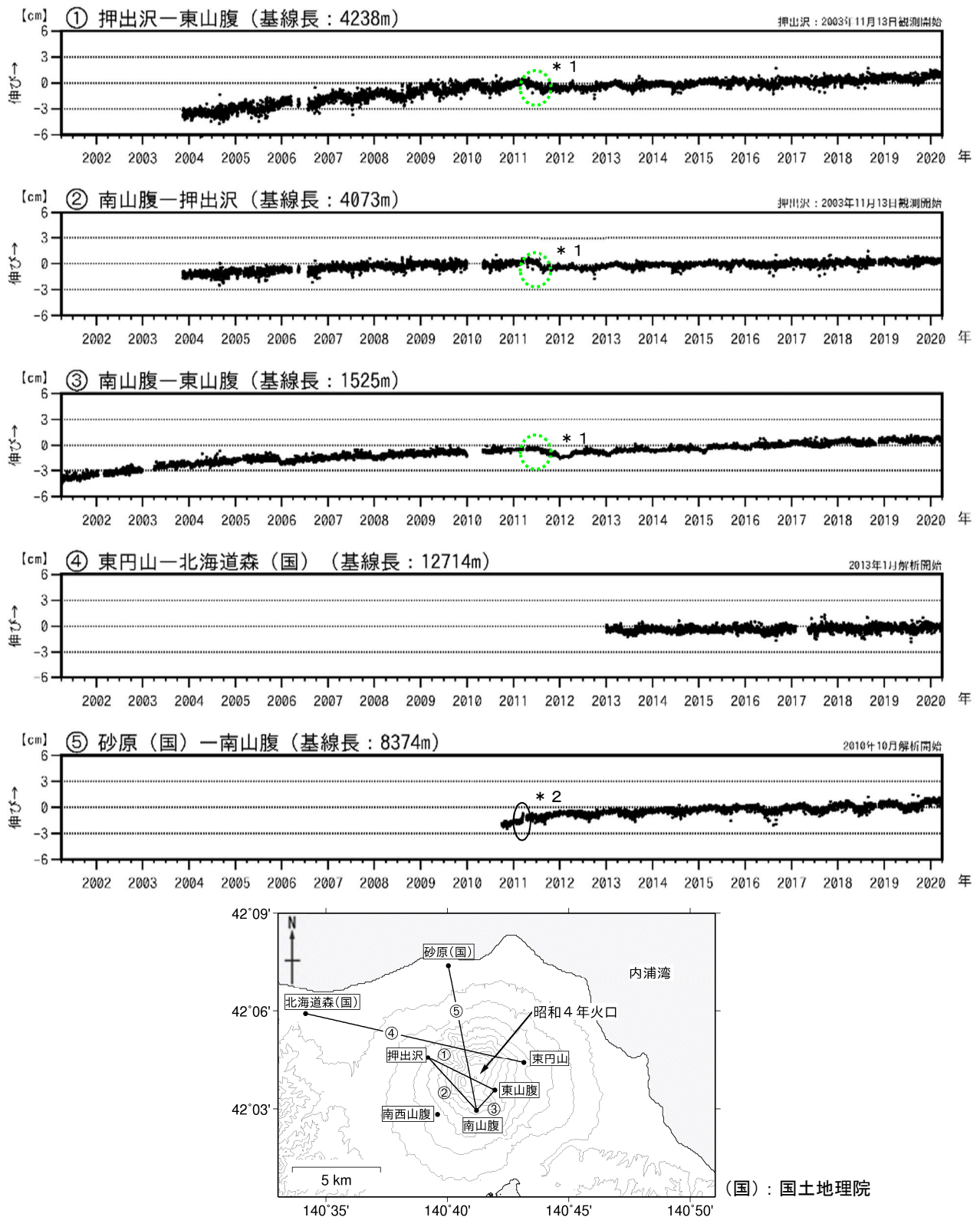
図5 北海道駒ヶ岳 GNSS連続観測による基線長変化（2001年4月～2020年3月）及び観測点配置図 GNSS基線①～⑤は観測点配置図の①～⑤に対応しています。 GNSS基線の空白部分は欠測を示します。 ①～③の緑点線円内の変動（* 1）は、機器更新によるものです。 ⑤の黒点線円内の変動（* 2）は、2011年3月11日に発生した「平成23年（2011年）東北地方太平洋沖地震」の影響によるものです。 2010年10月及び2016年1月に解析方法を変更しています
