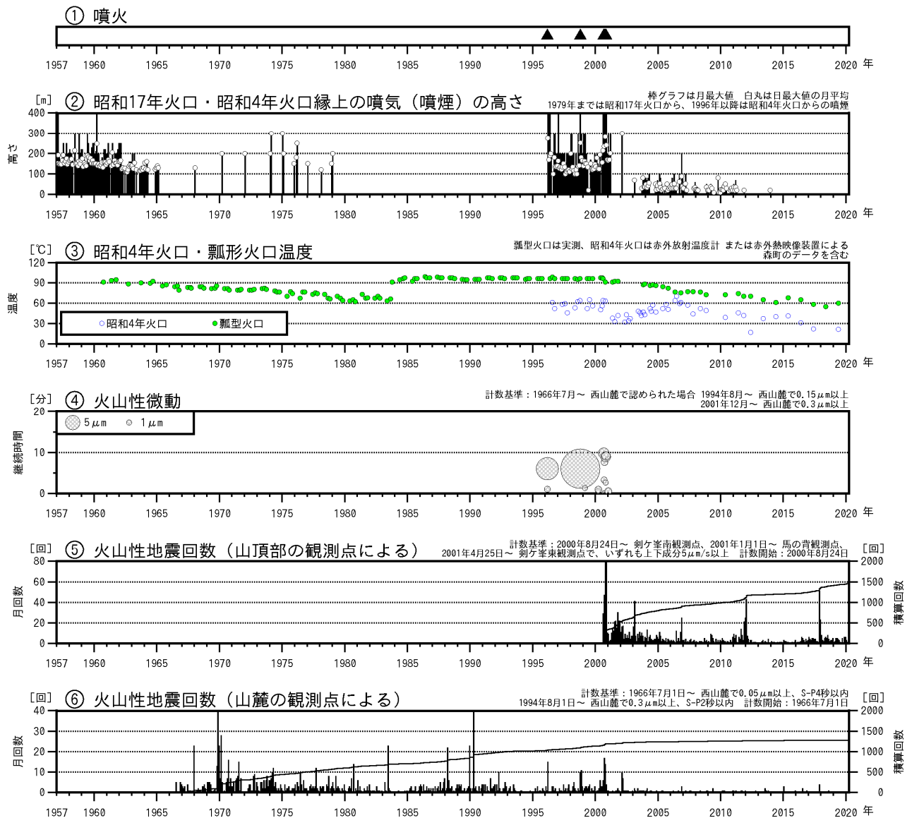
図1 北海道駒ヶ岳 火山活動経過図（1957年1月～2020年3月）
