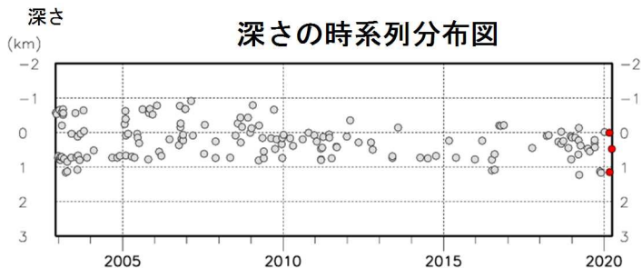
図4 北海道駒ヶ岳 火山性地震の震源分布（2002年12月～2020年3月）
