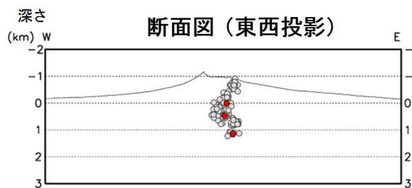
図4 北海道駒ヶ岳 火山性地震の震源分布（2002年12月～2020年3月）
