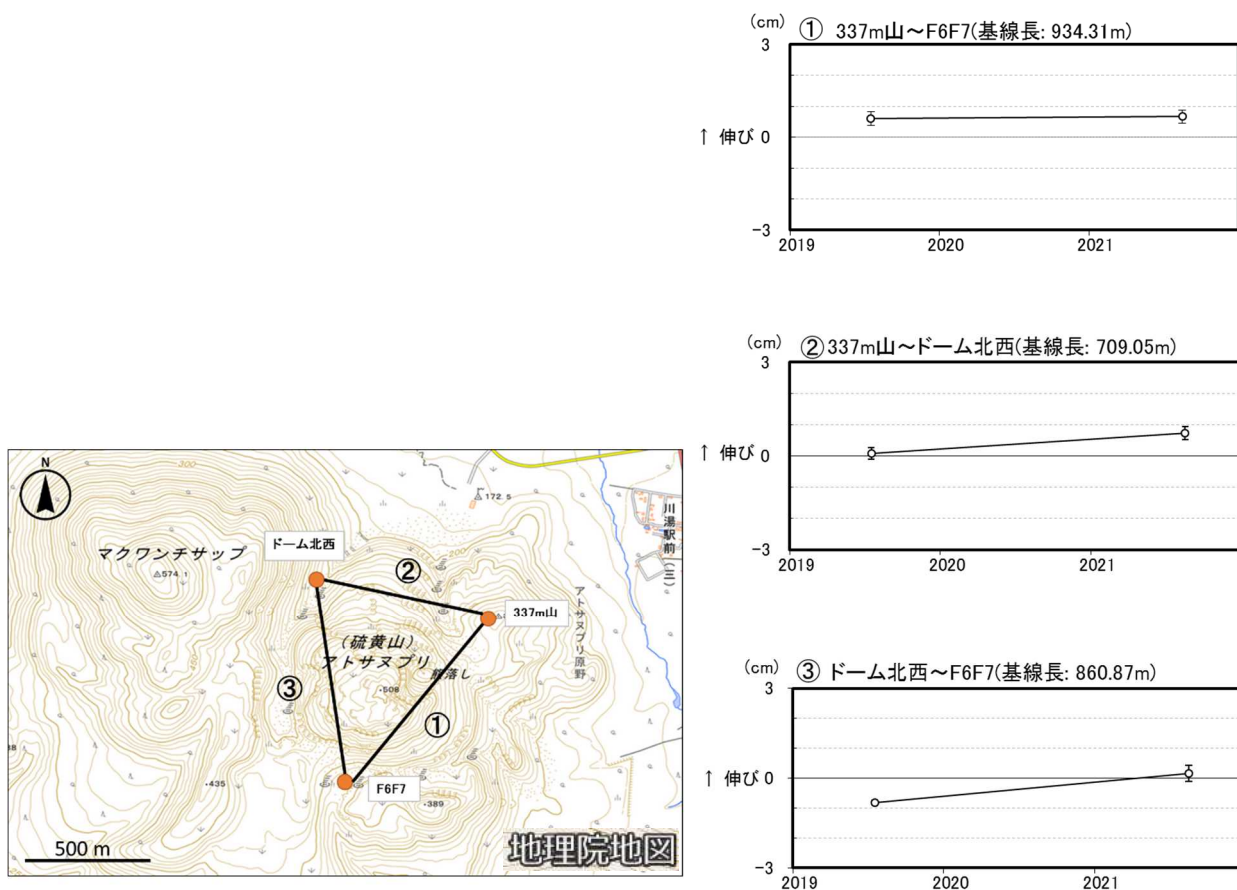
図11 アトサヌプリ GNSS繰り返し観測による基線長変化及び観測点配置図 (2019年8月～2021年8月) ・前回の観測 (2019年8月) に比べて、特段の変化は認められませんでした。
