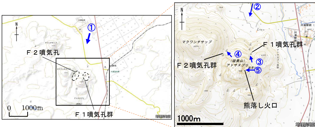
図3 アトサヌプリ 周辺図と写真及び赤外熱映像の撮影方向（矢印）
