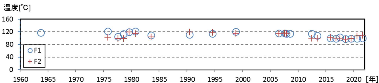
図6 アトサヌプリ 熱電対温度計によるF 1・F 2噴気孔群の最高温度（1963年～2021年） ・ F 1噴気孔群及びF 2噴気孔群の噴気温度は100°C前後で推移しています。
