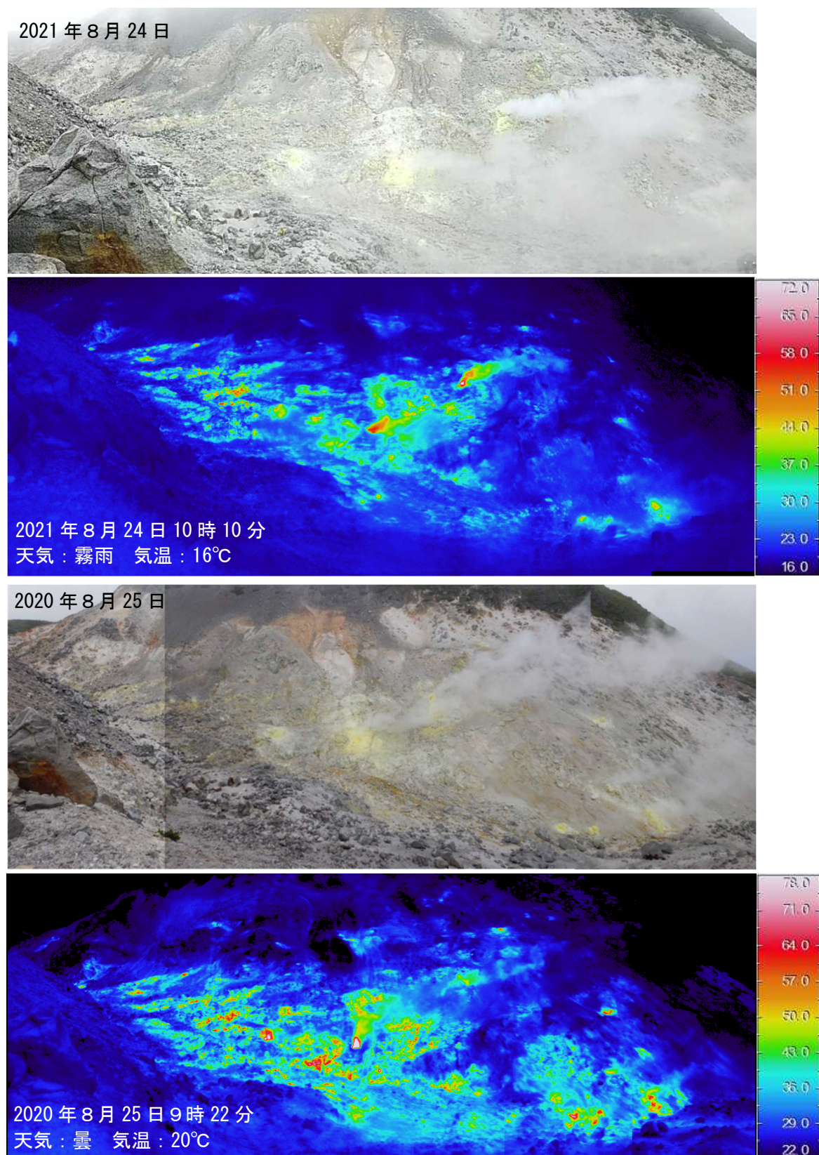
図8 アトサヌプリ 赤外熱映像装置によるF2噴気孔群の地表面温度分布
