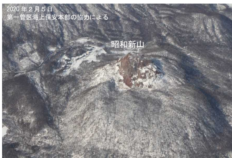
図5 有珠山 昭和新山の状況 南東側上空（図2-③）から撮影 ・ 昭和新山の噴気の状況に異常は認められませんでした。
