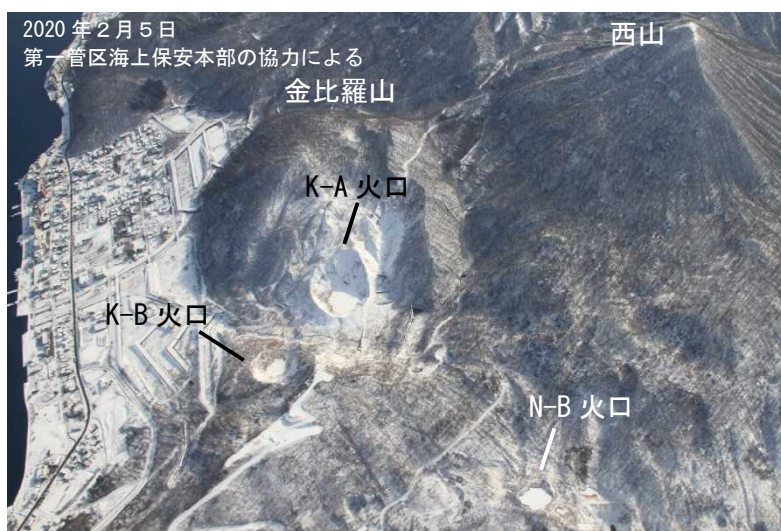
図4 有珠山 金比羅山火口群・西山火口群の状況 西側上空（図2-②）から撮影 ・ K-A火口、K-B火口及びN-B火口等において異常は認められませんでした。
