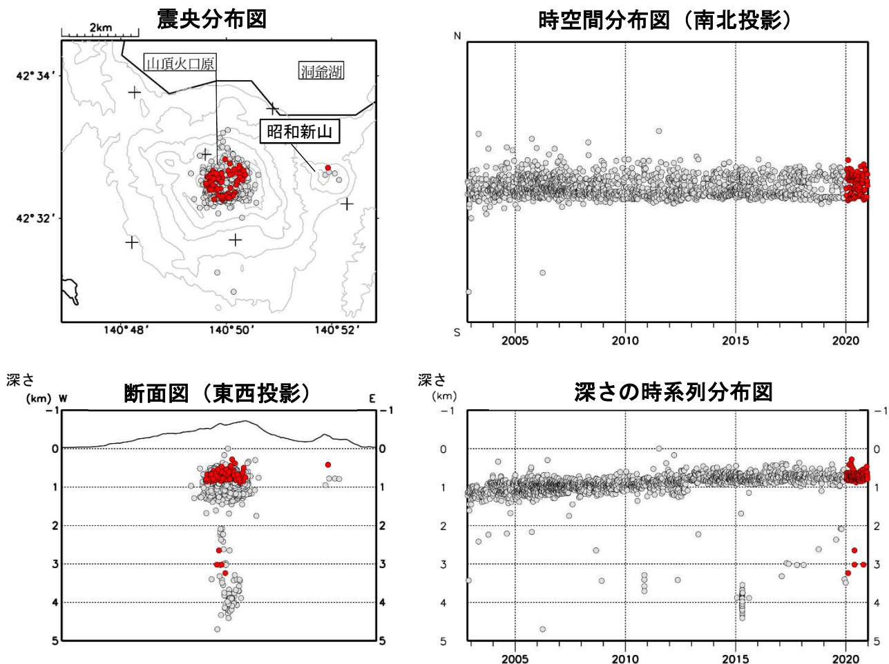
図9 有珠山 火山性地震の震源分布（2002年12月～2020年12月） ●印：2002年12月～2019年12月の震源 ●印：2020年の震源 +印：地震観測点 ・地震は、山頂火口原直下と昭和新山直下で発生しました。
