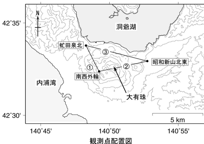
図10 有珠山 GNSS連続観測による基線長変化（2001年4月～2020年12月）及び観測点配置図
