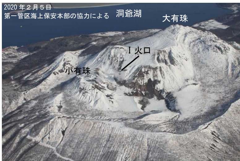
図3 有珠山 山頂火口原周辺の状況 南西側上空（図2-①）から撮影 ・ I火口周辺の噴気の状況に異常は認められませんでした。
