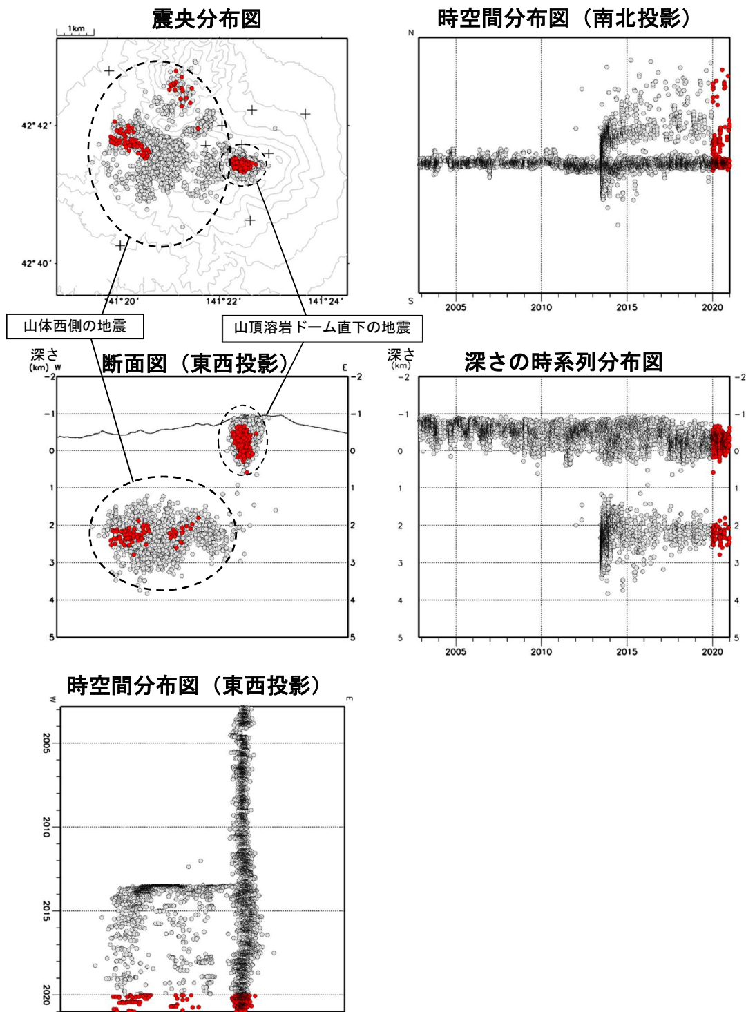
図11 樽前山 火山性地震の震源分布 (2002年11月～2020年12月)
