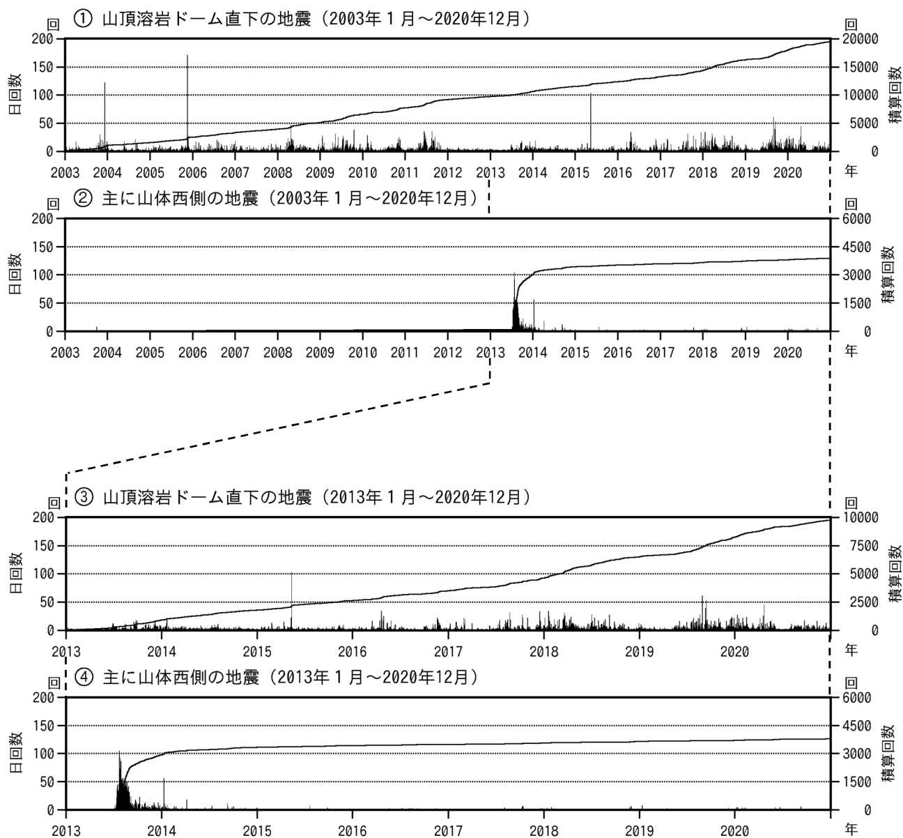
図10 樽前山 発生場所別の火山性地震の日回数及び積算回数
