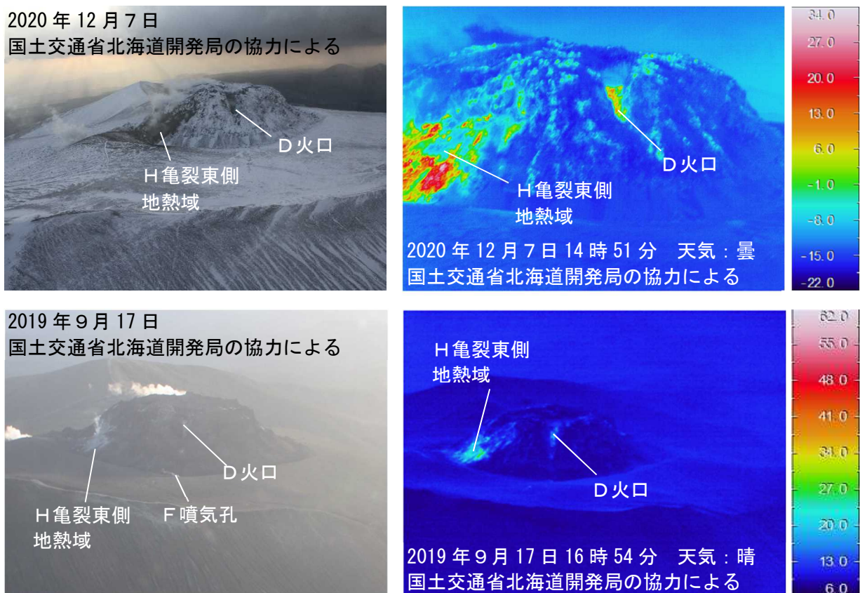
図5 樽前山 赤外熱映像装置による山頂溶岩ドーム東側の状況及び地表面温度分布 上：東側上空（図3の②）から撮影 下：北東側上空（図3の③）から撮影 ・山頂溶岩ドームの噴気や地表面温度分布の状況に変化は認められませんでした。
