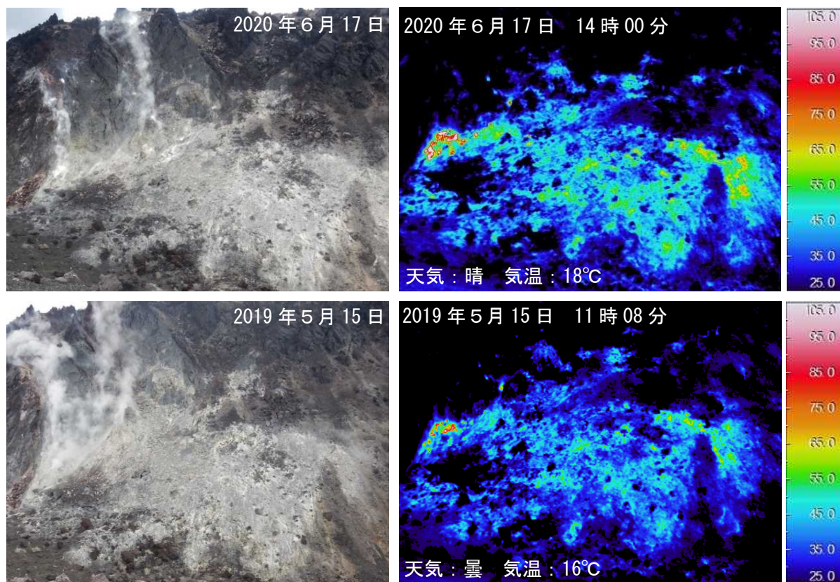
図9 樽前山 赤外熱映像装置によるH亀裂東壁の地表面温度分布 東側（図3の㊸）から撮影 ・H亀裂東壁では、地表面温度分布に変化は認められませんでした。
