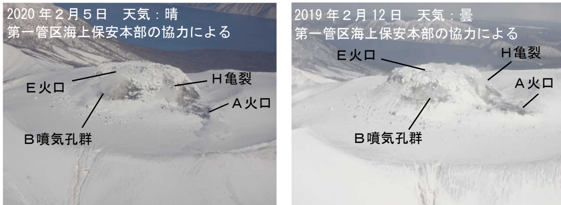
図4 樽前山 山頂溶岩ドームの状況 南側上空（図3の①）から撮影 ・山頂溶岩ドームの噴気の状態や融雪域の広がりに変化は認められませんでした。
