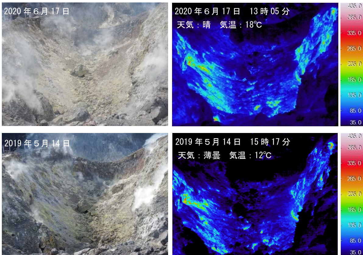
図7 樽前山 赤外熱映像装置によるA火口の地表面温度分布 南側(図3の㉗)から撮影 ・A火口では、地表面温度分布に変化は認められませんでした。
