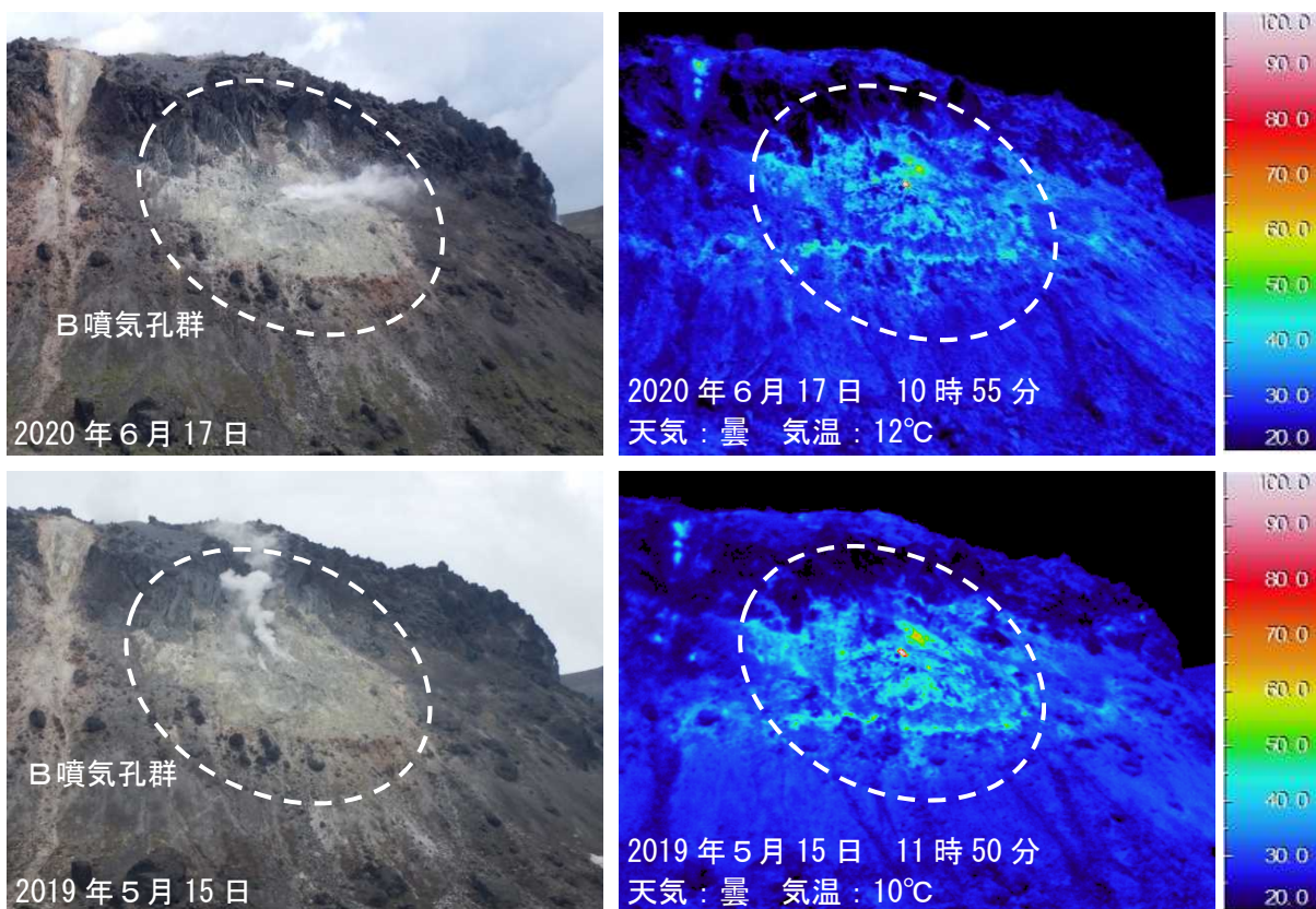
図8 樽前山 赤外熱映像装置によるB噴気孔群の地表面温度分布 南西側(図3の㉘)から撮影 ・B噴気孔群では、地表面温度分布に変化は認められませんでした。
