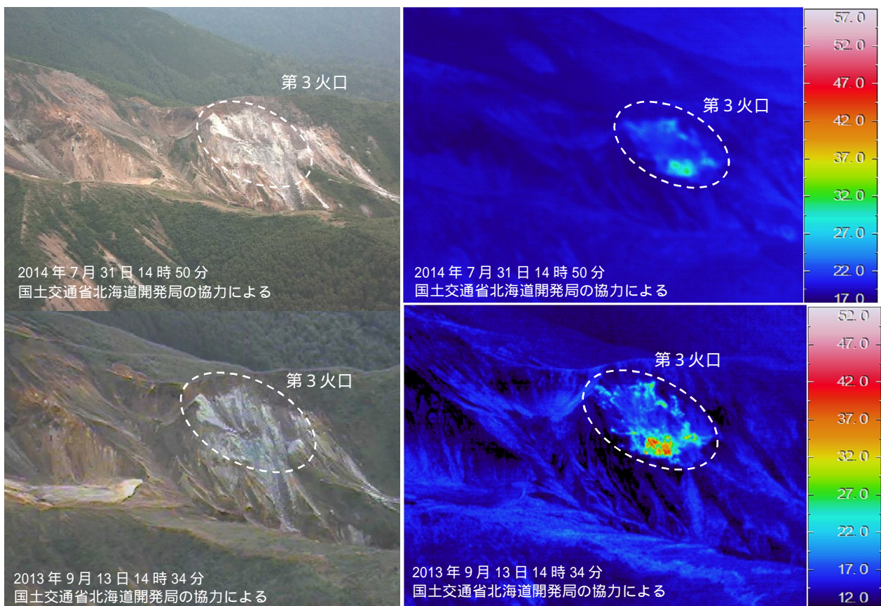
図3 赤外熱映像装置による第3火口の地表面温度分布 上：図1- から撮影 下：図1- から撮影
