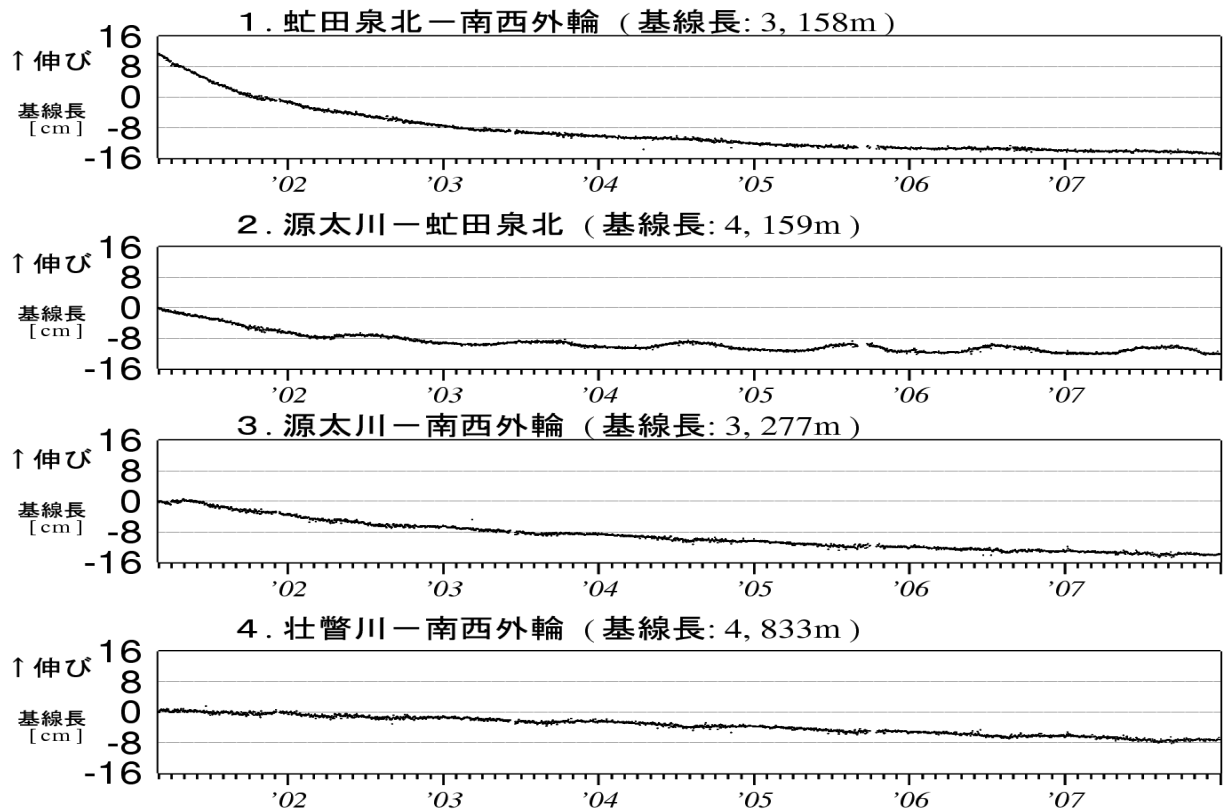
図9 有珠山 GPS 連続観測による基線長変化 (2001年3月～2007年12月)
