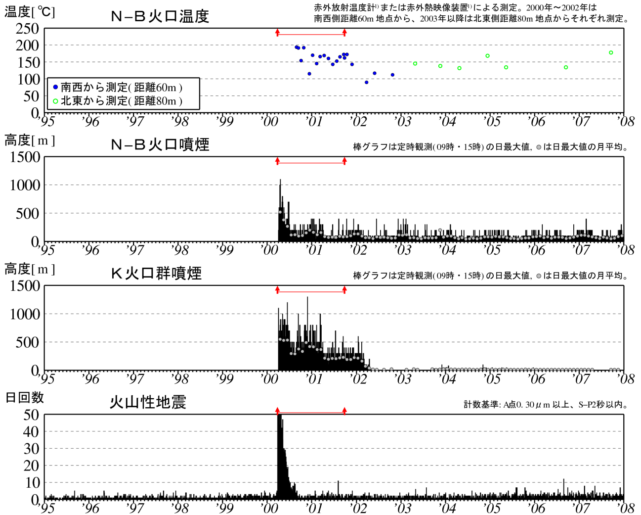
図1 有珠山 近年の火山活動経過図 (1995年1月～2007年12月)
