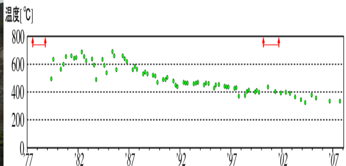
図 6 有珠山 I 火口の噴気温度 (1979 年～2007 年)
