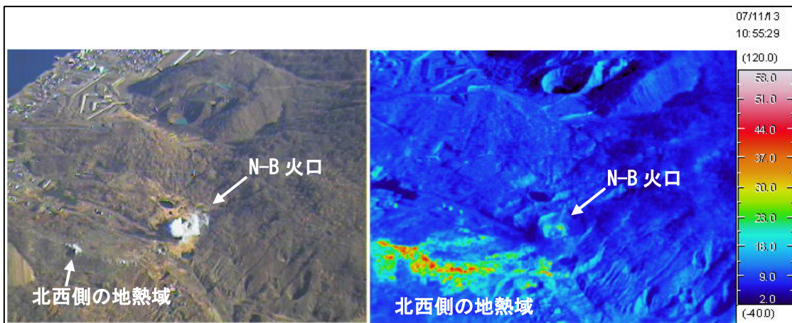
図 4 有珠山 赤外熱映像装置 1) による西山西麓火口群周辺の地表面温度分布 (2007 年 11 月 13 日 南西側上空から撮影)
