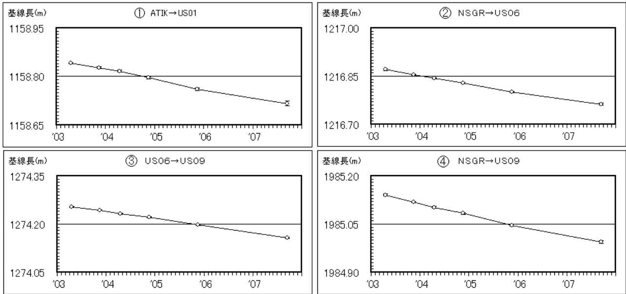
図 10 有珠山 GPS 繰り返し観測による火口付近の基線長変化 (2003 年 4 月～2007 年 9 月、図 10 の①～④は図 11 の基線①～④に対応しています。)
