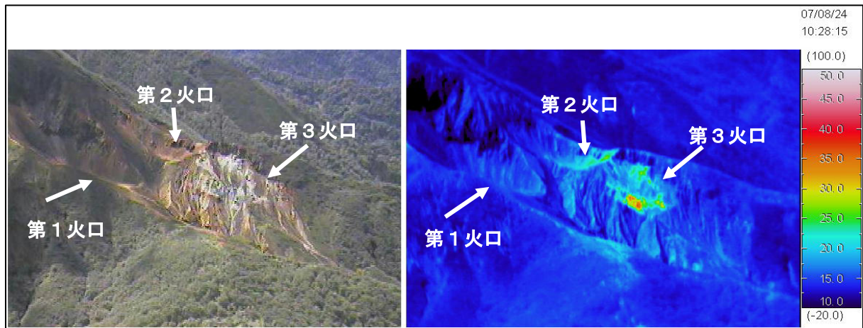
図 3 丸山 赤外熱映像装置 1) による北西斜面火口列の地表面温度分布 (2007年8月24日 図1 ②方向から撮影)
