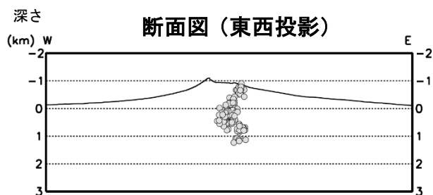
図4 北海道駒ヶ岳 火山性地震の震源分布（2002年12月～2019年12月）
