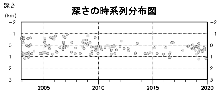
図4 北海道駒ヶ岳 火山性地震の震源分布（2002年12月～2019年12月）
