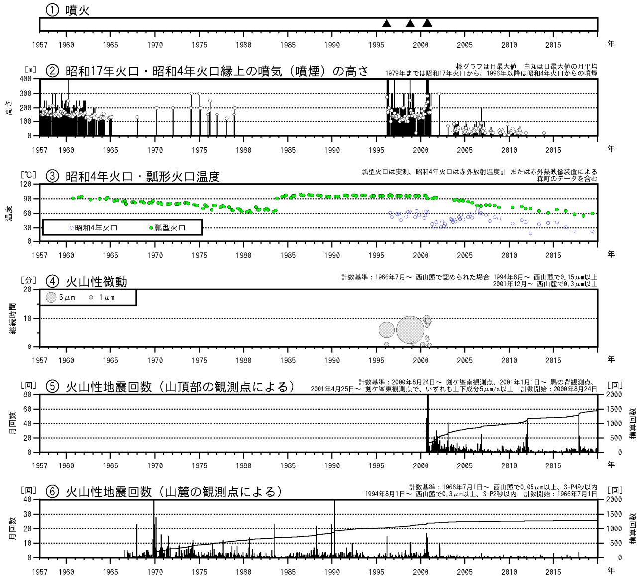
図1 北海道駒ヶ岳 火山活動経過図（1957年1月～2019年12月）
