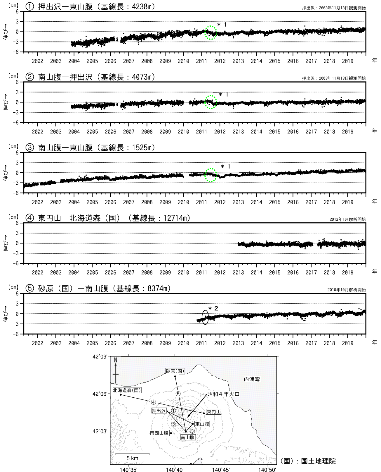
図5 北海道駒ヶ岳 GNSS連続観測による基線長変化（2001年4月～2019年12月）及び観測点配置図 GNSS基線①～⑤は観測点配置図の①～⑤に対応しています。 GNSS基線の空白部分は欠測を示します。 ①～③の緑点線円内の変動（＊1）は、機器更新によるものです。 ⑤の黒楕円内の変動（＊2）は、2011年3月11日に発生した「平成23年（2011年）東北地方太平洋沖地震」の影響によるものです。 2010年10月及び2016年1月に解析方法を変更しています。
