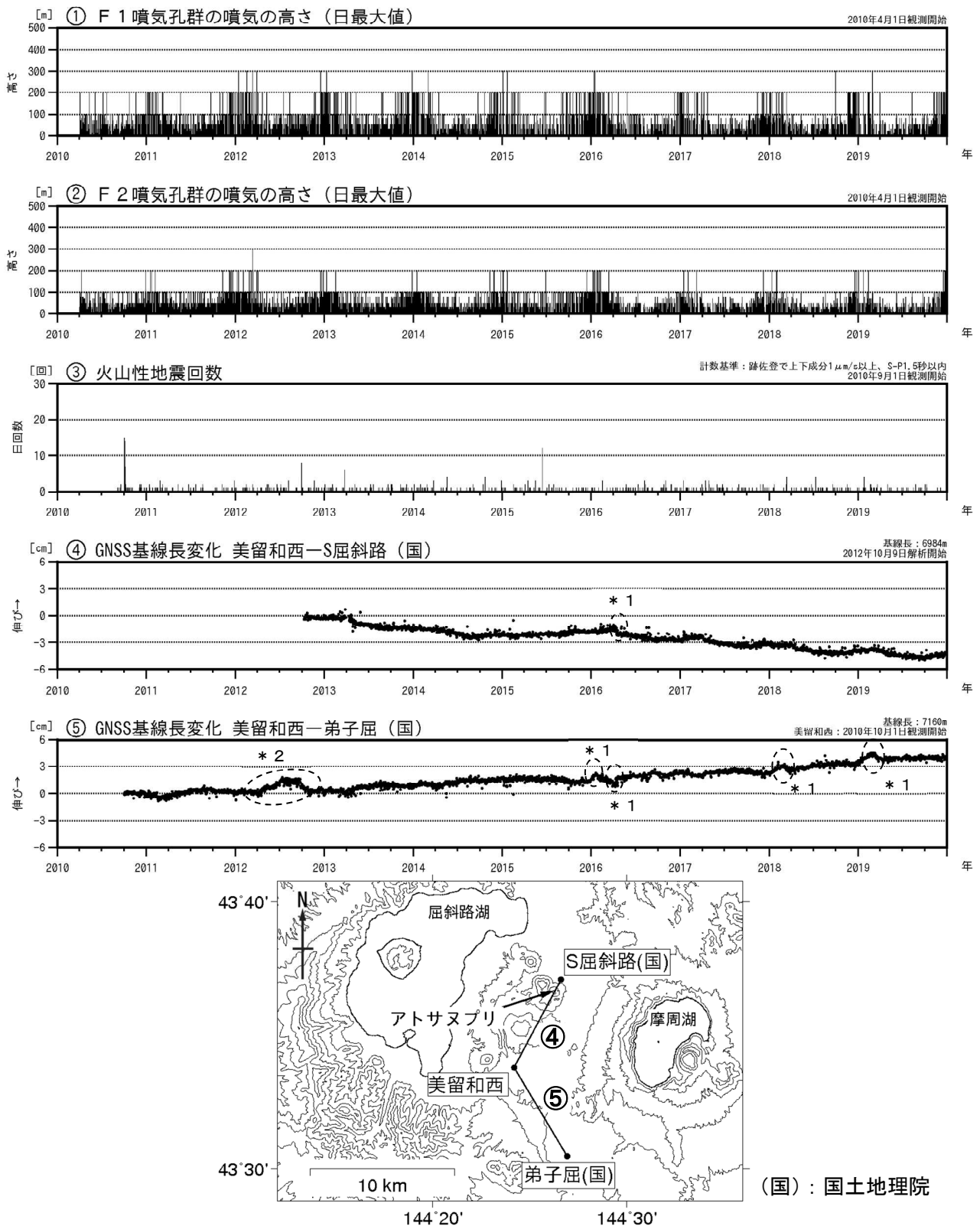
図1 アトサヌプリ 火山活動経過図（2010年4月～2019年12月）及びGNSS連続観測点配置図
