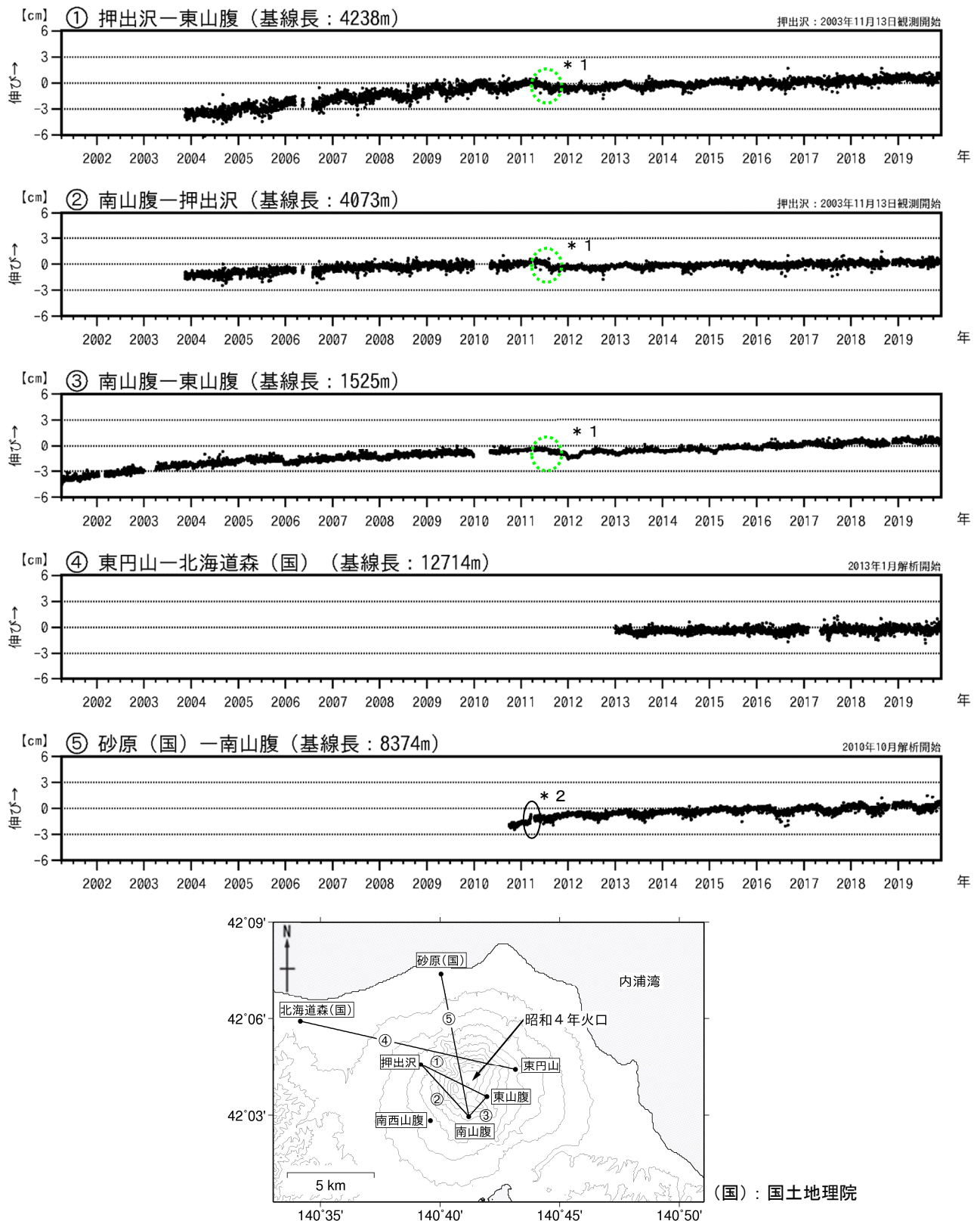
図5 北海道駒ヶ岳 GNSS連続観測による基線長変化（2001年4月～2019年11月）及び観測点配置図 GNSS基線①～⑤は観測点配置図の①～⑤に対応しています。 GNSS基線の空白部分は欠測を示します。 ①～③の緑点線円内の変動（＊1）は、機器更新によるものです。 ⑤の黒楕円内の変動（＊2）は、2011年3月11日に発生した「平成23年（2011年）東北地方太平洋沖地震」の影響によるものです。 2010年10月及び2016年1月に解析方法を変更しています。
