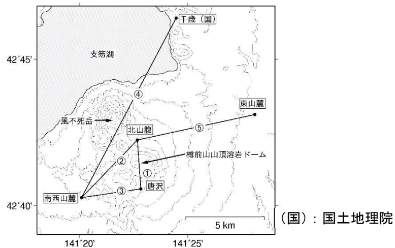
図7 樽前山 GNSS連続観測による基線長変化（2005年1月～2019年9月）及び観測点配置図 GNSS基線①～⑤は観測点配置図の①～⑤に対応しています。 GNSS基線の空白部分は欠測を示します。 ①、②の緑点線円内の変動（*1）は機器更新によるものです。 ②～④の黒楕円内の変動（*2）は、2014年7月8日に発生した胆振地方中東部の地震によるものです。 2010年10月及び2016年1月に解析方法を変更しています。
