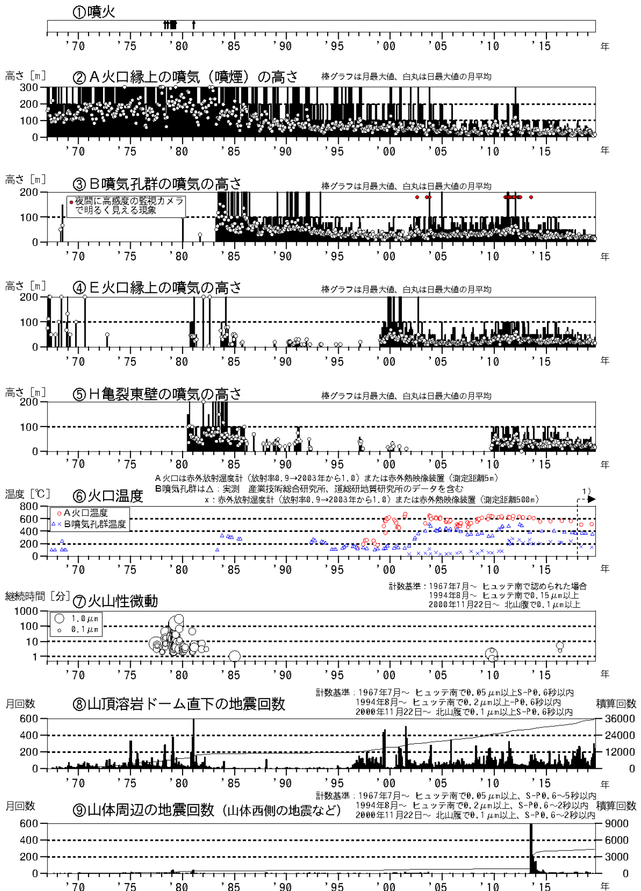
図1 樽前山 火山活動経過図（1967年1月～2019年9月）
