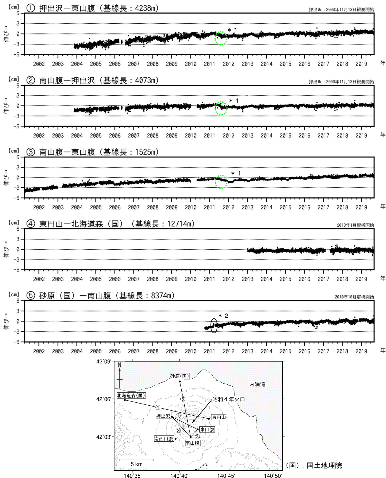
図5 北海道駒ヶ岳 GNSS連続観測による基線長変化（2001年4月～2019年8月）及び観測点配置図 GNSS基線①～⑤は観測点配置図の①～⑤に対応しています。 GNSS基線の空白部分は欠測を示します。 ①～③の緑点線内の変動（* 1）は、機器更新によるものです。 ⑤の黒点線内の変動（* 2）は、2011年3月11日に発生した「平成23年（2011年）東北地方太平洋沖地震」の影響によるものです。 2010年10月及び2016年1月に解析方法を変更しています。
