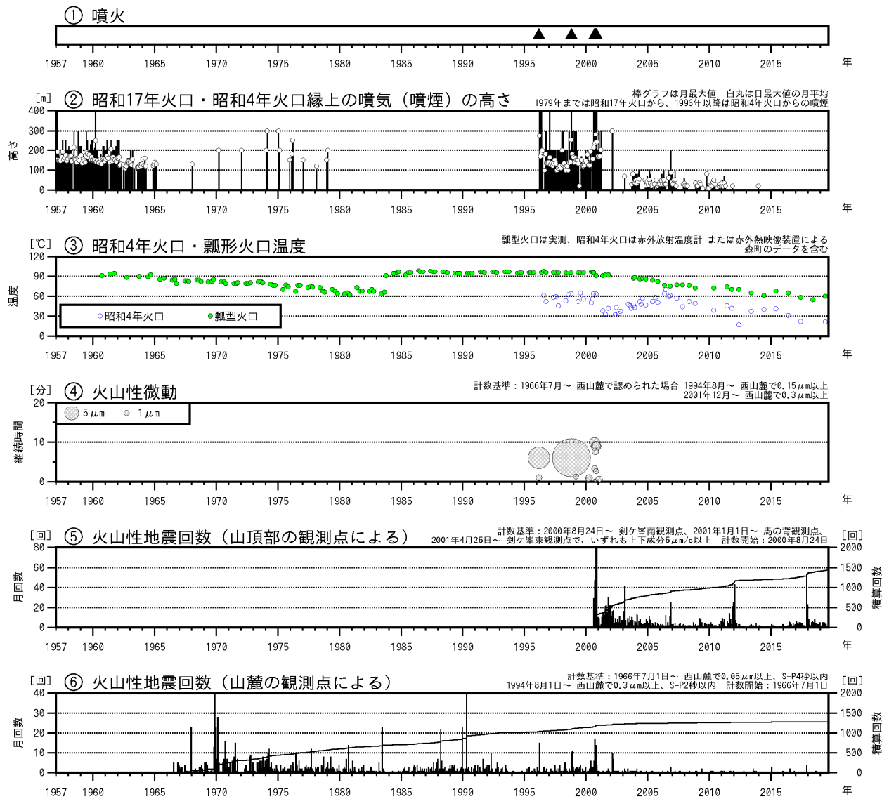
図1 北海道駒ヶ岳 火山活動経過図（1957年1月～2019年8月）
