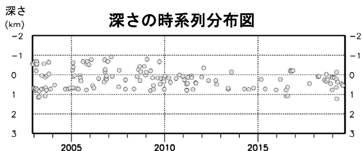
図4 北海道駒ヶ岳 火山性地震の震源分布（2002年12月～2019年8月）
