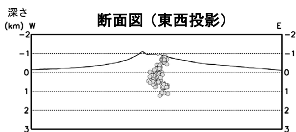
図4 北海道駒ヶ岳 火山性地震の震源分布（2002年12月～2019年8月）
