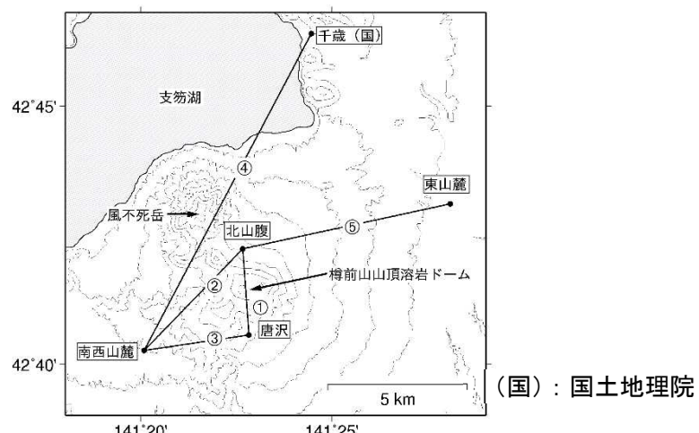
図7 樽前山 GNSS連続観測による基線長変化（2005年1月～2019年8月）及び観測点配置図 GNSS基線①～⑤は観測点配置図の①～⑤に対応しています。 GNSS基線の空白部分は欠測を示します。 ①、②の緑点線円内の変動（*1）は機器更新によるものです。 ②～④の黒楕円内の変動（*2）は、2014年7月8日に発生した胆振地方中東部の地震によるものです。 2010年10月及び2016年1月に解析方法を変更しています。
