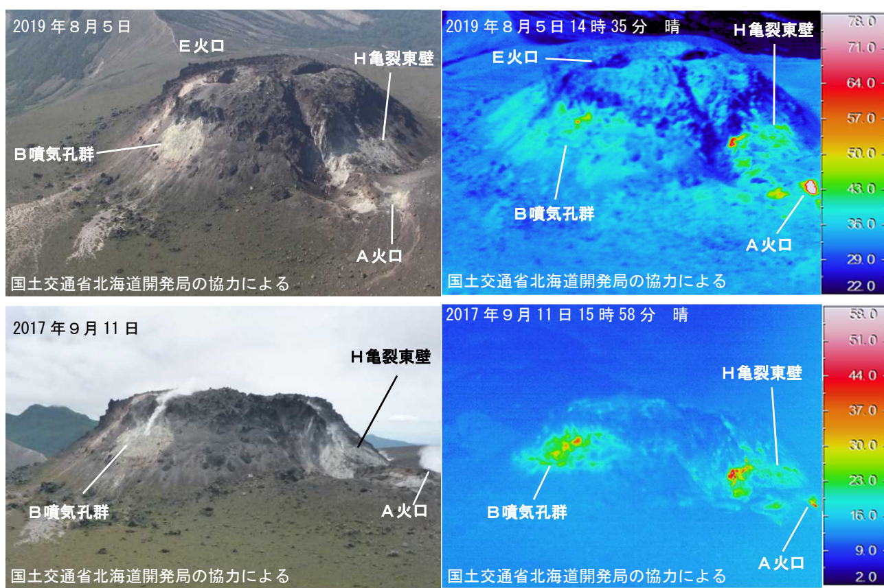
図5 樽前山 赤外熱映像装置による山頂溶岩ドーム周辺の地表面温度分布 南側上空（図3の②）から撮影 ・山頂溶岩ドームの噴気や地表面温度分布の状況に特段の変化は認められませんでした。
