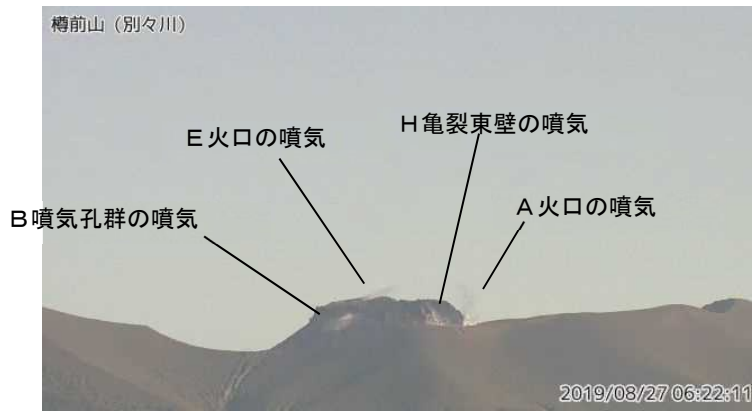
図2 樽前山 南側から見た山頂部の状況 (8月27日、別々川監視カメラによる)
