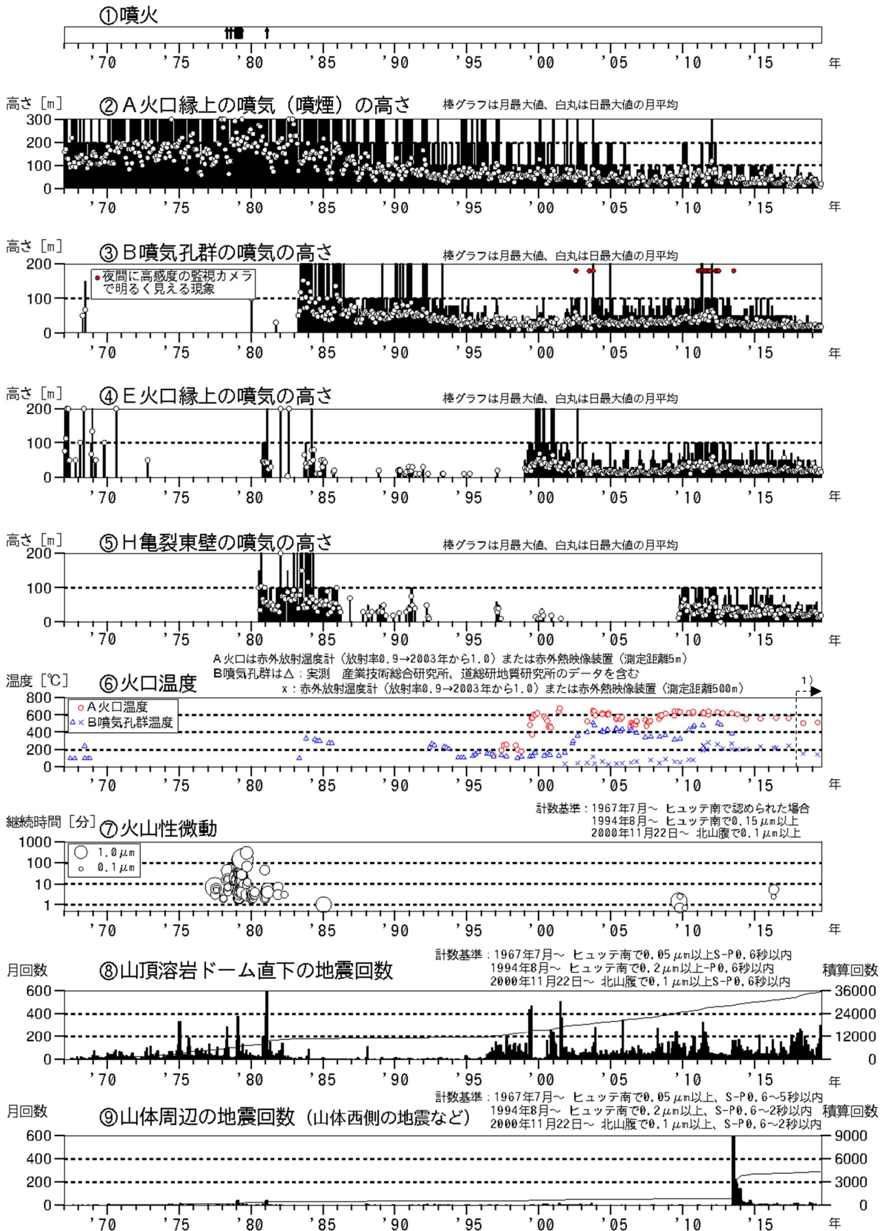
図1 樽前山 火山活動経過図（1967年1月～2019年8月）
