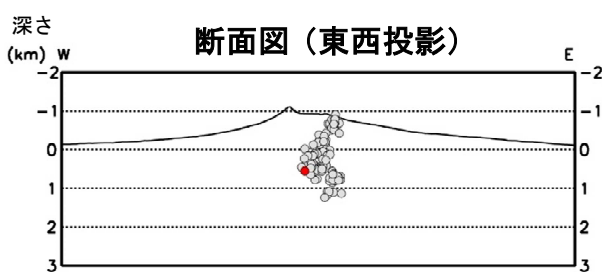
図4 北海道駒ヶ岳 火山性地震の震源分布（2002年12月～2019年7月）
