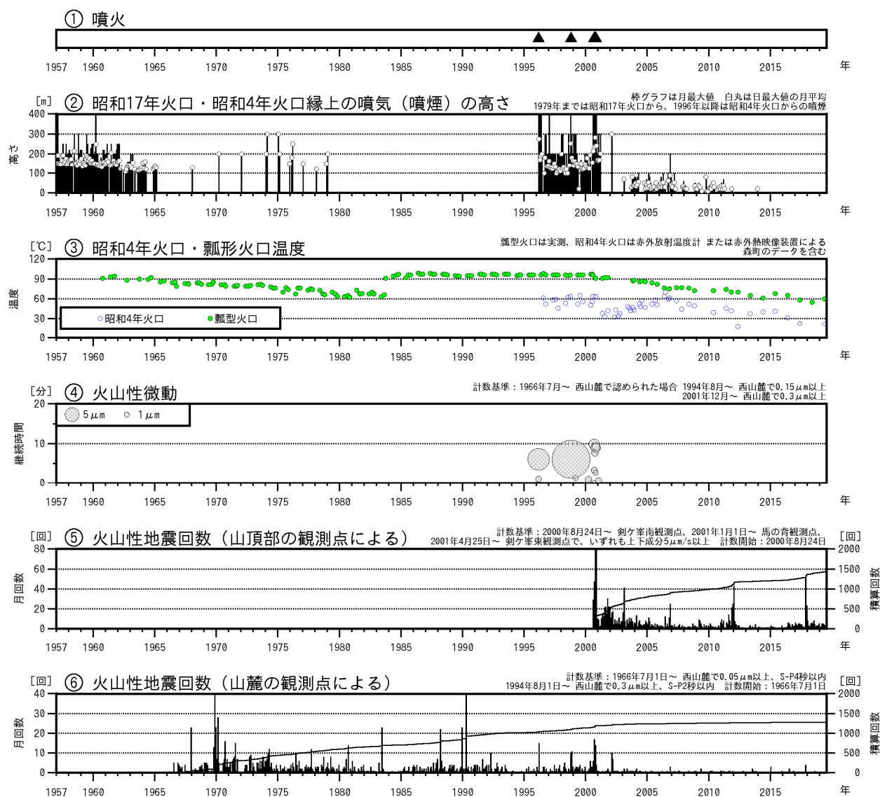
図1 北海道駒ヶ岳 火山活動経過図（1957年1月～2019年7月）
