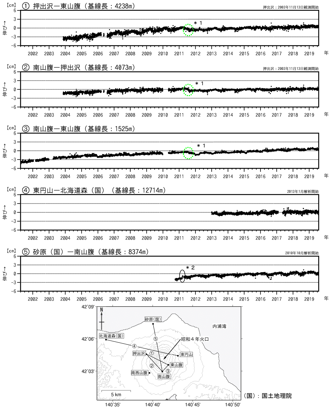
図5 北海道駒ヶ岳 GNSS連続観測による基線長変化（2001年4月～2019年7月）及び観測点配置図 GNSS基線①～⑤は観測点配置図の①～⑤に対応しています。 GNSS基線の空白部分は欠測を示します。 ①～③の緑点線円内の変動（*1）は、機器更新によるものです。 ⑤の黒点線円内の変動（*2）は、2011年3月11日に発生した「平成23年（2011年）東北地方太平洋沖地震」の影響によるものです。 2010年10月及び2016年1月に解析方法を変更しています。
