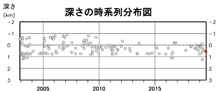
図4 北海道駒ヶ岳 火山性地震の震源分布（2002年12月～2019年7月）
