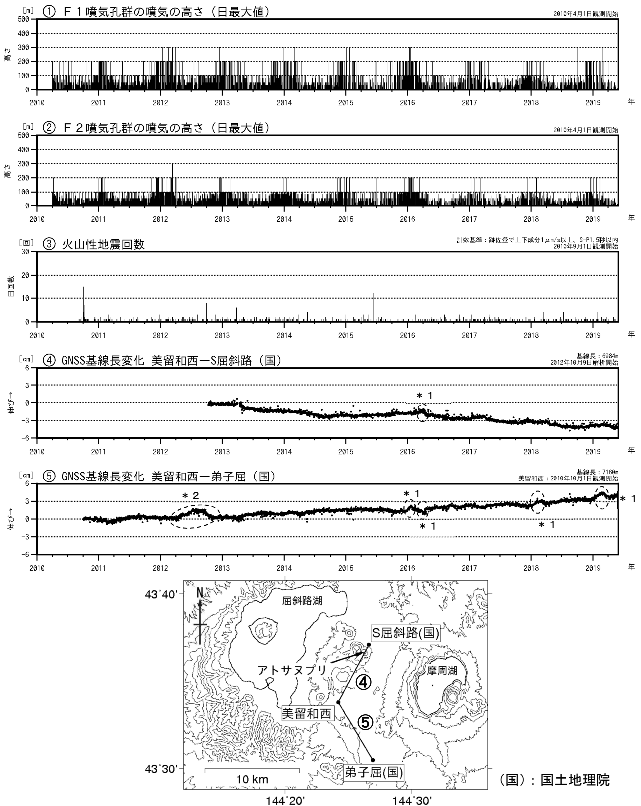
図1 アトサヌプリ 火山活動経過図（2010年4月～2019年5月）及びGNSS連続観測点配置図
