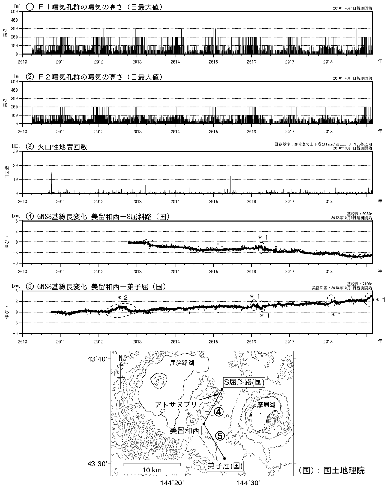
図1 アトサヌプリ 火山活動経過図（2010年4月～2019年2月）及びGNSS連続観測点配置図
