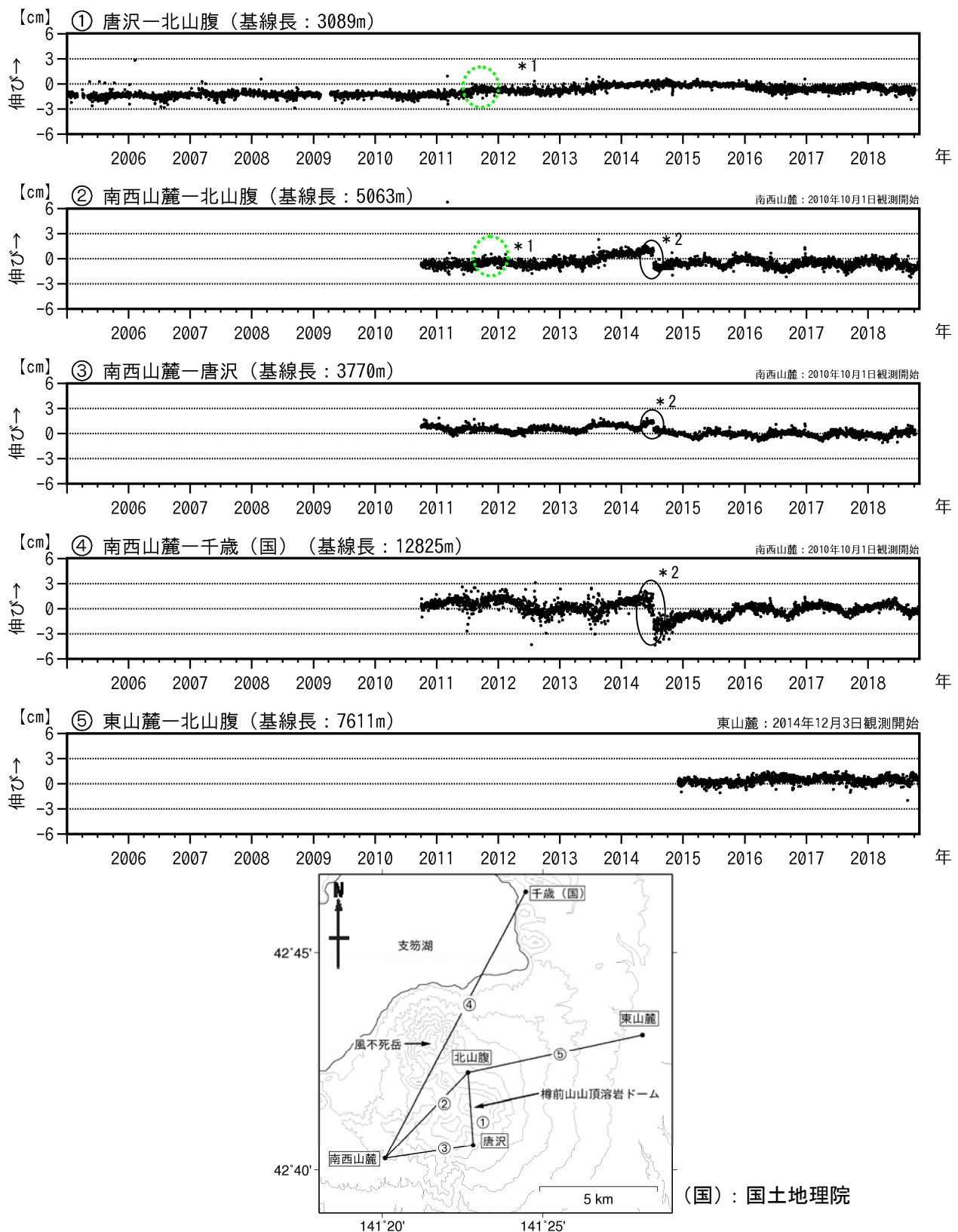
図7 樽前山 GNSS連続観測による基線長変化 (2005年1月~2018年10月) 及び観測点配置図
