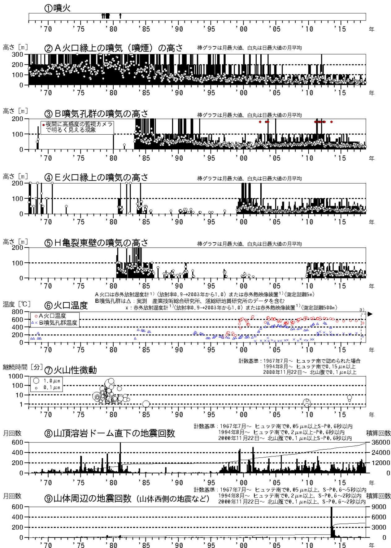
図1 樽前山 火山活動経過図(1967年1月~2018年10月)
