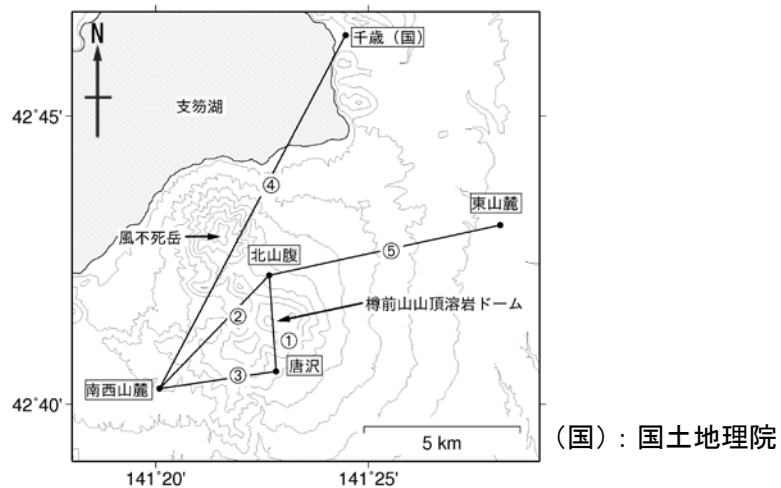
図 4 樽前山 GNSS連続観測による基線長変化（2005年 1月～2018年 7月）及び観測点配置図
