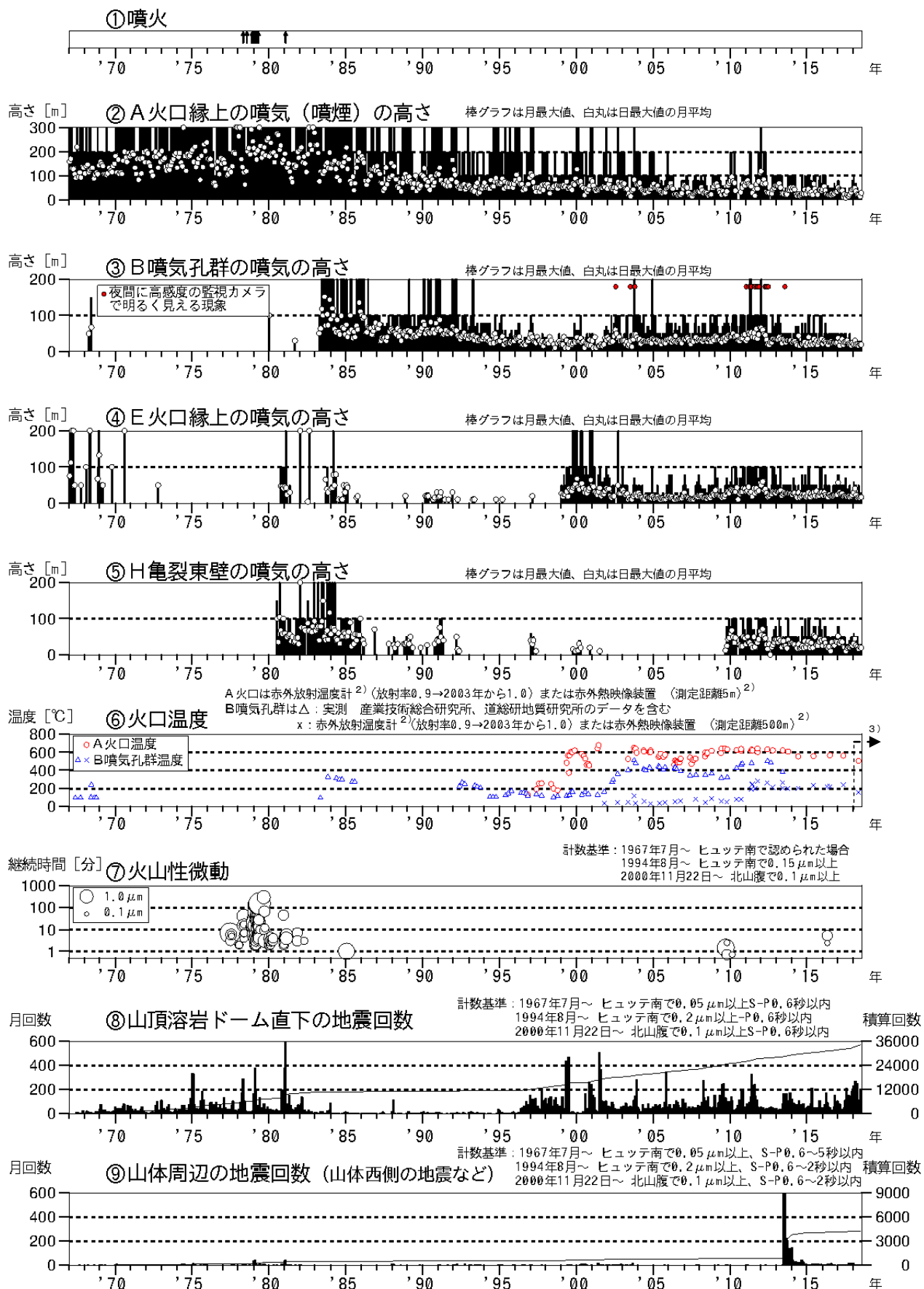
図1 樽前山 火山活動経過図（1967年1月～2018年7月）
