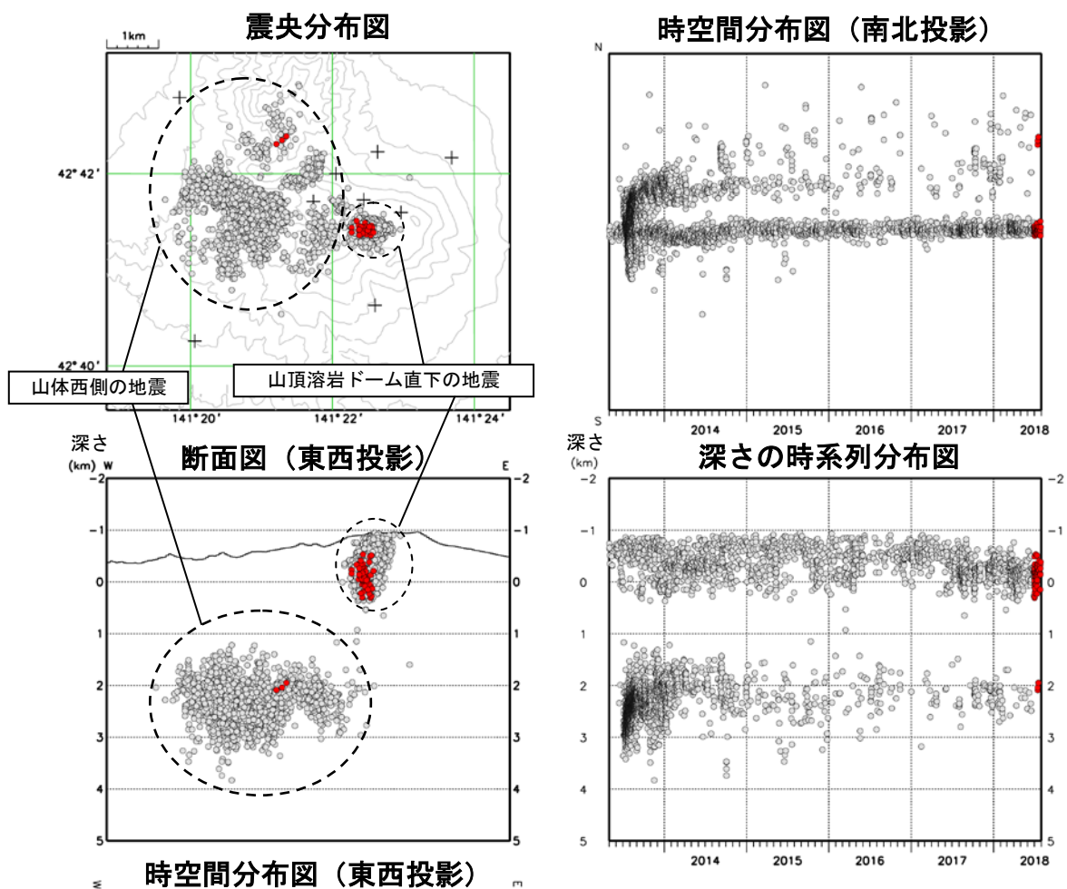
図3 樽前山 火山性地震の震源分布 （2013年5月～2018年7月） ●印：2013年5月～2018年6月の震源 ●印：2018年7月の震源 +印：地震観測点 ・2017年10月31日以降、震源計算に利用する観測点を変更しています。
