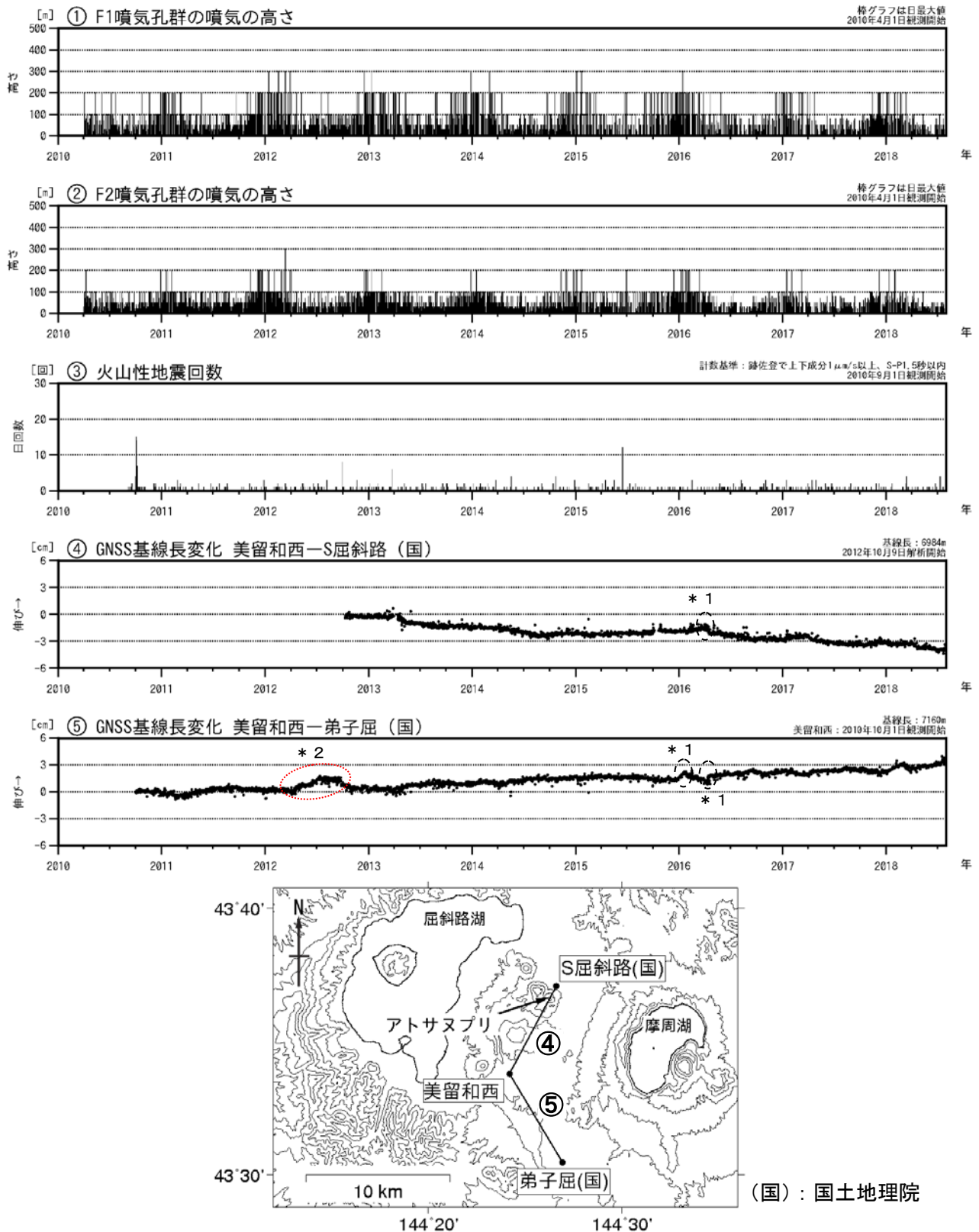
図1 アトサヌプリ 火山活動経過図（2010年4月～2018年7月）及びGNSS連続観測点配置図
