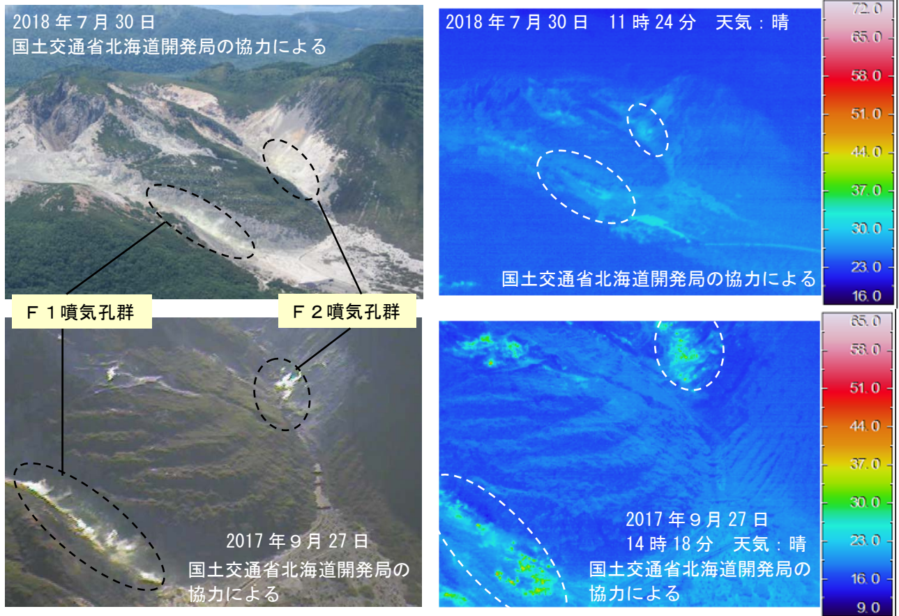
図5 アトサヌプリ F1噴気孔群及びF2噴気孔群の地表面温度分布
