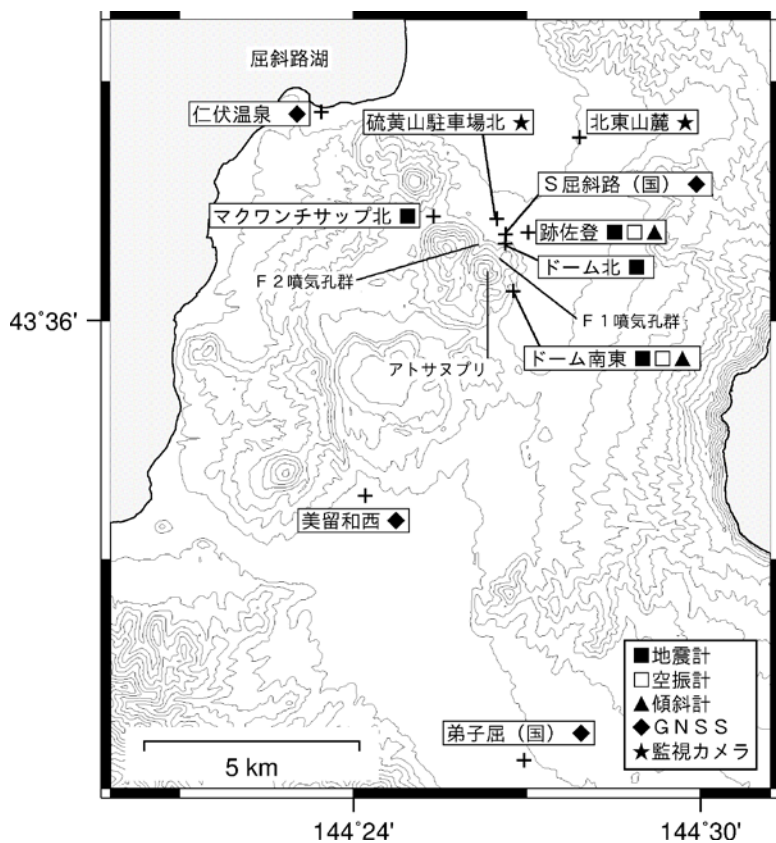
図7 アトサヌプリ 観測点配置図
