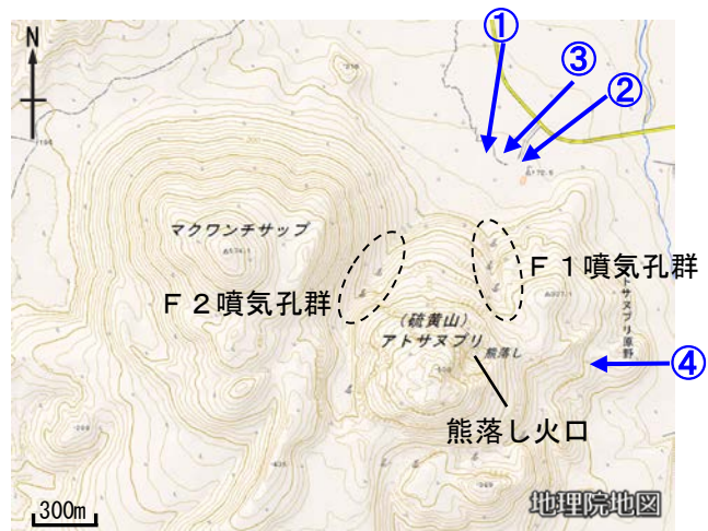
図3 アトサヌプリ 周辺図と写真及び 赤外熱映像の撮影方向（矢印）
