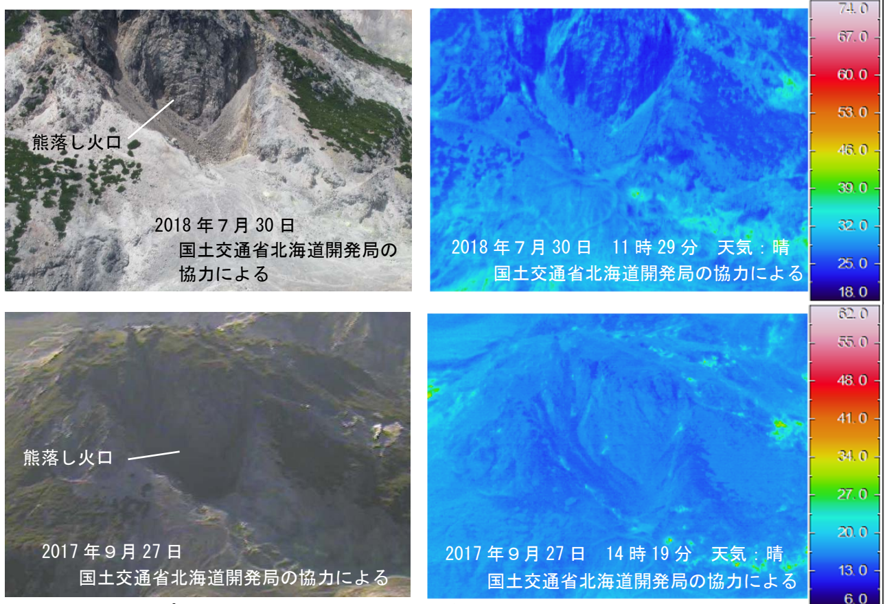
図6 アトサヌプリ 熊落し火口の地表面温度分布
