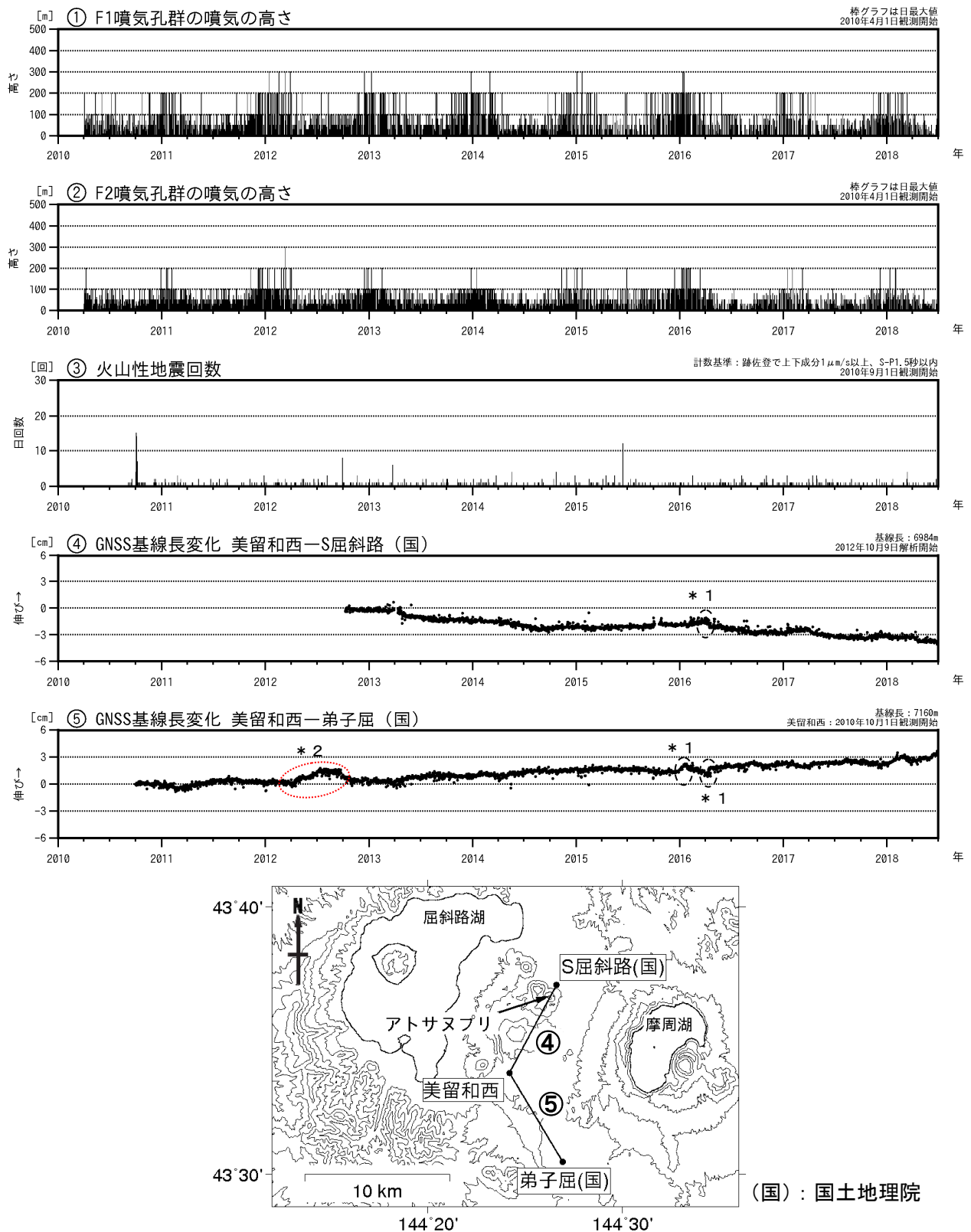
図1 アトサヌプリ 火山活動経過図（2010年4月～2018年6月）及びGNSS連続観測点配置図
