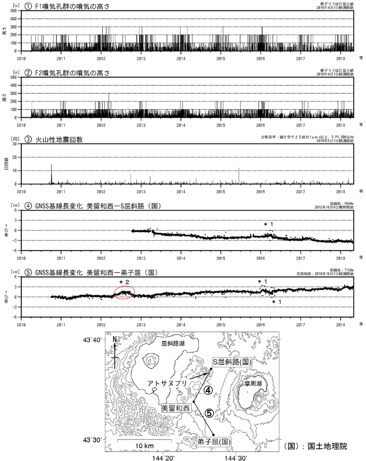
図1 アトサヌプリ 火山活動経過図（2010年4月～2018年4月）及びGNSS連続観測点配置図
