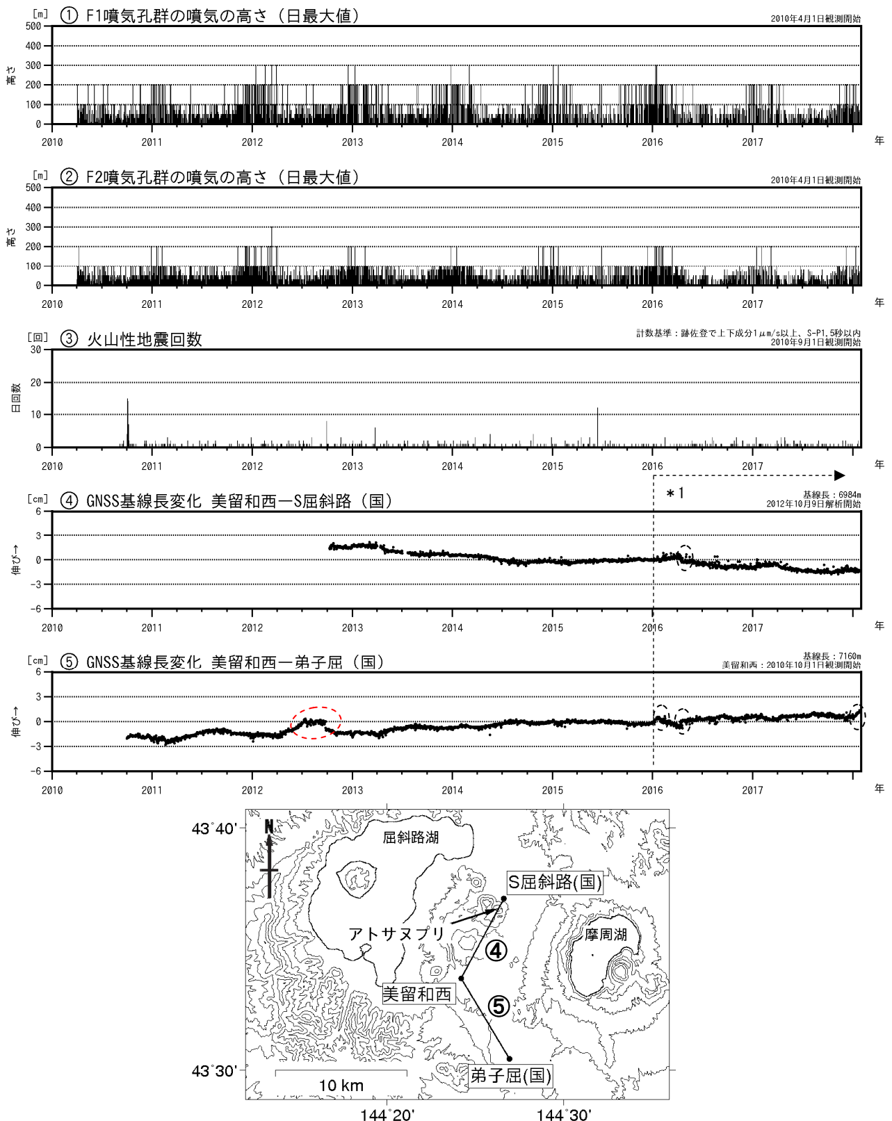
図1 アトサヌプリ 火山活動経過図（2010年4月～2018年1月）及びGNSS連続観測点配置図
