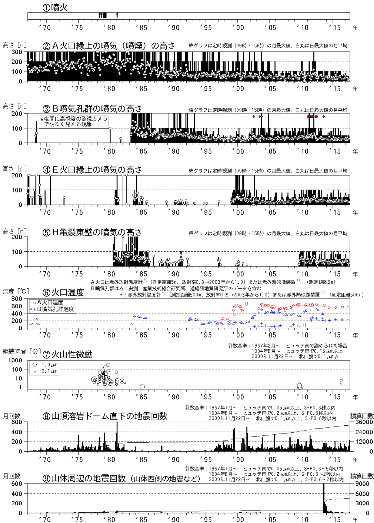
図1 樽前山 火山活動経過図（1967年1月～2017年8月）
