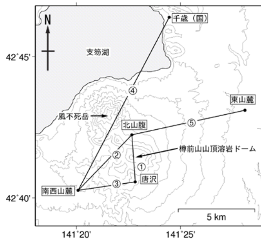
図 7 樽前山 GNSS連続観測による基線長変化（2005年 1 月～2017年 5 月）及び観測点配置図
