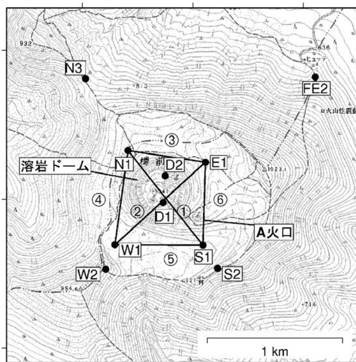
図 8 樽前山 GNSS繰り返し観測による山頂溶岩ドーム付近の基線長変化（1999年～2017年）及び観測点配置図
