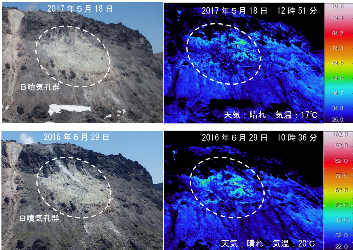
図4 樽前山 赤外熱映像装置によるB噴気孔群の地表面温度分布 (図5中の②から撮影) ・B噴気孔群では地表面温度分布に特段の変化はありませんでした
