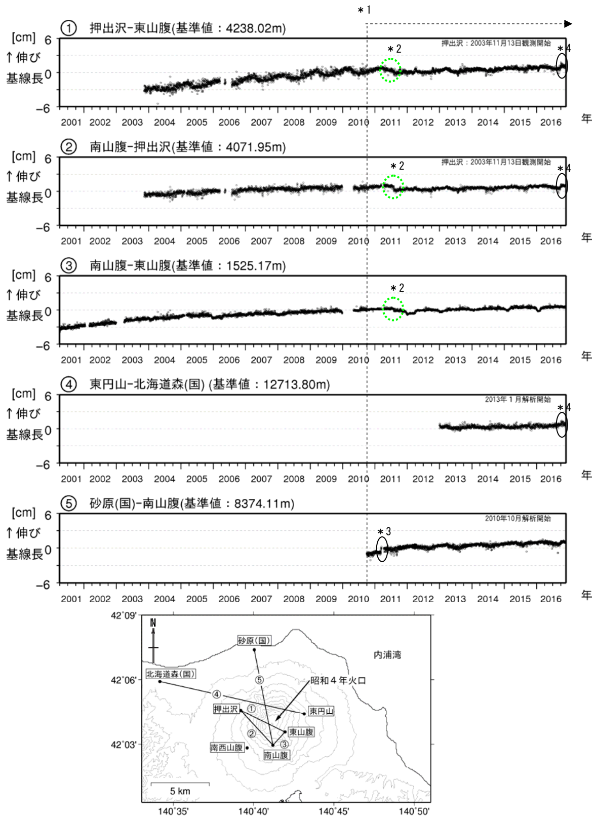
図 5 北海道駒ヶ岳 GNSS連続観測による基線長変化（2001年4月～2016年11月）及び観測点配置図
