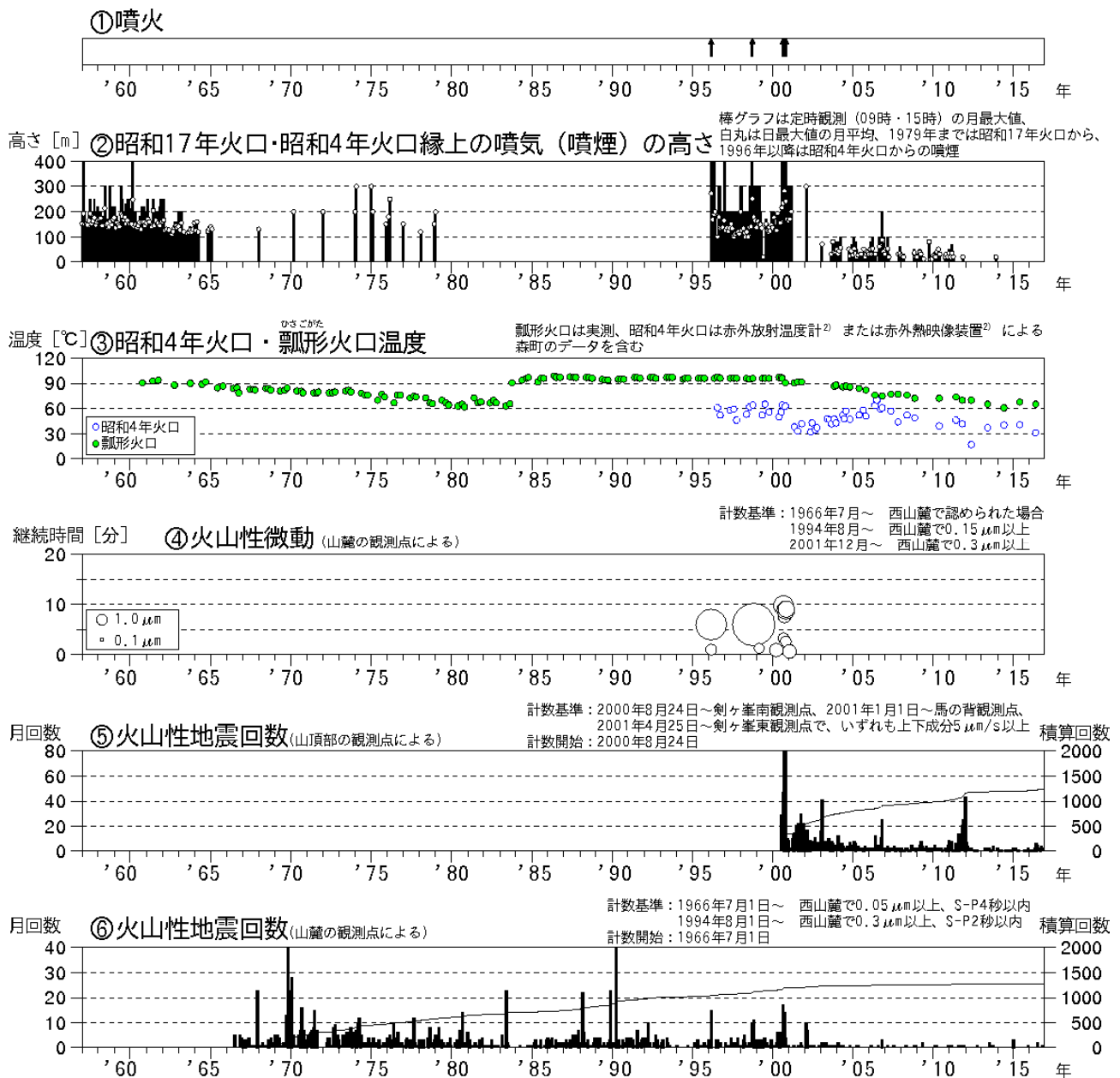
図1 北海道駒ヶ岳 火山活動経過図（1957年1月～2016年11月）
