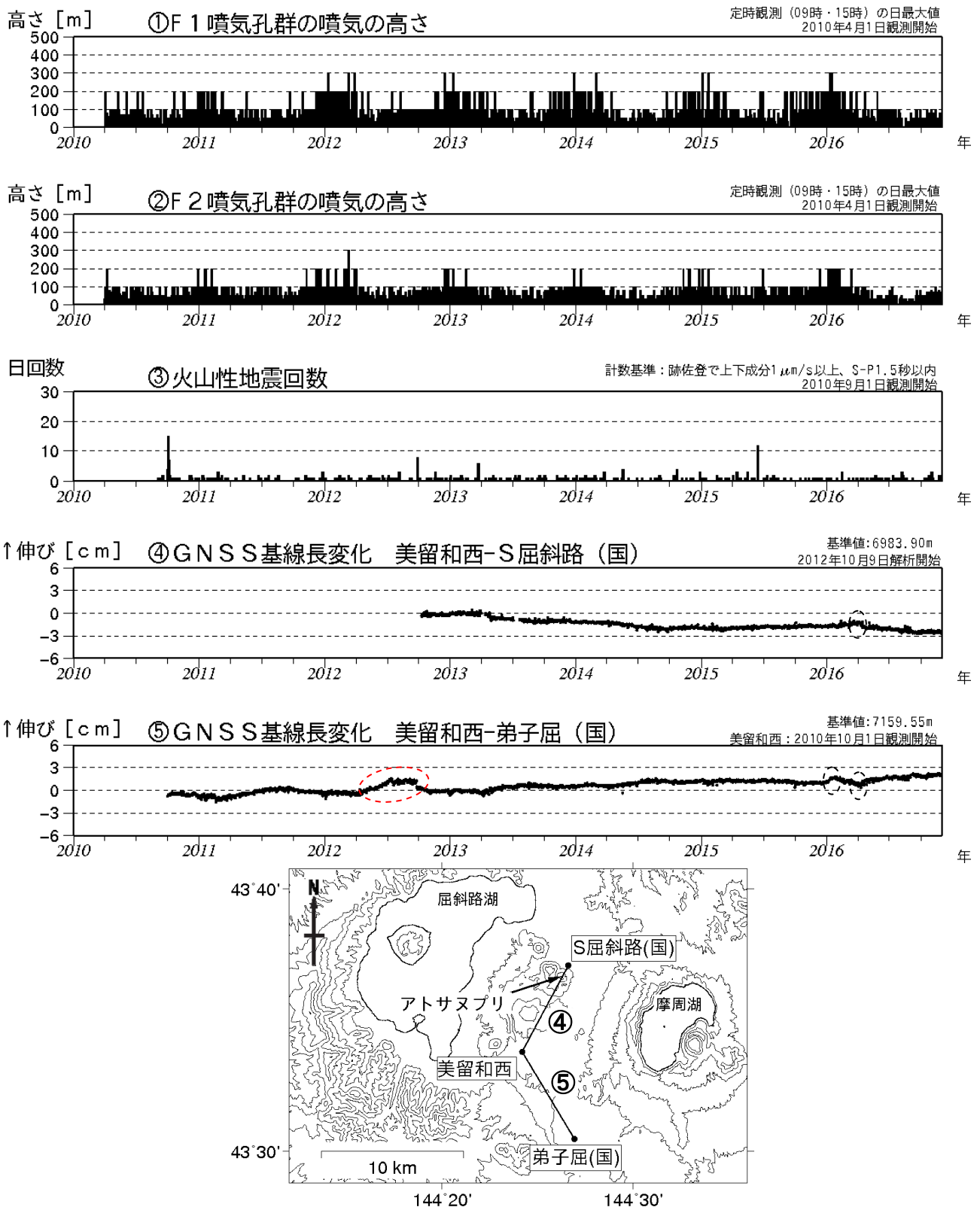
図1 アトサヌプリ 火山活動経過図 (2010年4月~2016年11月) 及びGNSS連続観測点配置図 ・GNSS基線の④⑤は観測点配置図の④⑤に対応しています ・GNSS基線の空白部分は欠測を示します ・④⑤の黒破線円内の変化は、美留和西観測点の局所的な動きによるもので、火山活動によるものではないと考えられます ・⑤の赤破線円内の変化は、弟子屈(国)付近の樹木の影響及び伐採 (2012年9月下旬) によるものです ・(国): 国土地理院
