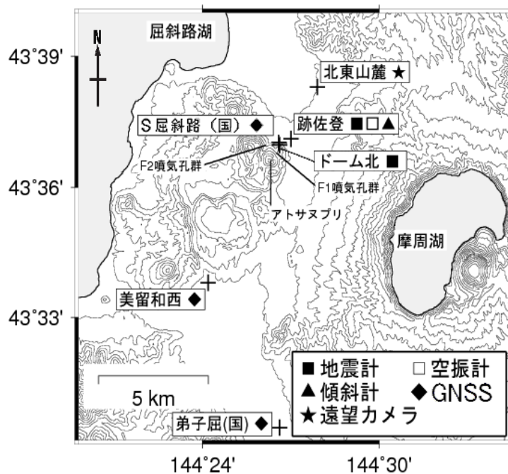
図3 アトサヌプリ 観測点配置図 +印は観測点の位置を示します 気象庁以外の機関の観測点には以下の記号を付しています (国)：国土地理院
