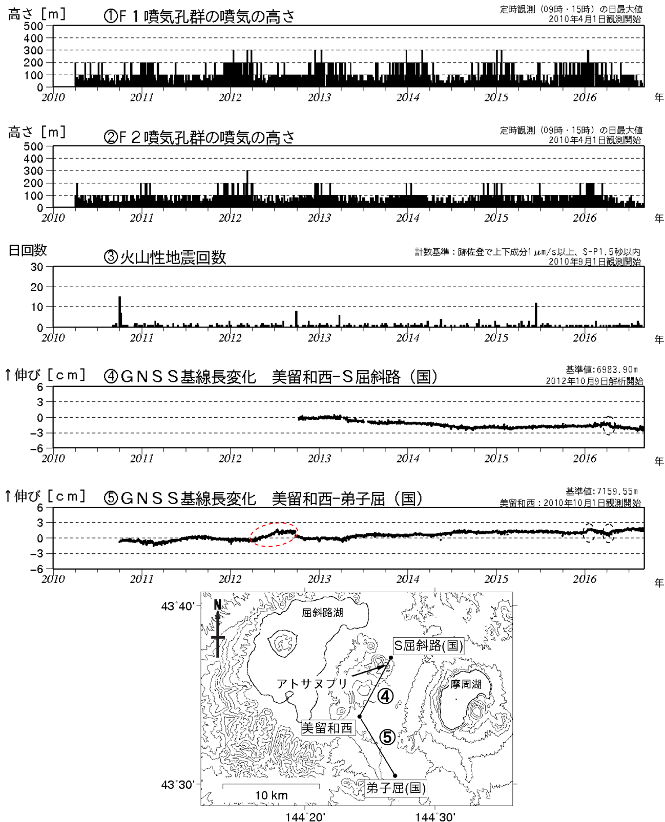
図1 アトサヌプリ 火山活動経過図（2010年4月～2016年8月）及びGNSS連続観測点配置図 ・GNSS基線の④⑤は観測点配置図の④⑤に対応しています ・GNSS基線の空白部分は欠測を示します ・④⑤の黒破線円内の変化は、美留和西観測点の局所的な動きによるもので、火山活動によるものではないと考えられます ・⑤の赤破線円内の変化は、弟子屈(国)付近の樹木の影響及び伐採（2012年9月下旬）によるものです ・(国)：国土地理院
