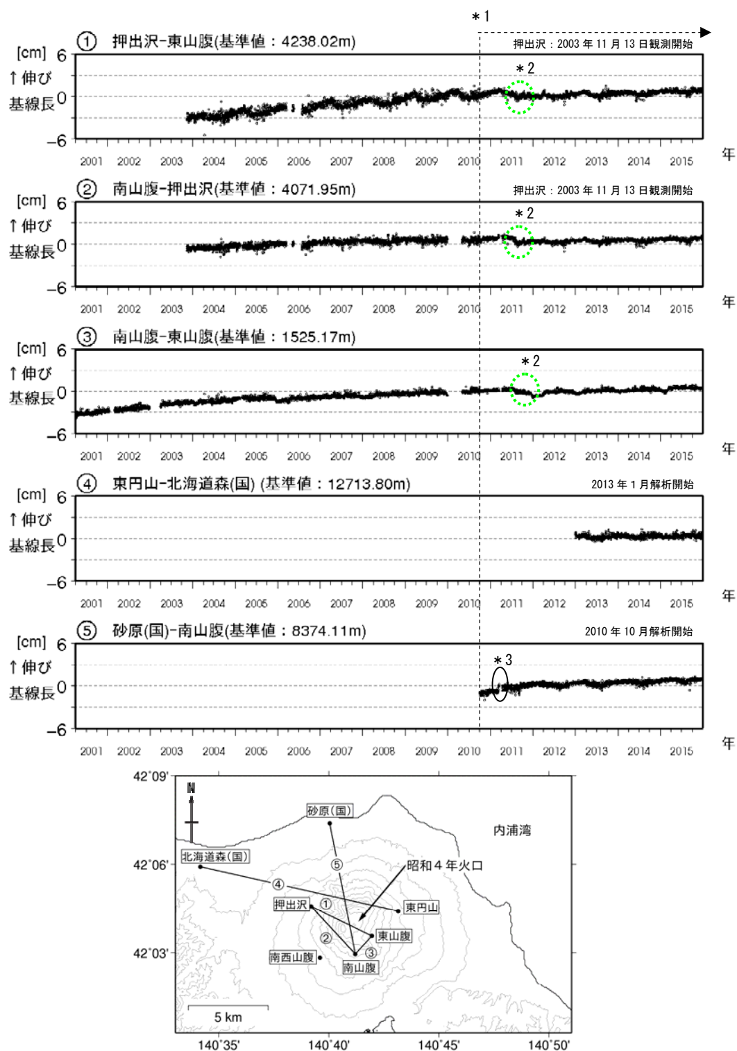
図5 北海道駒ヶ岳 GNSS連続観測による基線長変化（2001年4月～2015年12月）及び観測点配置図
