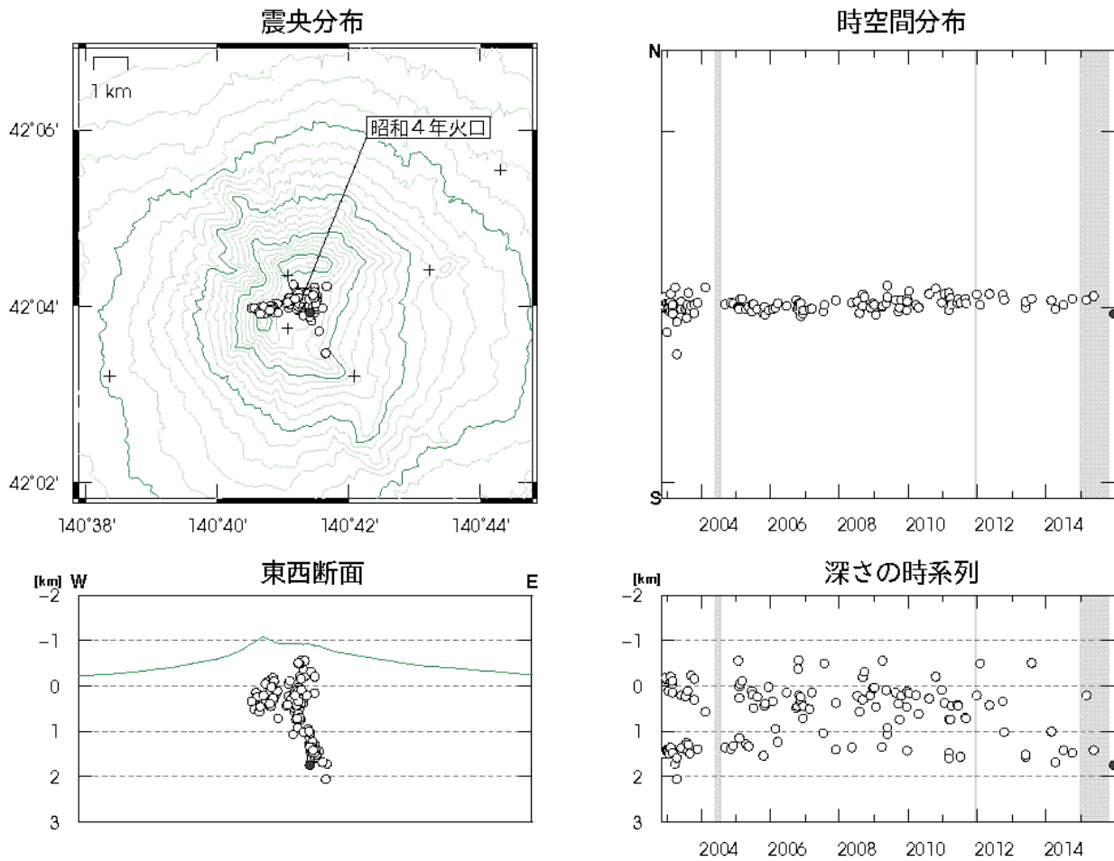
図 4 北海道駒ヶ岳 火山性地震の震源分布（2002年12月～2015年12月） 灰色の期間は一部観測点欠測のため震源の決定数減少や精度低下が見られます ○印：2002年12月～2015年11月の震源 ●印：2015年12月の震源 +印：地震観測点
