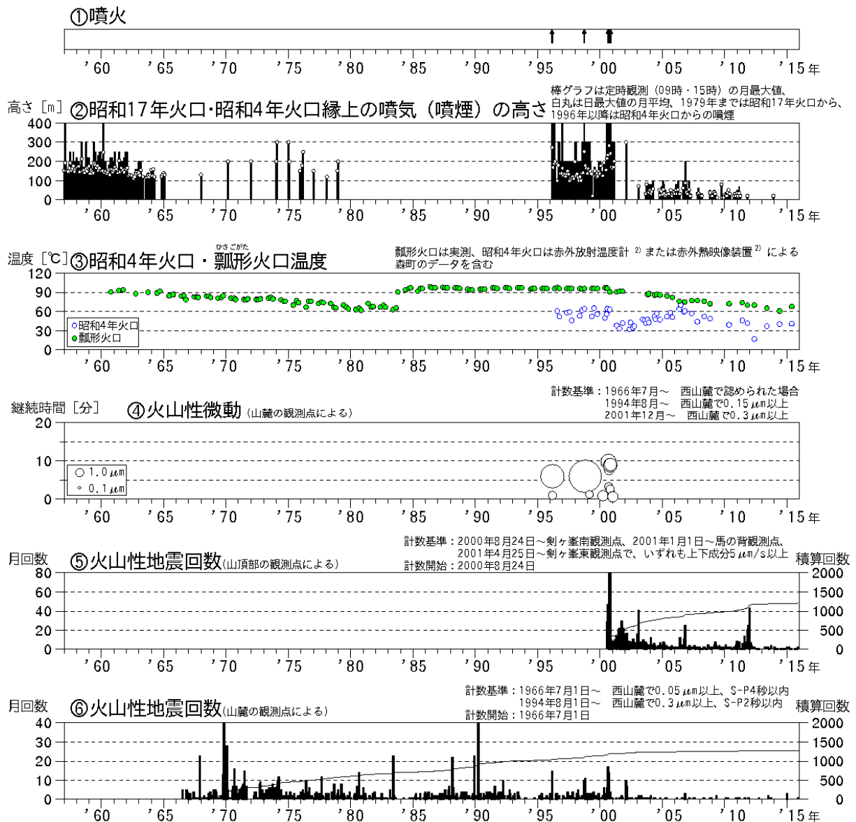
図1 北海道駒ヶ岳 火山活動経過図（1957年1月～2015年12月）
