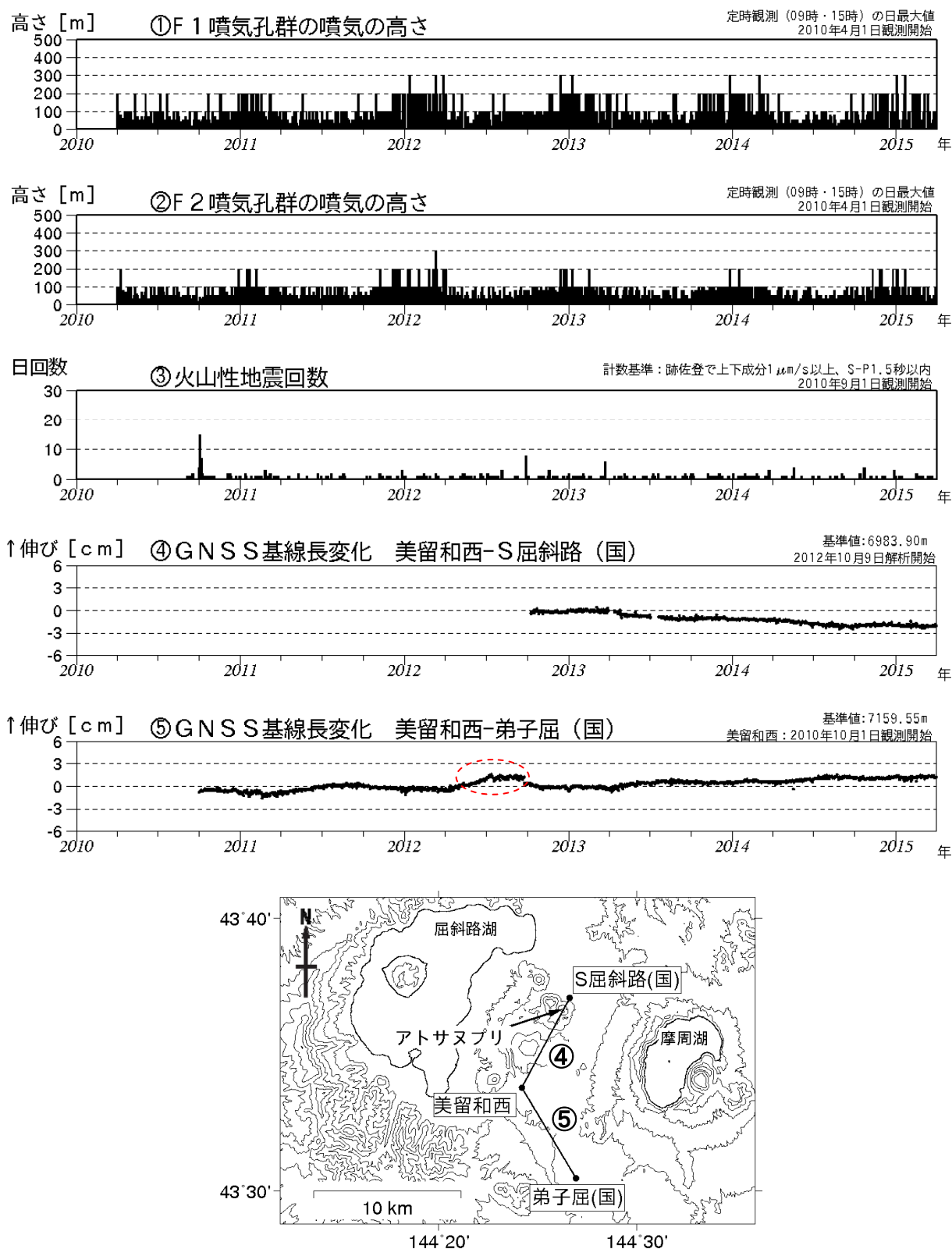
図1 アトサヌプリ 火山活動経過図（2010年4月～2015年3月）及びGNSS連続観測点配置図
