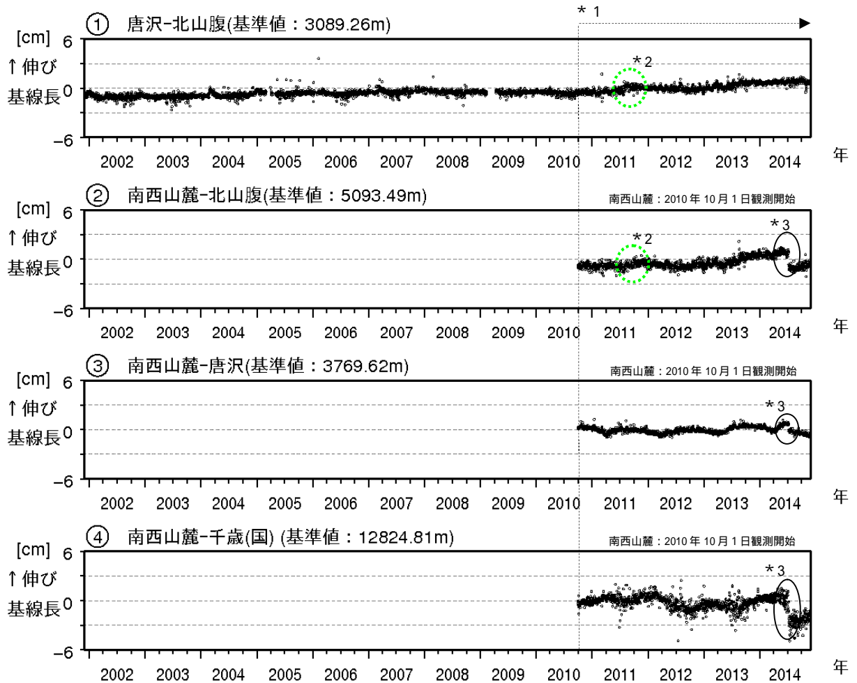
図4 樽前山 GNSS連続観測による基線長変化(2001年12月~2014年11月)
