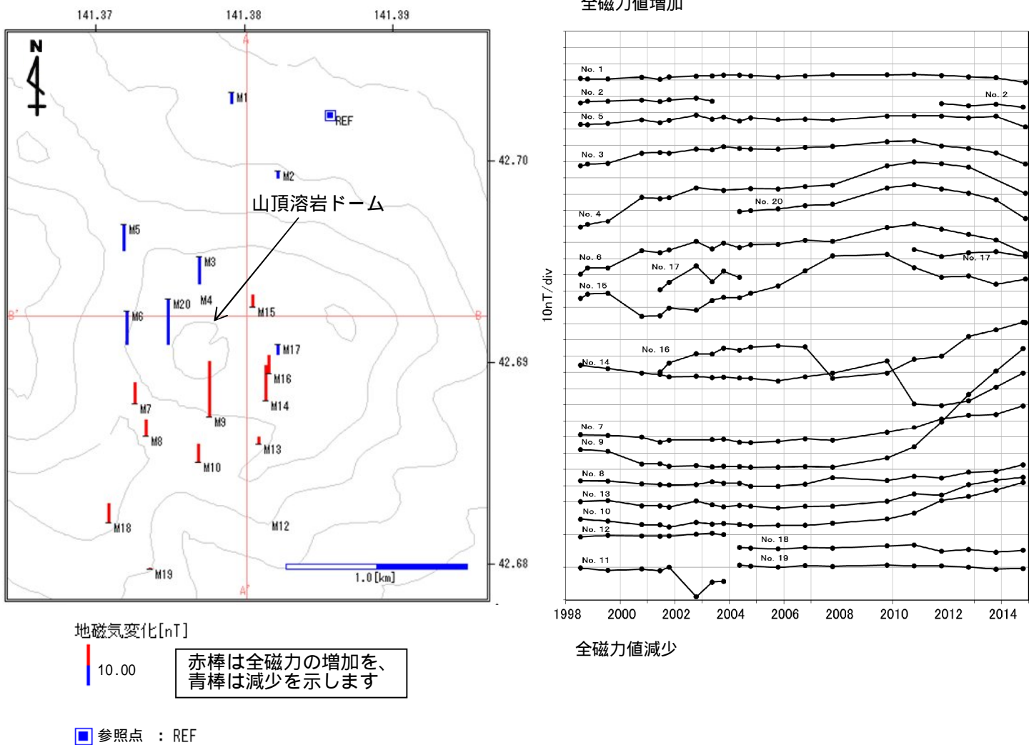
図6 樽前山 繰り返し観測による全磁力変化(参照点:北側山麓REF)
