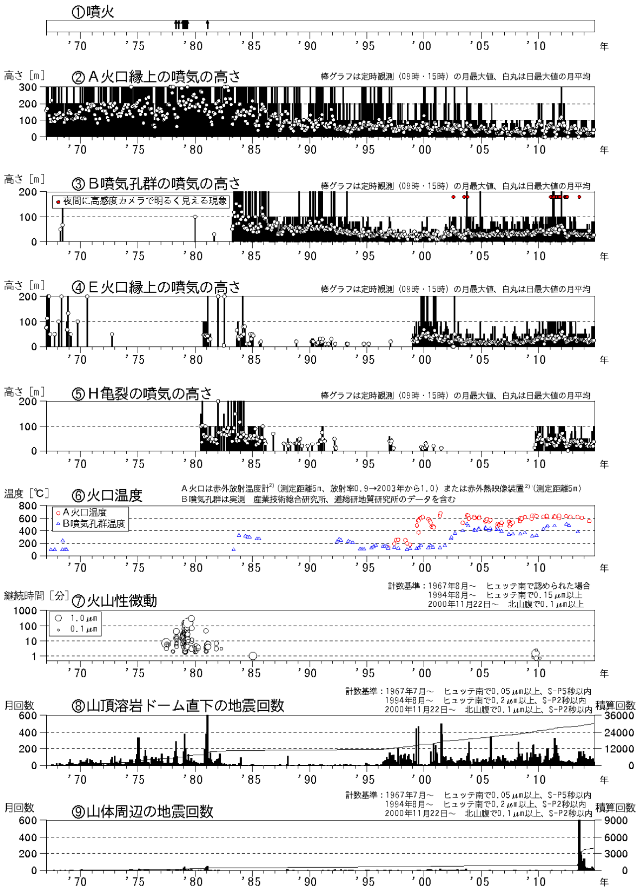
図1 樽前山 火山活動経過図(1967年1月～2014年11月)
