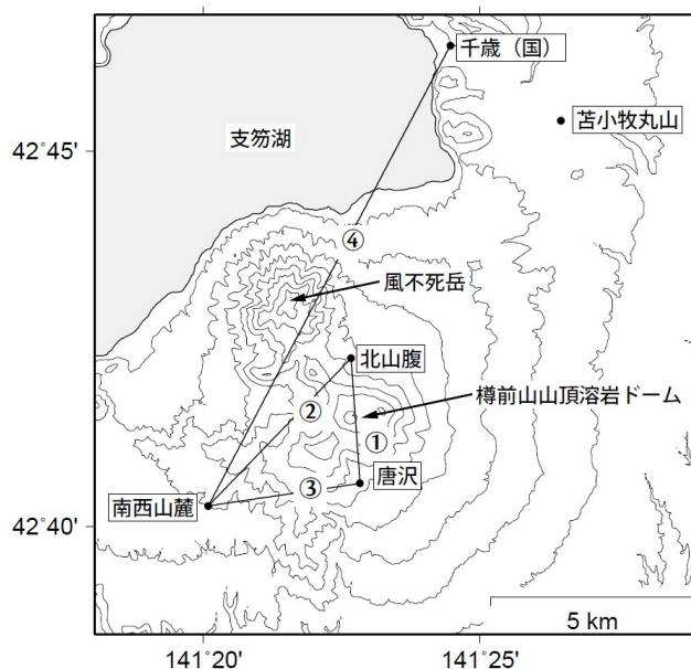
図8 樽前山 GNSS連続観測点配置図 (国): 国土地理院
