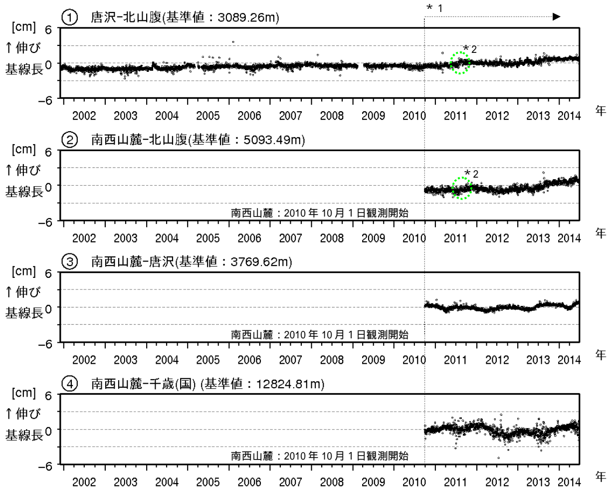
図7 樽前山 GNSS連続観測による基線長変化(2001年12月~2014年6月)
