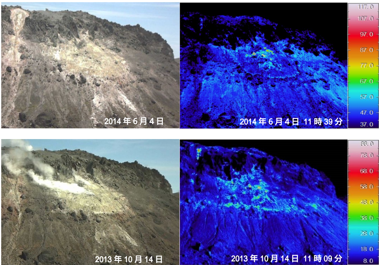
図4 樽前山 赤外熱映像装置によるB噴気孔群の地表面温度分布 （図5- から撮影）
