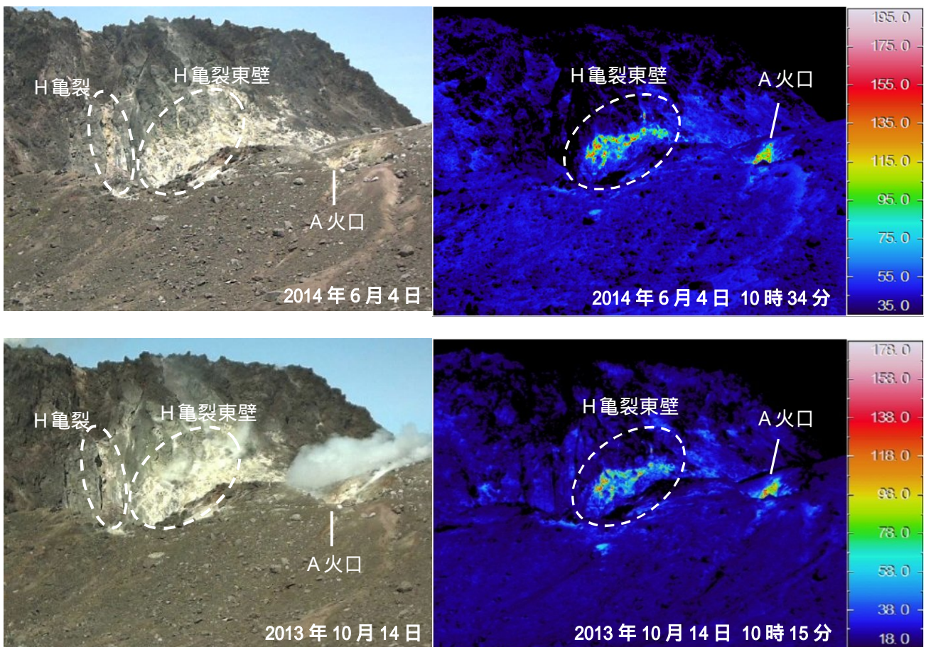
図3 樽前山 赤外熱映像装置によるA火口、H亀裂及び周辺の地表面温度分布 （図5- から撮影）
