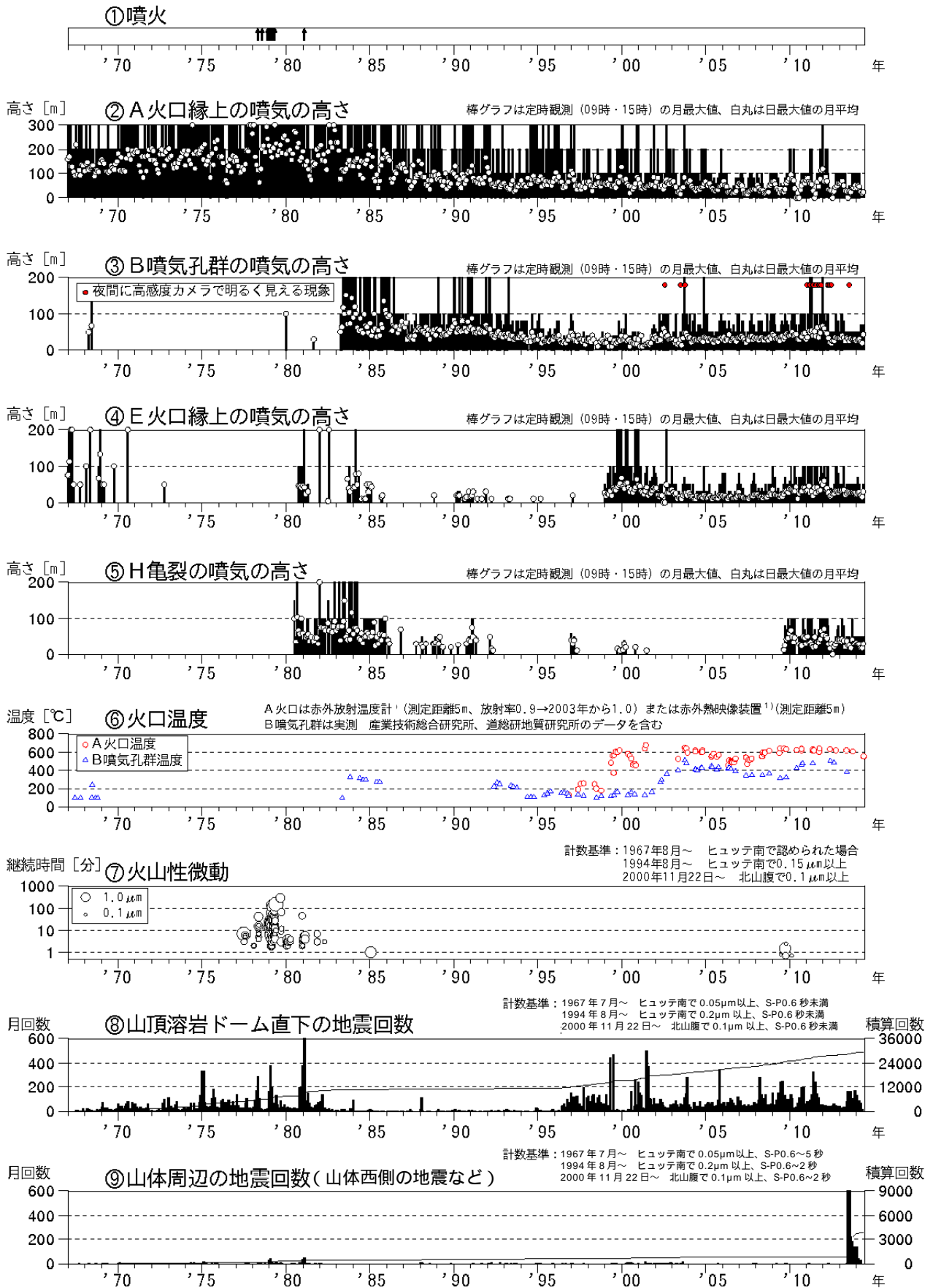
図 1 樽前山 火山活動経過図 (1967年 1 月 ~ 2014年 6 月)
