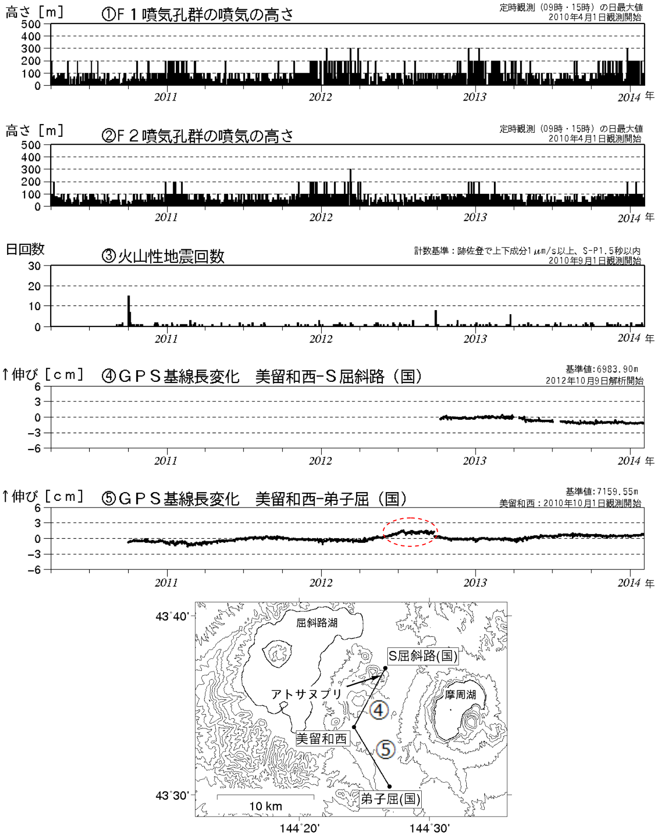
図1 アトサヌプリ 火山活動経過図（2010年4月～2014年1月）及びGPS連続観測点配置図 ・ GPS基線の④⑤は配置図の④⑤に対応しています ・ GPS基線の空白部分は欠測を示します ・ ⑤の赤破線円内の変化は、弟子屈(国)付近の樹木の影響及び伐採（2012年9月下旬）によるものです ・ (国)：国土地理院
