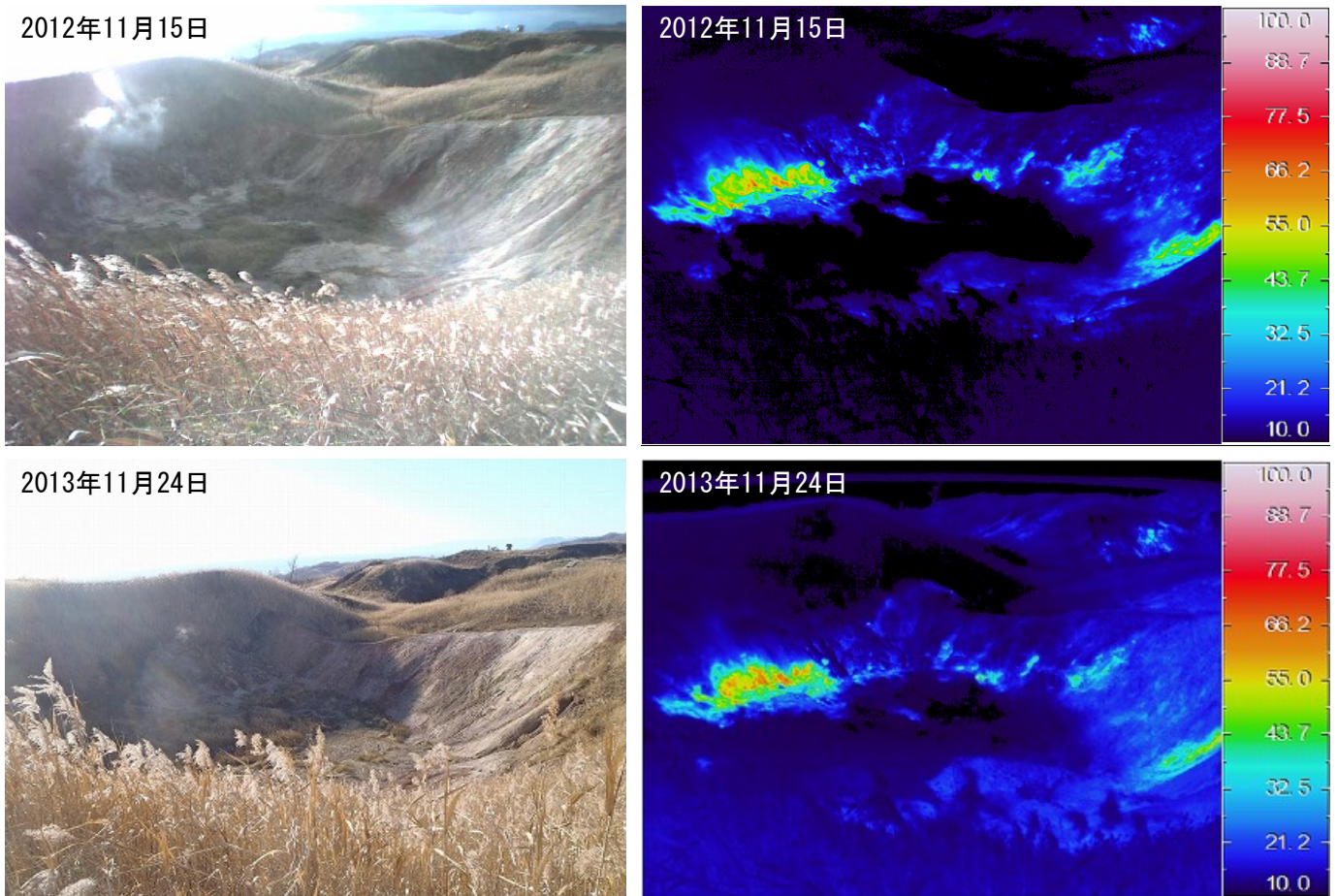
図3 有珠山 N-B火口の地表面温度分布 1) 北東側火口縁 (図2-①) から撮影
