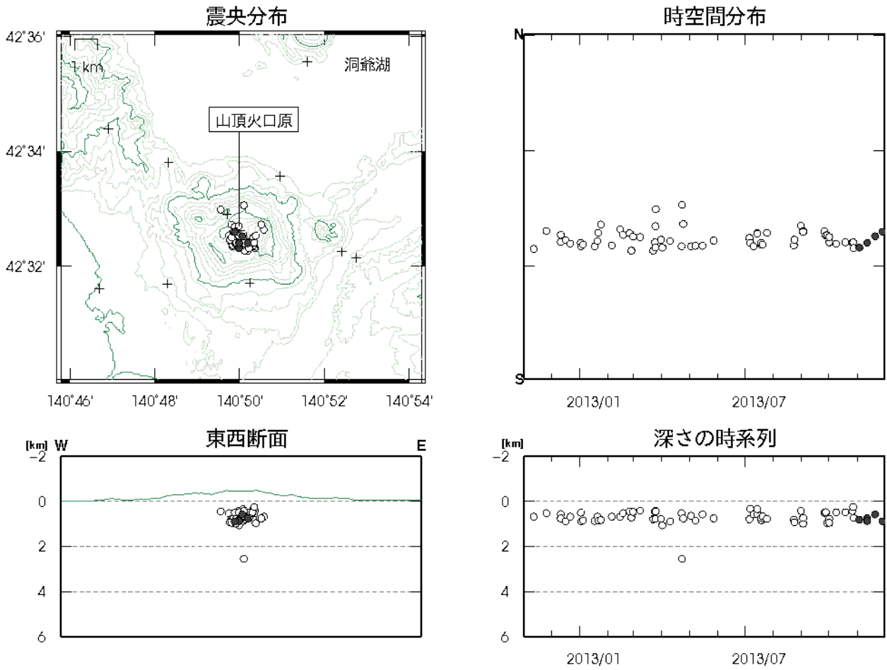
図6 有珠山 火山性地震の震源分布 (2012年11月~2013年11月)
