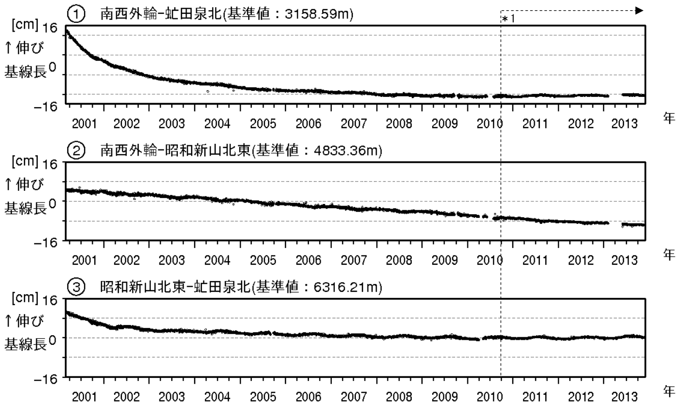
図7 有珠山 GPS連続観測による基線長変化 (2001年3月~2013年11月)
