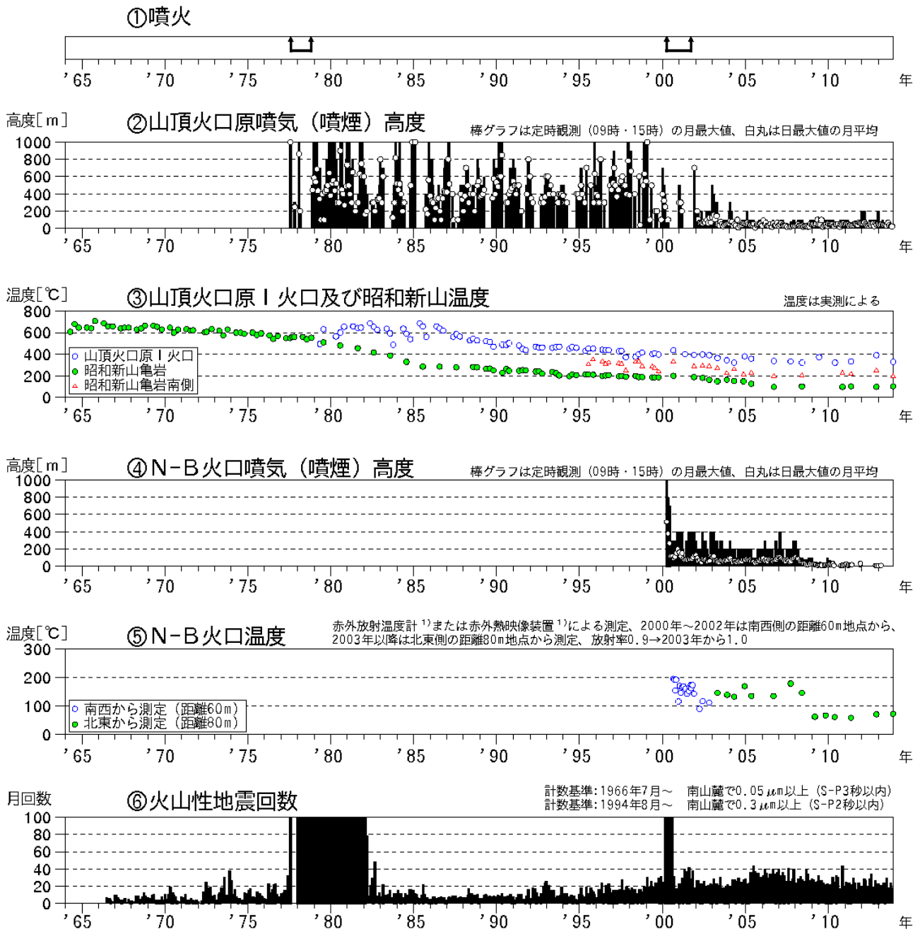
図1 有珠山 火山活動経過図 (1964年1月～2013年11月)
