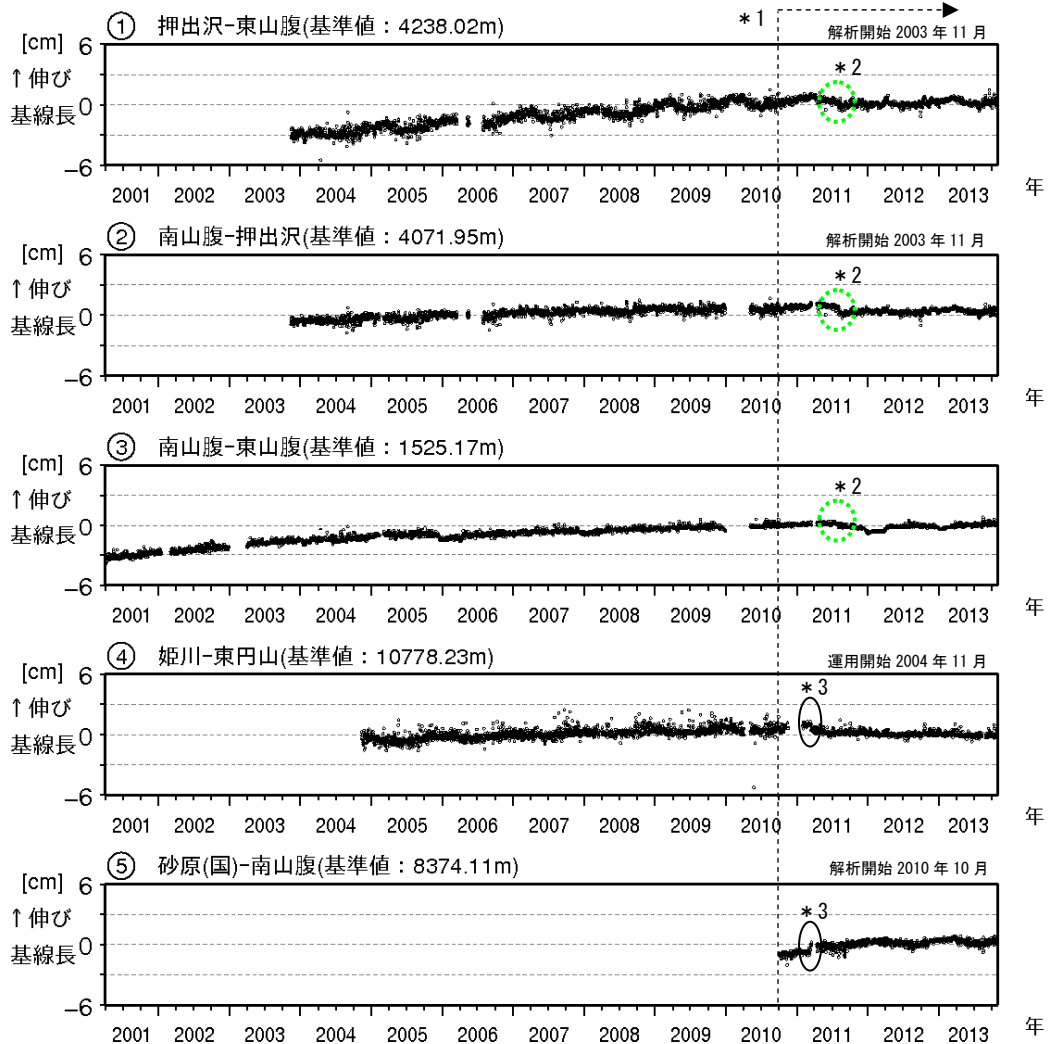
図 4 北海道駒ヶ岳 GPS連続観測による基線長変化（2001年 4 月～2013年10月）
