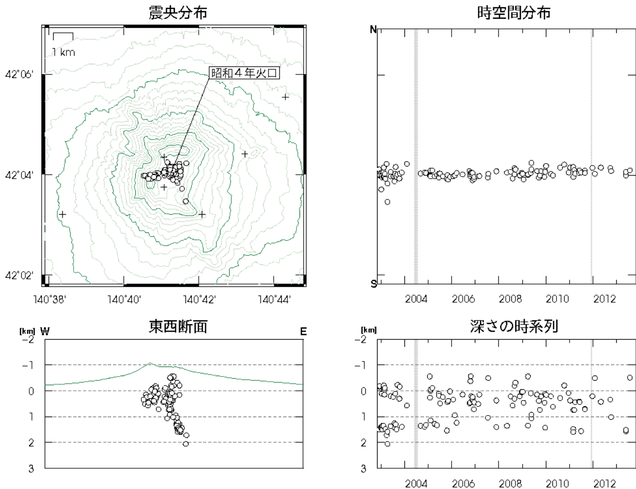
図3 北海道駒ヶ岳 火山性地震の震源分布（2002年11月～2013年10月）
