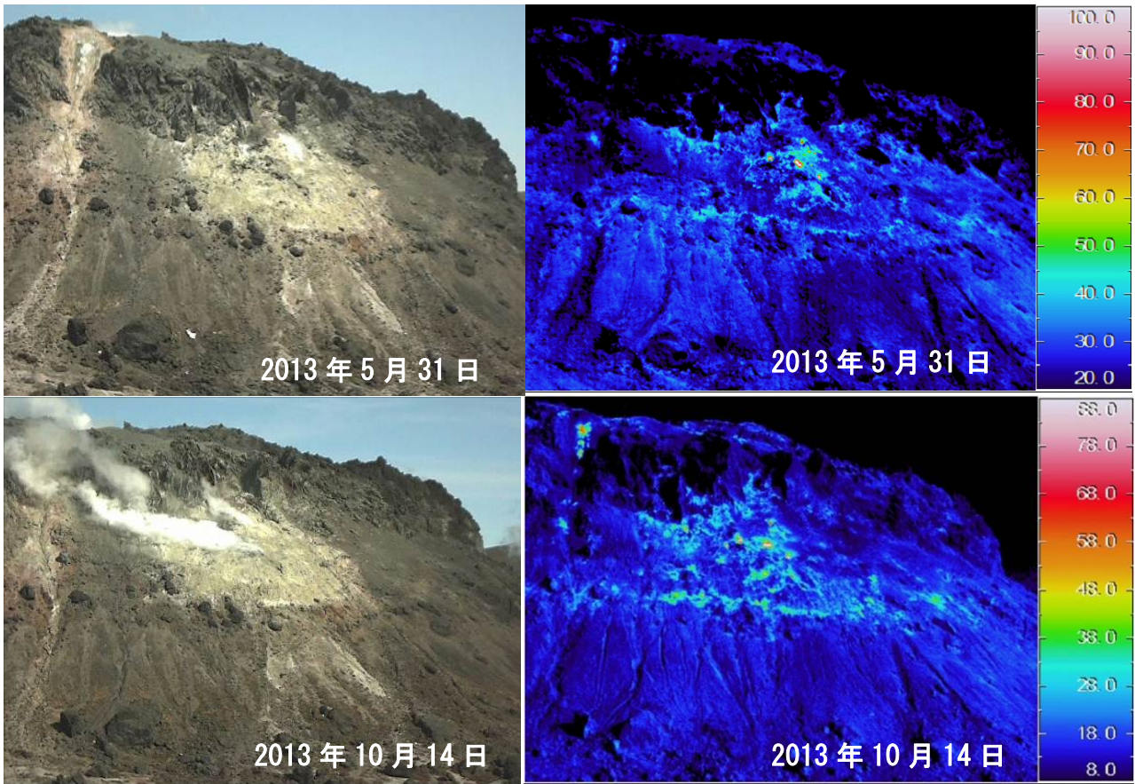
図4 樽前山 赤外熱映像装置 1) によるB噴気孔群の地表面温度分布 (図5-②から撮影)
