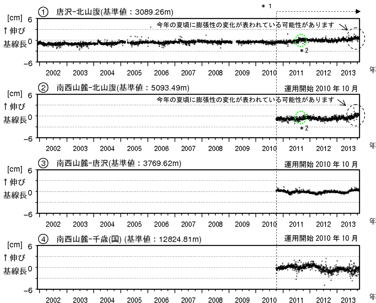
図 8 樽前山 GPS連続観測による基線長変化 (2001年12月~2013年10月)
