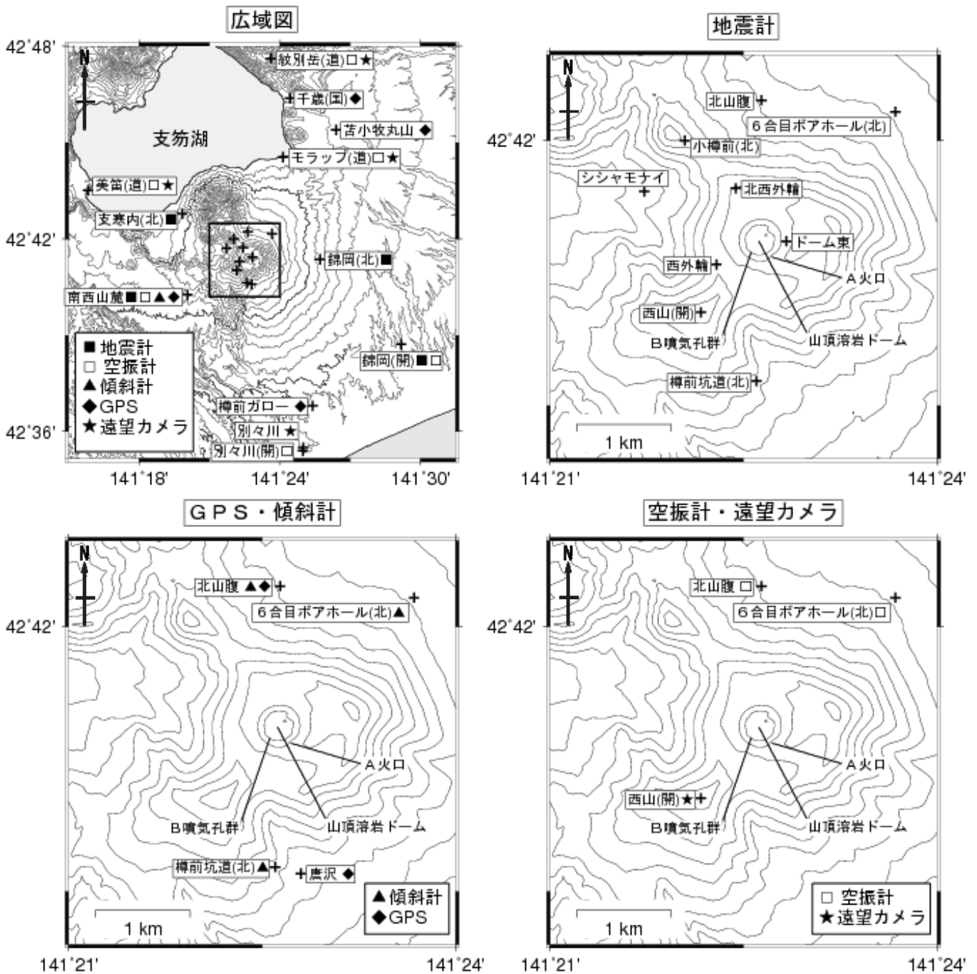
図11 樽前山 観測点配置図
