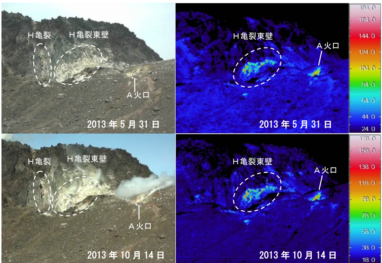
図3 樽前山 赤外熱映像装置 1) によるA火口、H亀裂および周辺の地表面温度分布 (図5-①から撮影)
