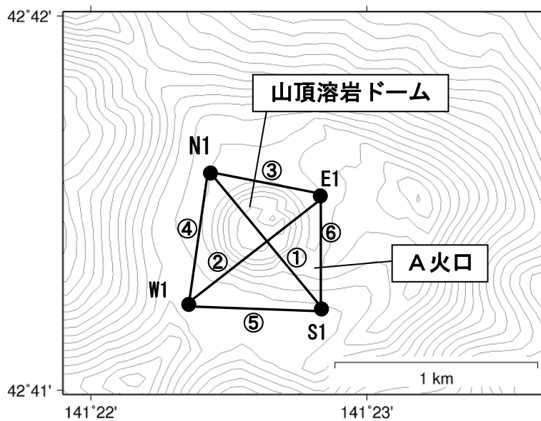
図10 樽前山 GPS繰り返し観測による山頂溶岩ドーム付近の基線長変化 (1999年～2013年) および観測点配置図
