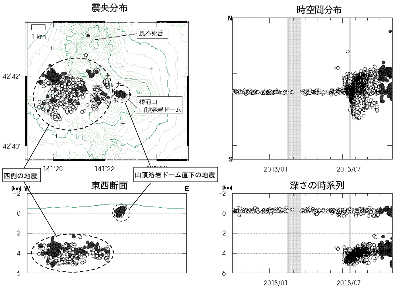
図7 樽前山 火山性地震の震源分布 (2012年9月～2013年10月)
