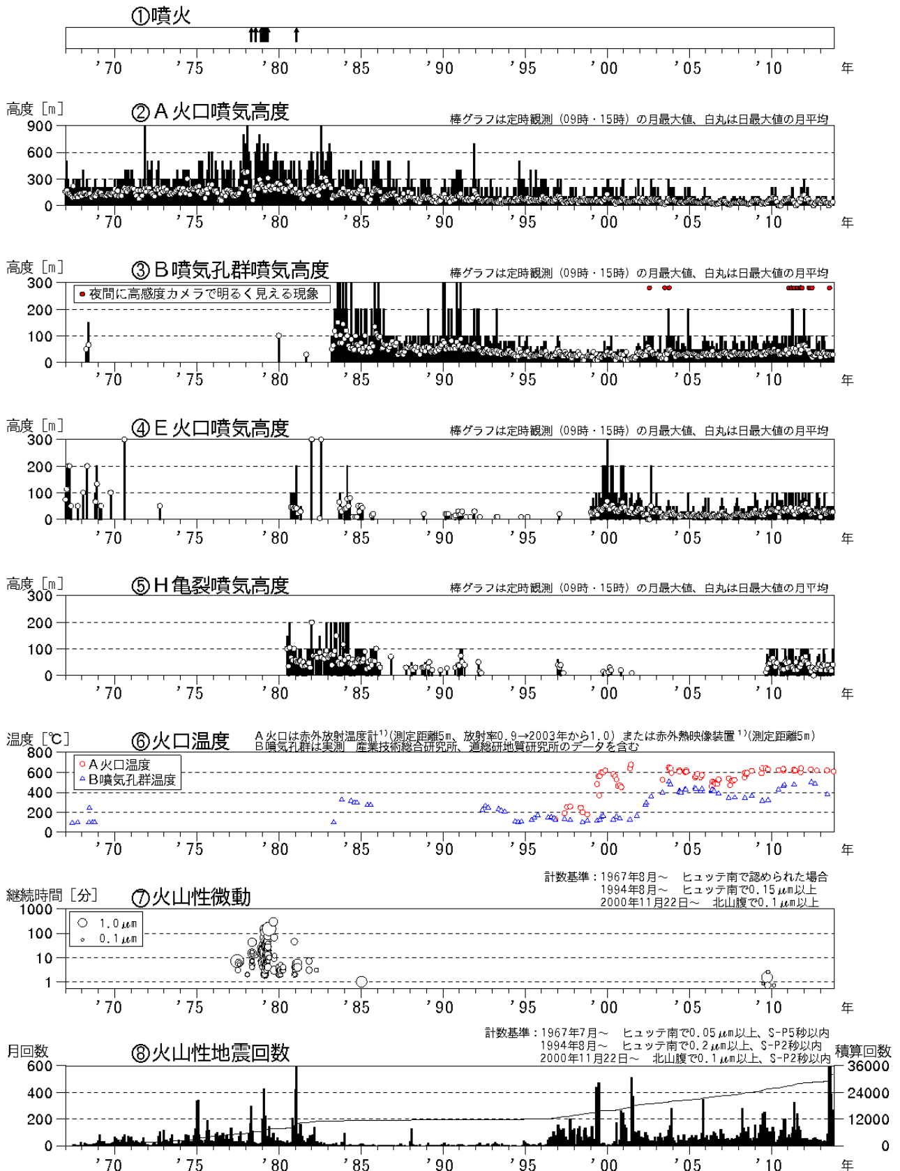
図1 樽前山 火山活動経過図 (1967年1月～2013年10月)
