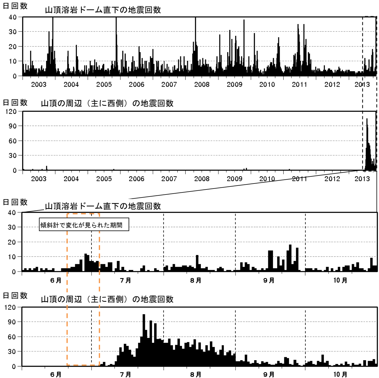
図 6 樽前山 発生領域毎の日別地震回数 (上段 : 2003 年 1 月 1 日 ~ 2013 年 10 月 31 日) (下段 : 2013 年 6 月 1 日 ~ 10 月 31 日)
