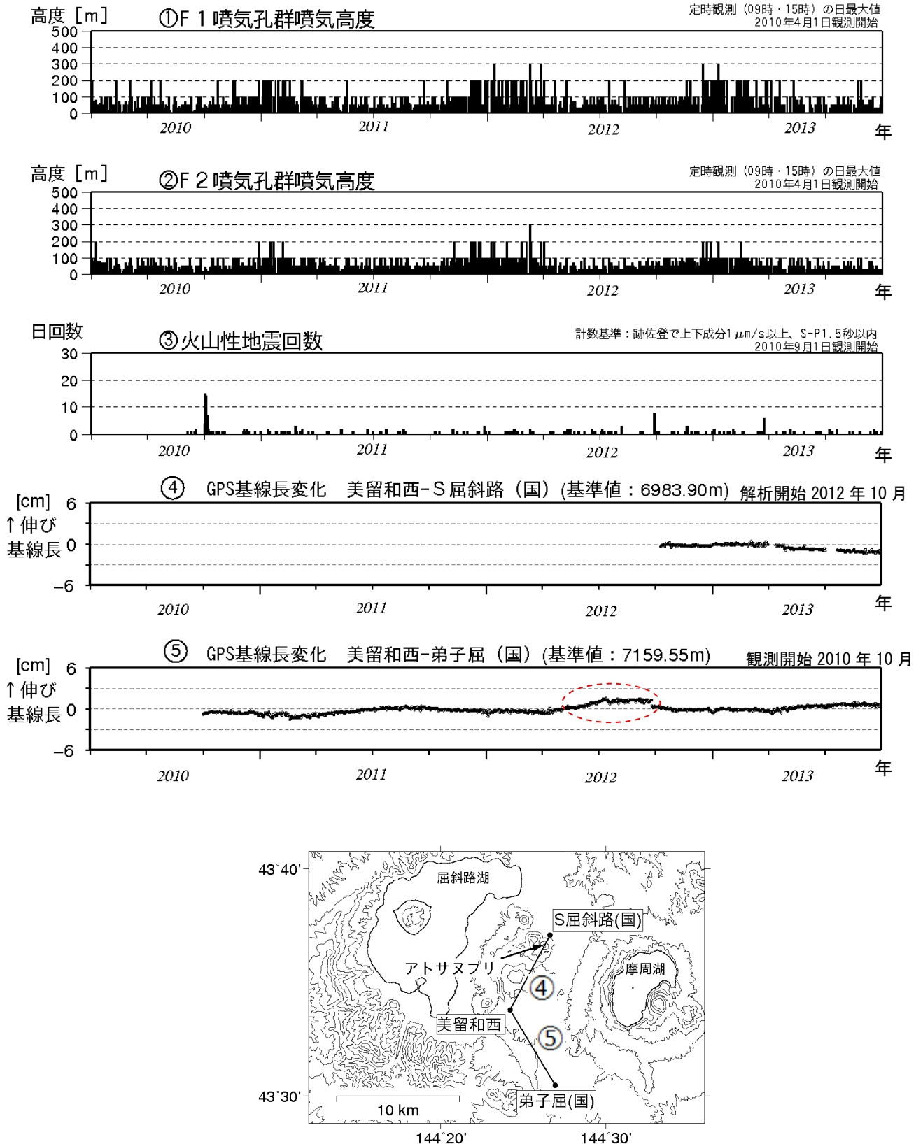
図1 アトサヌプリ 火山活動経過図 (2010年4月～2013年9月) 及びGPS連続観測点配置図 ・GPS基線の④⑤は配置図の④⑤に対応しています ・⑤の赤破線円内の変化は、弟子屈(国)付近の樹木の影響及び伐採 (2012年9月下旬) によるものです ・(国): 国土地理院
