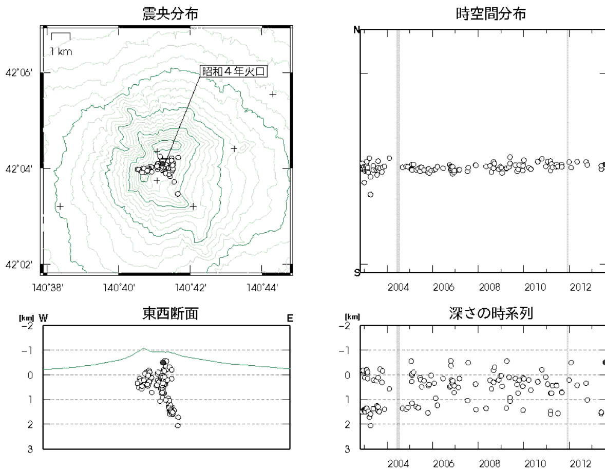
図3 北海道駒ヶ岳 火山性地震の震源分布（2002年11月～2013年8月）
