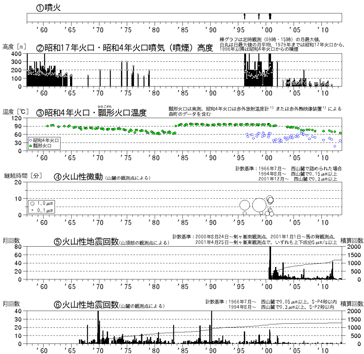
図1 北海道駒ヶ岳 火山活動経過図（1957年1月～2013年8月）
