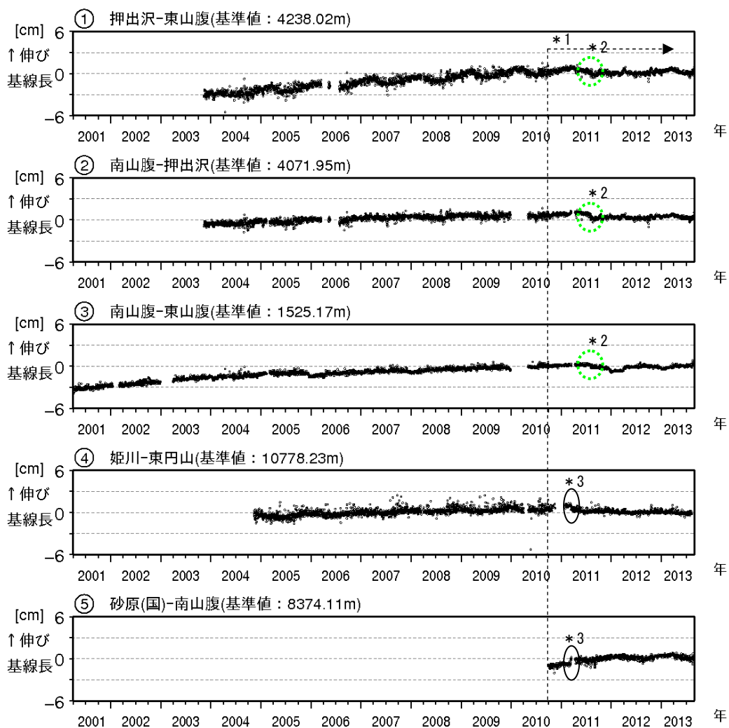
図 4 北海道駒ヶ岳 GPS連続観測による基線長変化（2001年 4 月～2013年 8 月） ・GPS基線①～⑤は図 5 の①～⑤に対応しています * 1 : 2010年10月以降のデータについては、解析方法を改良して精度を向上させています * 2 : 緑点線円内の変動は、機器更新によるものです * 3 : 楕円内の変動は、2011年 3 月11日に発生した東北地方太平洋沖地震の影響によるものであり、火山活動によるものではありません
