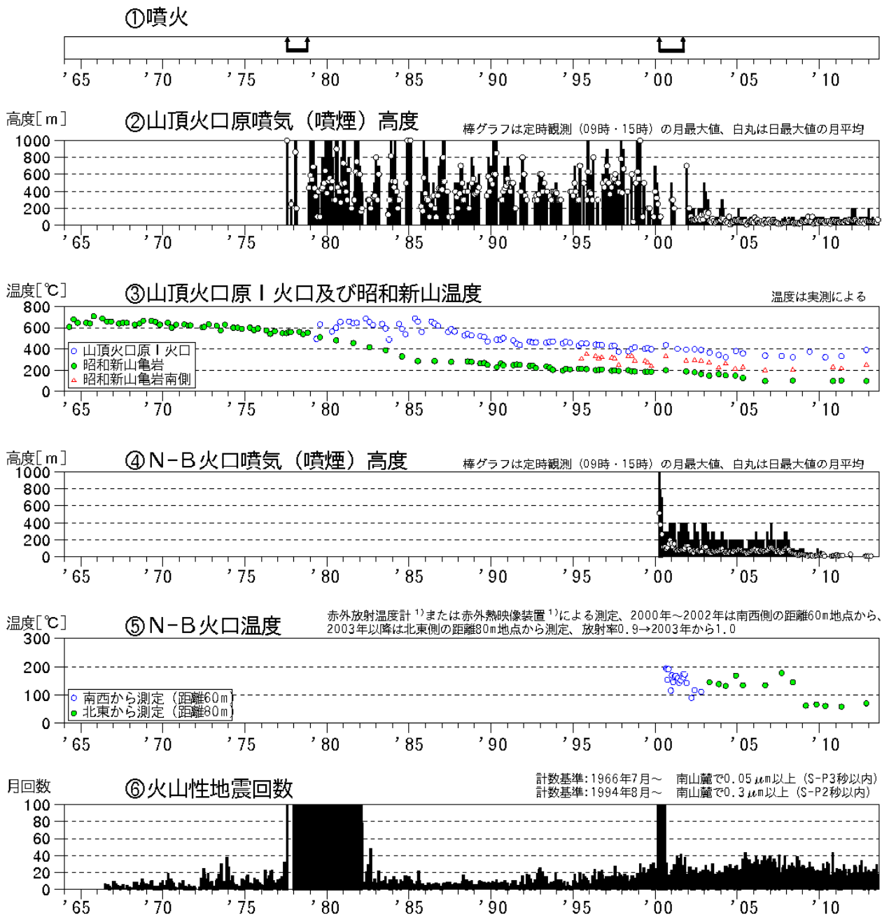
図 1 有珠山 火山活動経過図（1964年 1 月～2013年 8 月） ↑印で挟まれた期間は噴火活動期を示します
