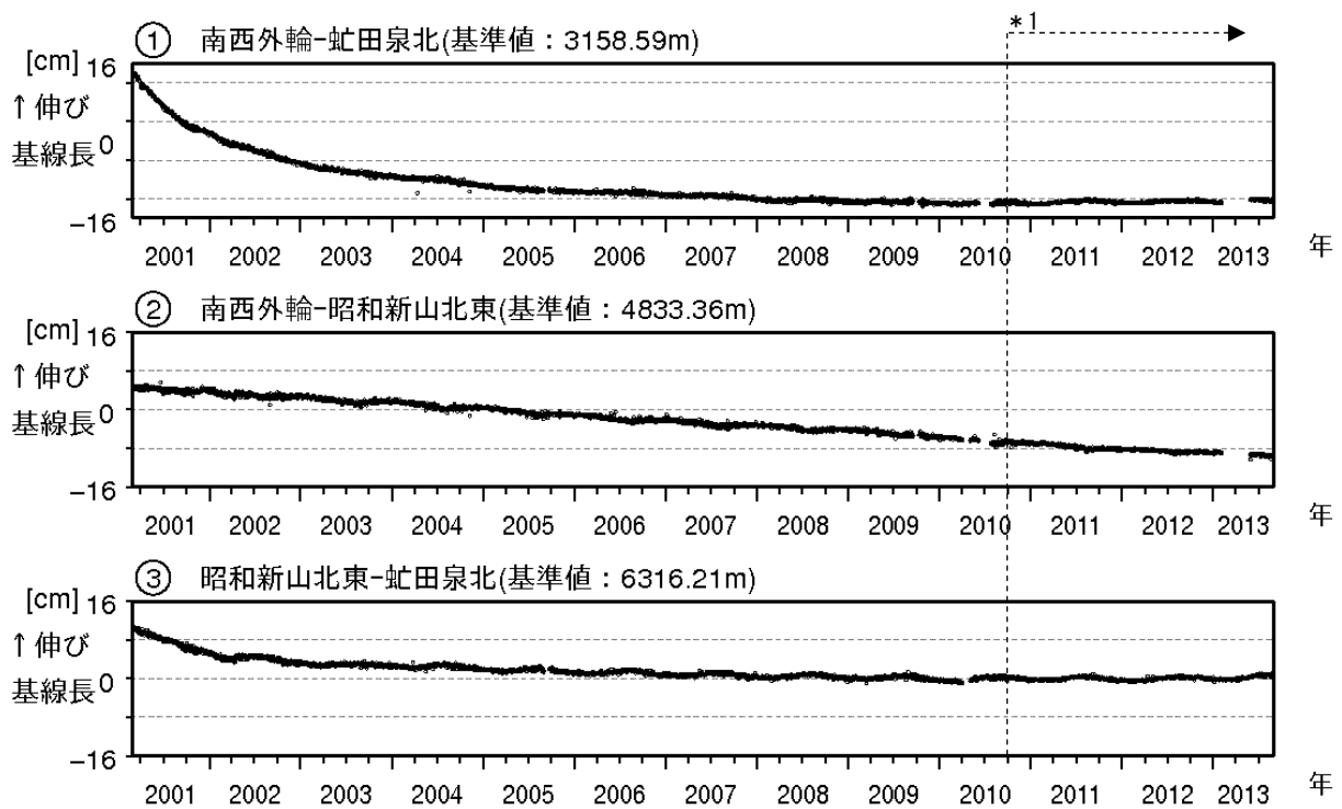
図 4 有珠山 GPS連続観測による基線長変化 (2001年3月～2013年8月)
