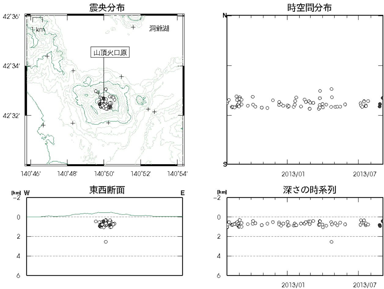
図3 有珠山 火山性地震の震源分布 (2012年8月～2013年8月)
